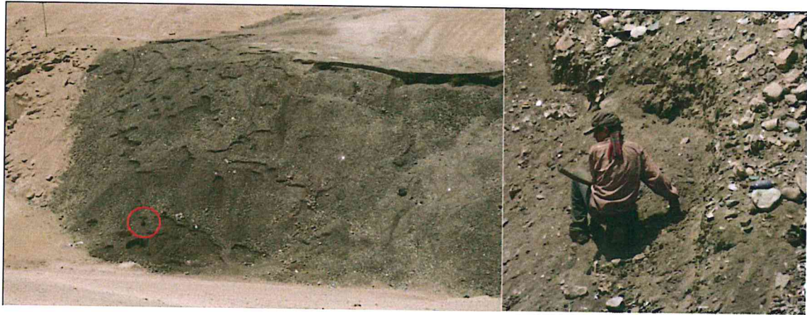
Foto 2. Antiguo botadero municipal de la ciudad de Tacna, recicladores de basura socavan base del talud del botadero provocando derrumbes en margen derecha de la quebrada del Diablo. En la foto de la izquierda se aprecia un reciclador (circulo rojo), en la foto de la derecha el detalle.
