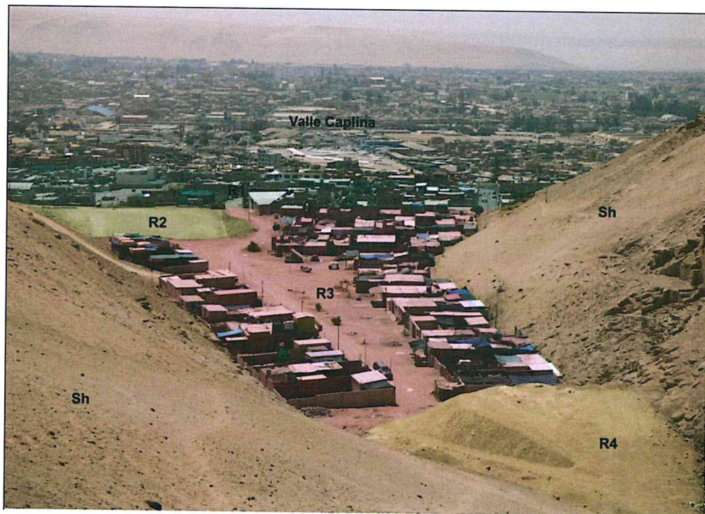
Foto 3. Asociación de Vivienda La Florida, donde se diferenciaron hasta cuatro niveles de rellenos (R1, R2, R3 y R4). Las viviendas fueron edificadas sobre estos depósitos y en pleno cauce de la quebrada Del Diablo; sobre el R4 se encuentra el antiguo botadero municipal de la ciudad de Tacna, en ambas márgenes de la quebrada se aprecia las tobas de la Formación Huaylillas (Sh).
