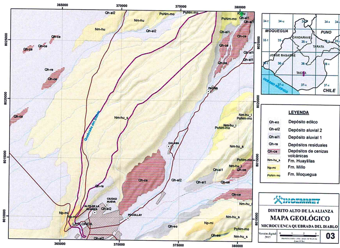
Figura 3. Unidades geológicas en la microcuenca de la quebrada del Diablo (Fuente: INGEMMET, 2011).
