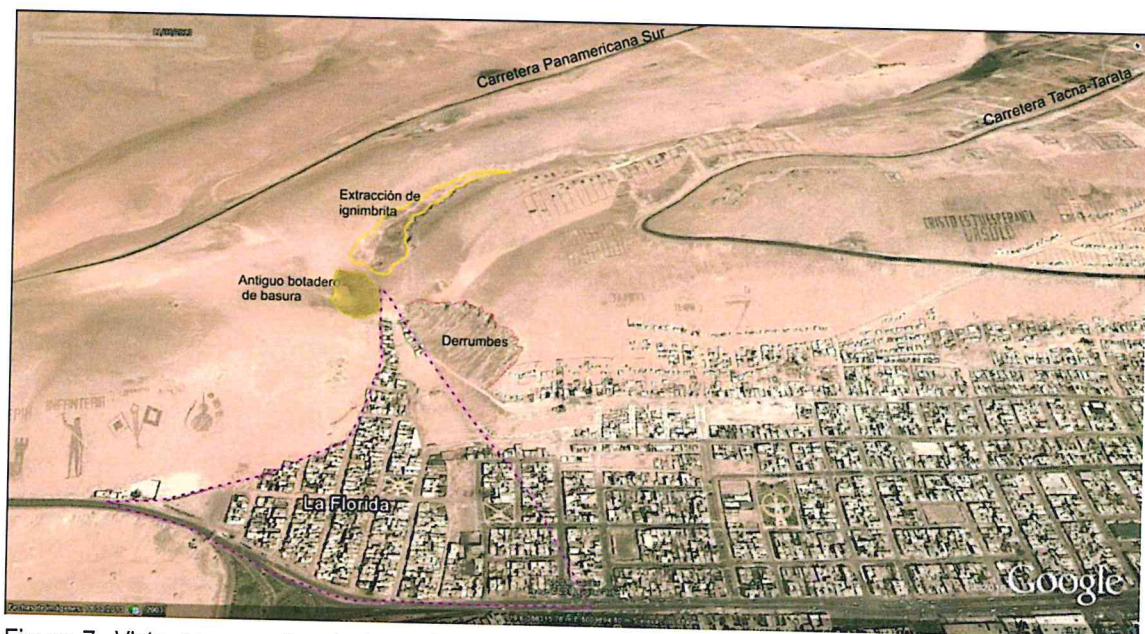
Figura 7. Vista aguas arriba de la quebrada Del Diablo obstruido por la construcción de viviendas, desmontes y botadero de basura (marcado con línea roja). La Florida se ubica asentado sobre el depósito antiguo de la quebrada Del Diablo.
