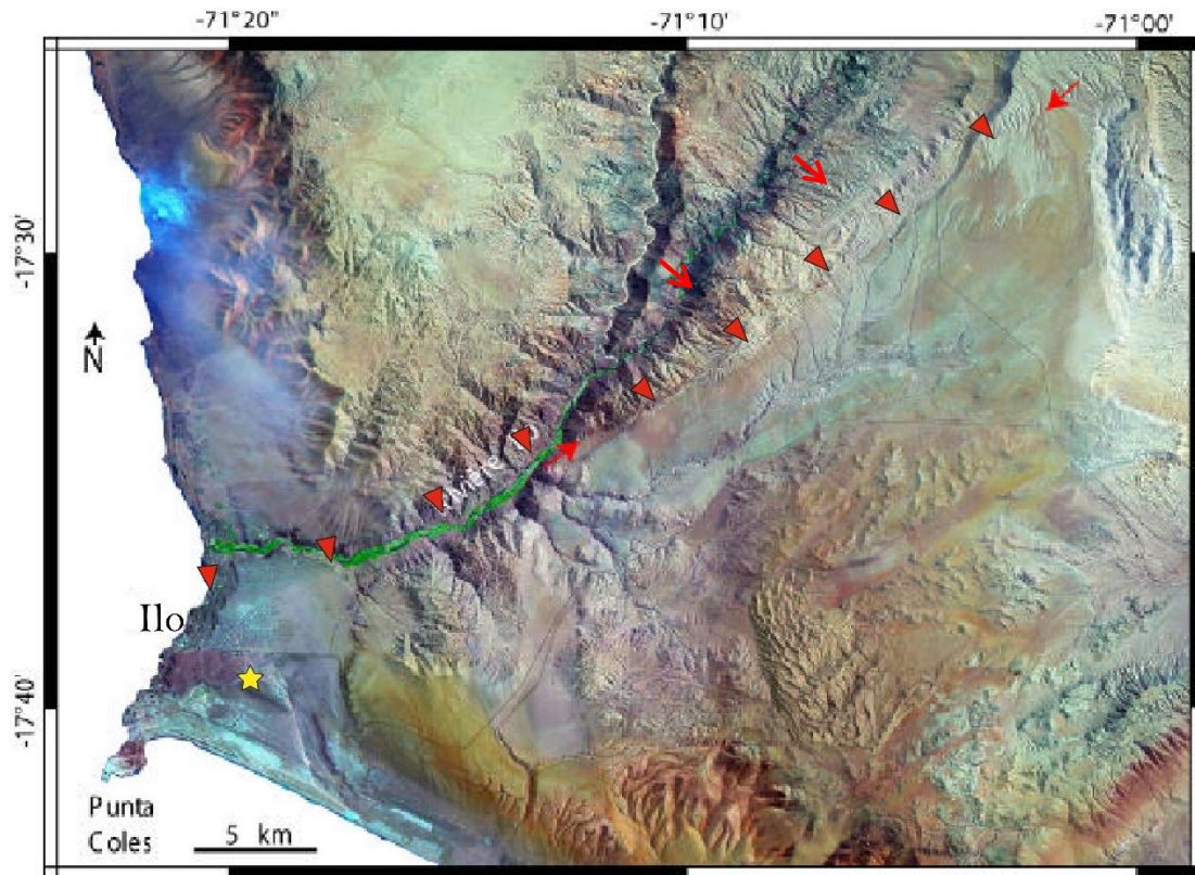
Figura 2. Ubicación de la falla Chololo, obsérvese las flechas rojas que indican el trazo de la falla. En estrella amarilla el predio de la SBN en consulta.
