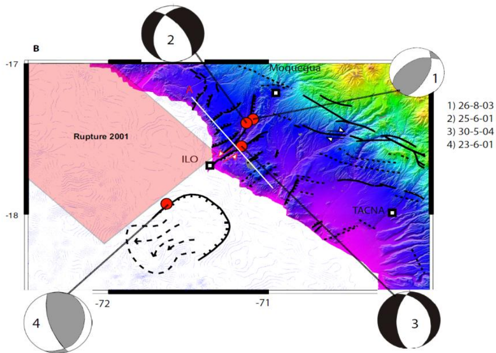
Figura 6. Imagen SRTM data donde se observa la traza de la falla Chololo y los sismos que se registraron después del sismo de Arequipa del año del 2001.
