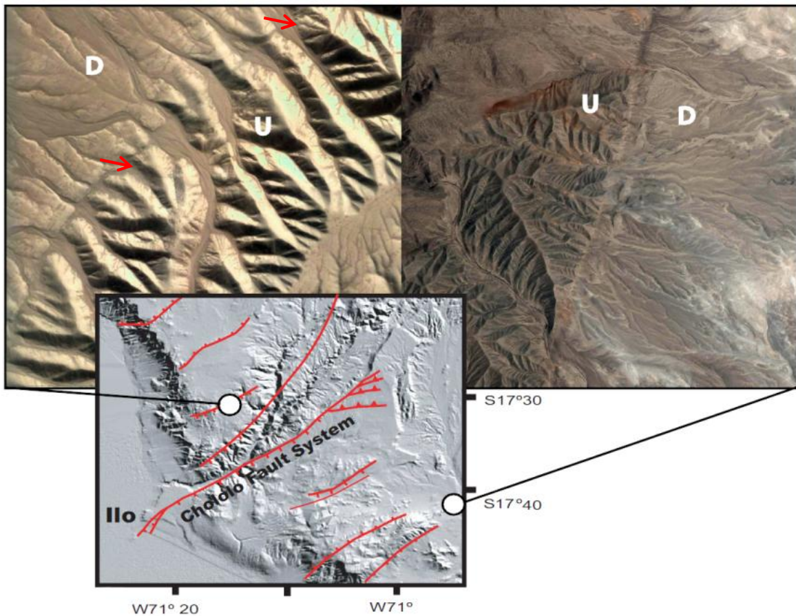
Figura 4. Detalle de dos de los segmentos de la Falla Chololo, imágenes Quickbird de Google Earth. Tomado de Audin et al., 2008
