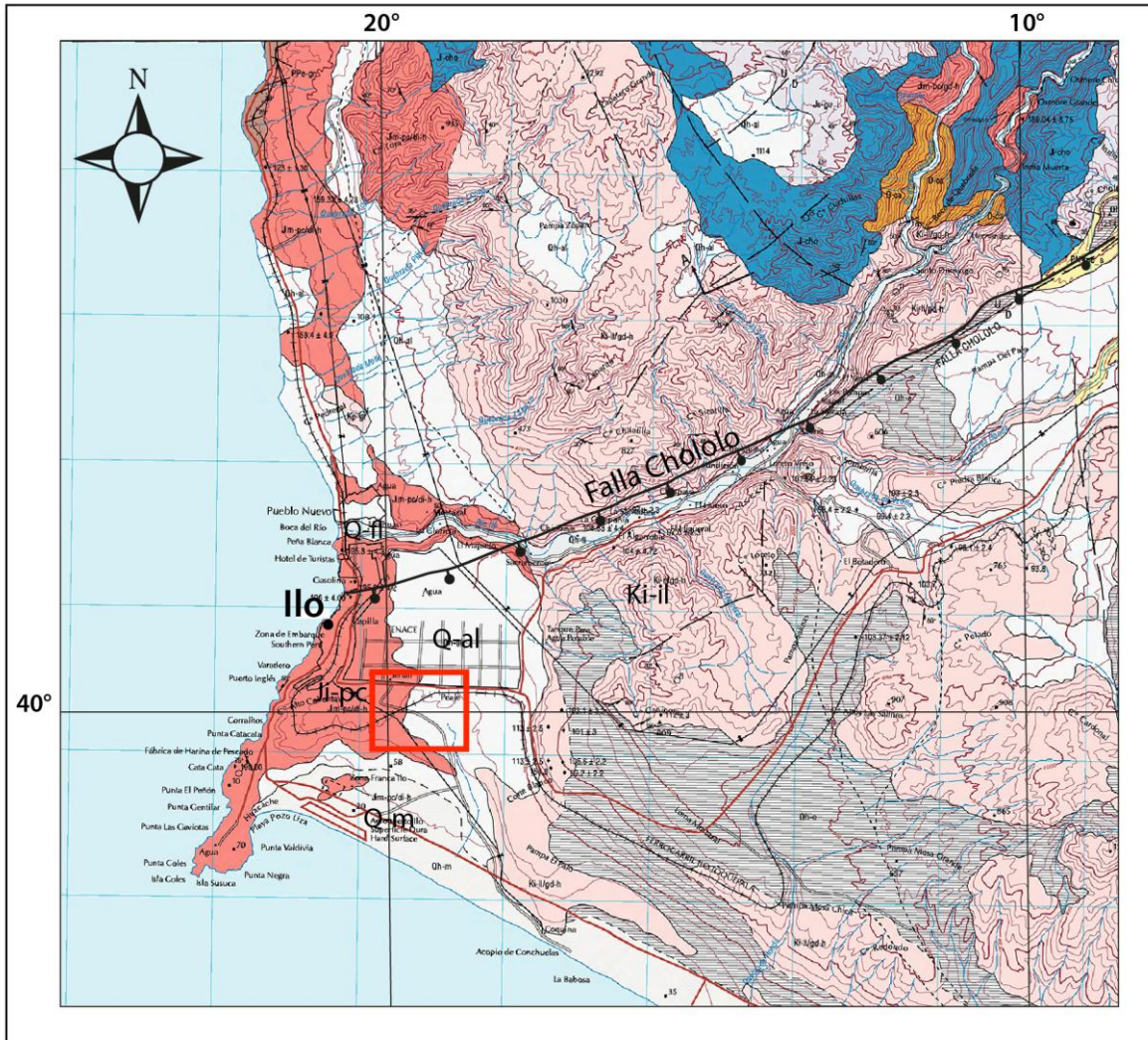
Figura 1. Mapa geológico del INGGEMMET, Hoja 36-t, Cuadrángulo de Ilo (Sanchez, et al. , 2000). El cuadrado con borde rojo indica el área de evaluada.
