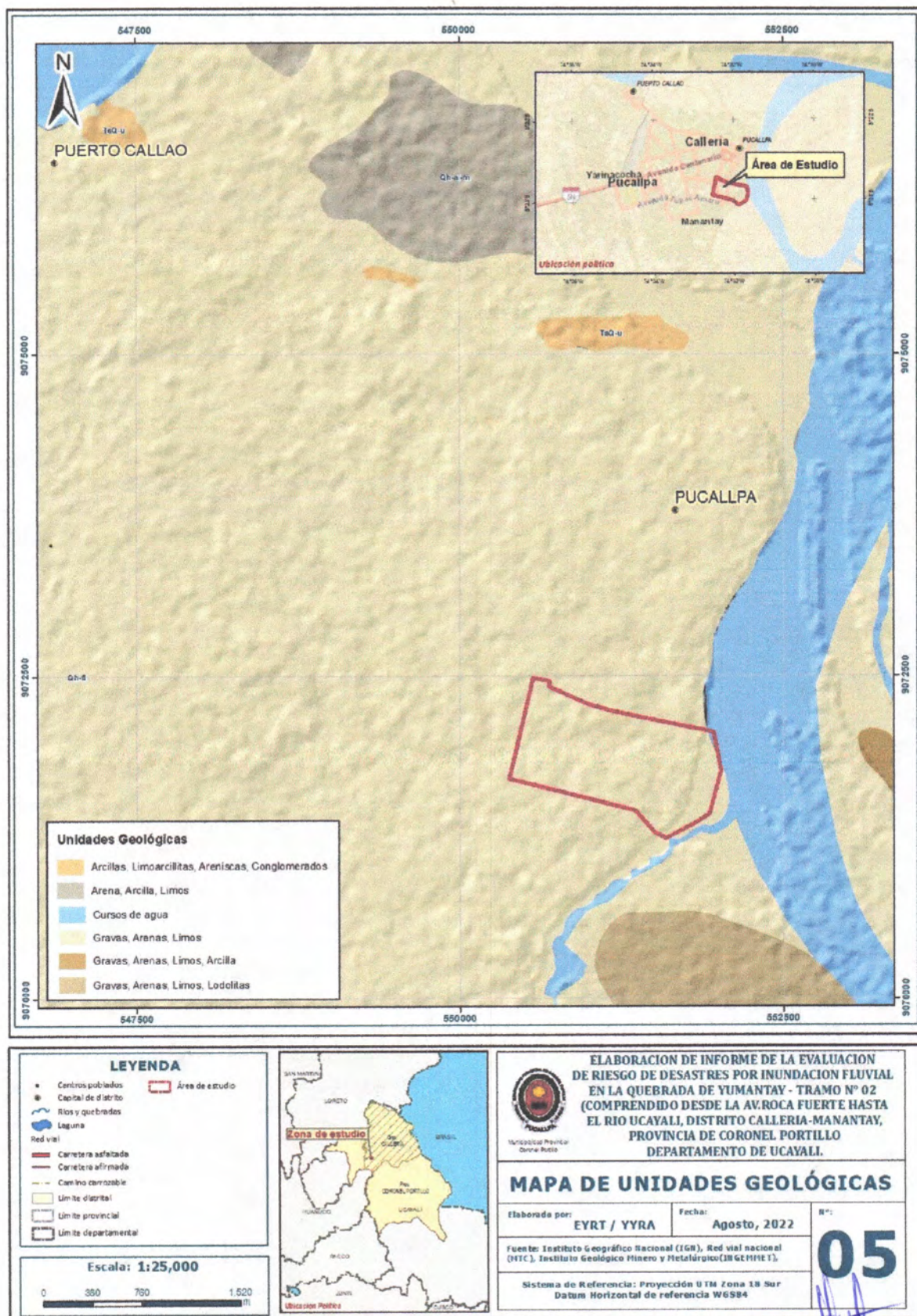
Figura N° 5. Mapa de Unidades Geológicas del área de estudio.
