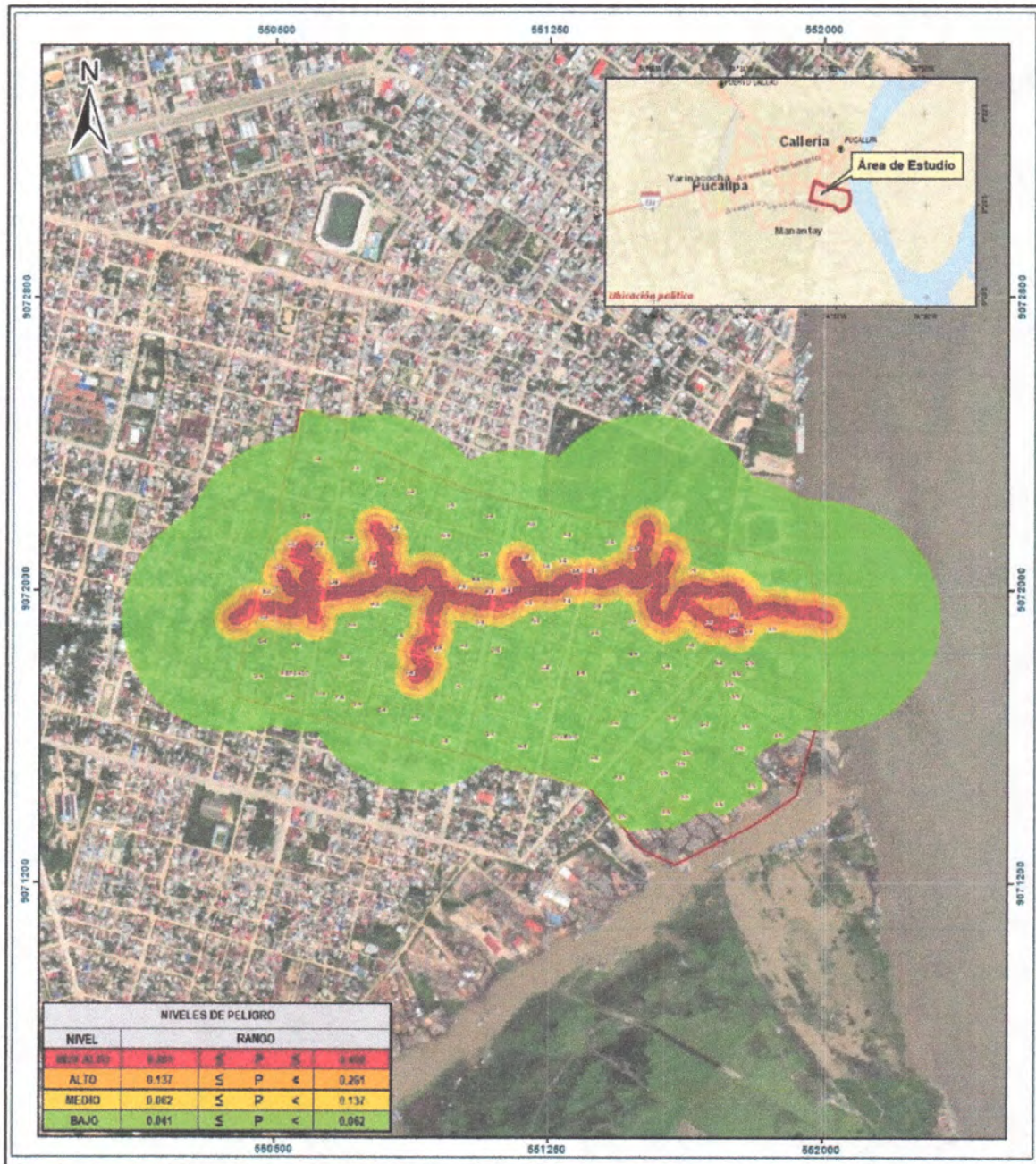
Figura N° 13. Mapa de peligro de inundación fluvial del área de estudio.
