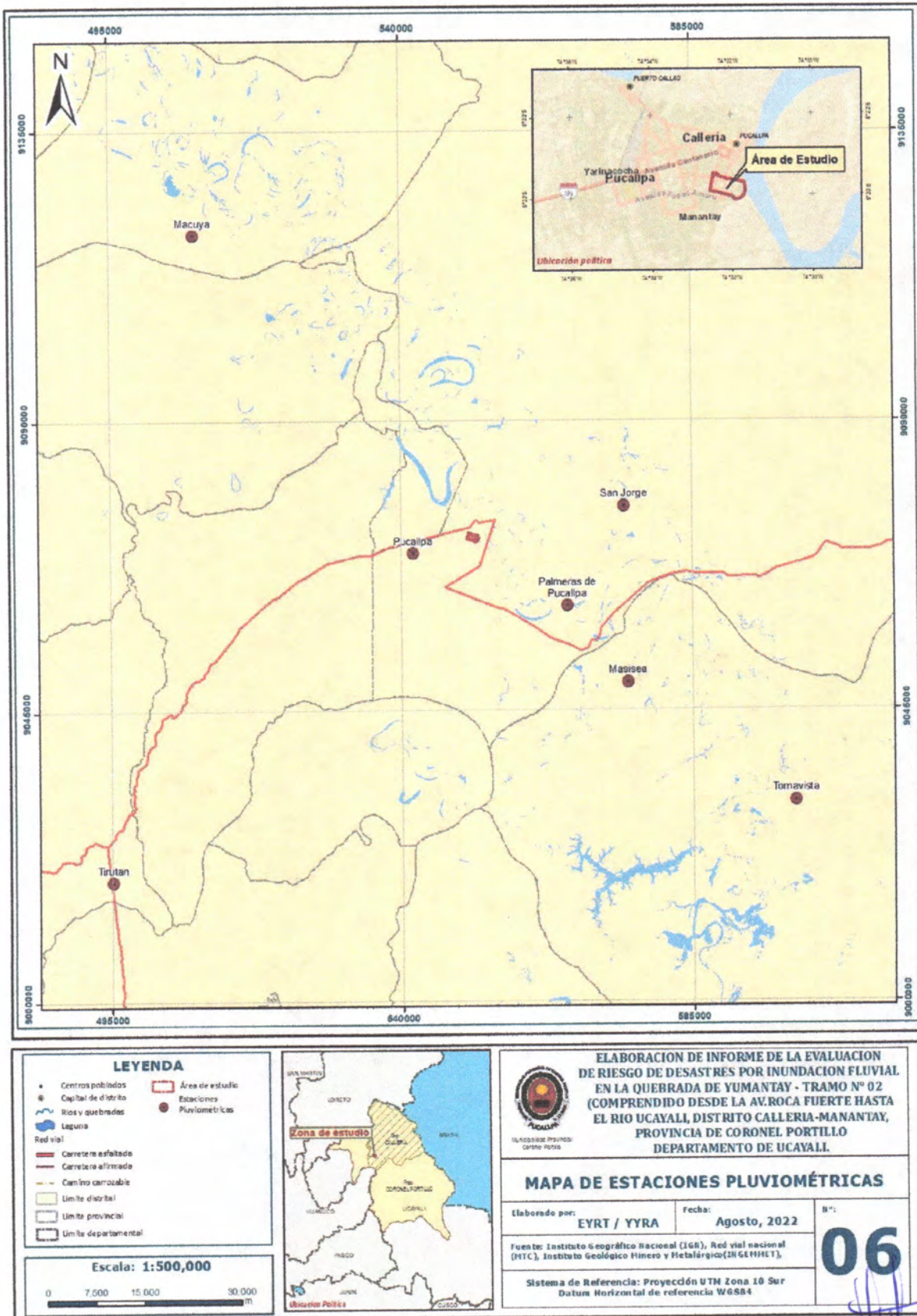
Figura N° 6. Mapa de estaciones pluviométricas.
