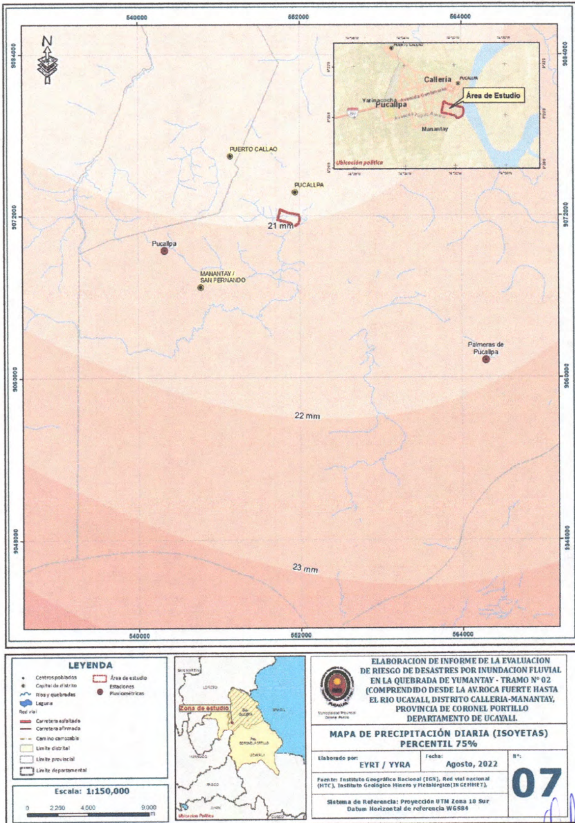
Figura N° 7. Mapa de precipitación diaria – percentil 75%.
