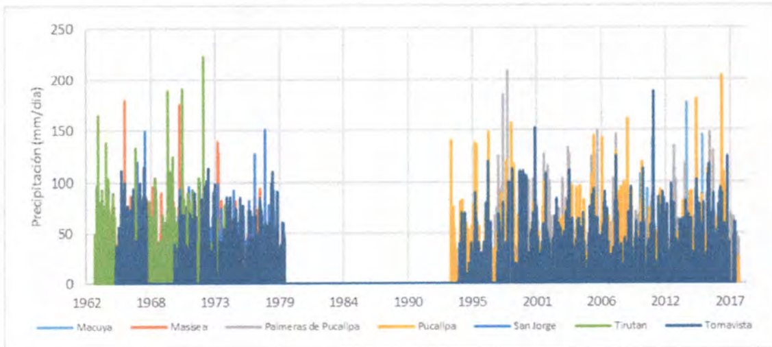
Gráfico N° 11. Series de precipitación a nivel diario (mm/día).
