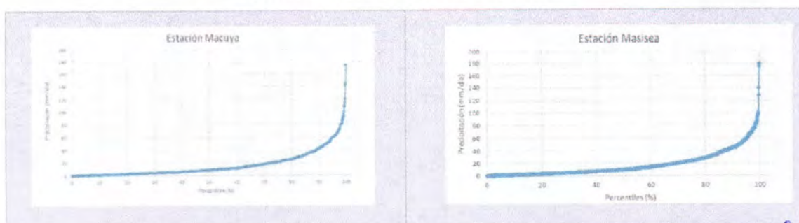
Gráfico N° 12. Percentiles de precipitación.
