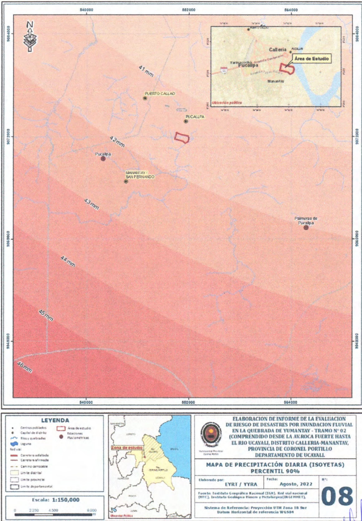
Figura N° 8. Mapa de precipitación diaria – percentil 90%.
