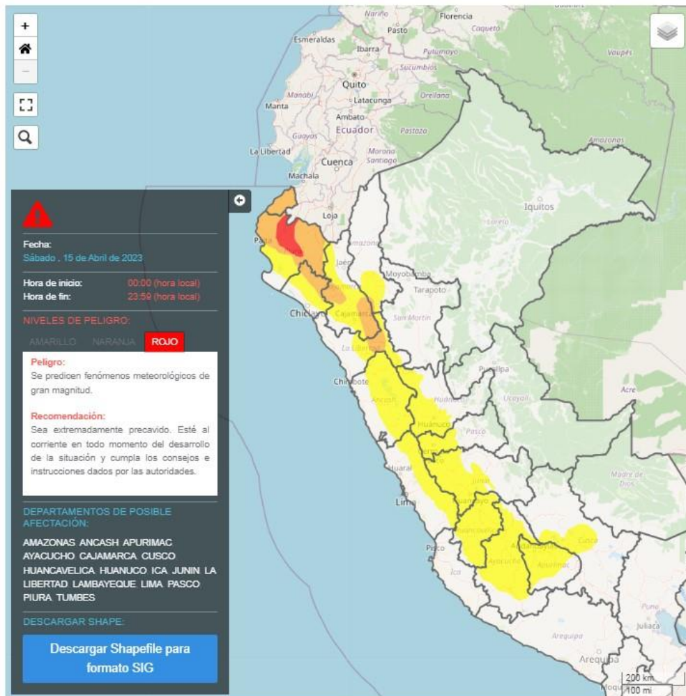
Figura 2. Pronóstico de precipitaciones en la costa norte y sierra del 15 de abril del 2023
