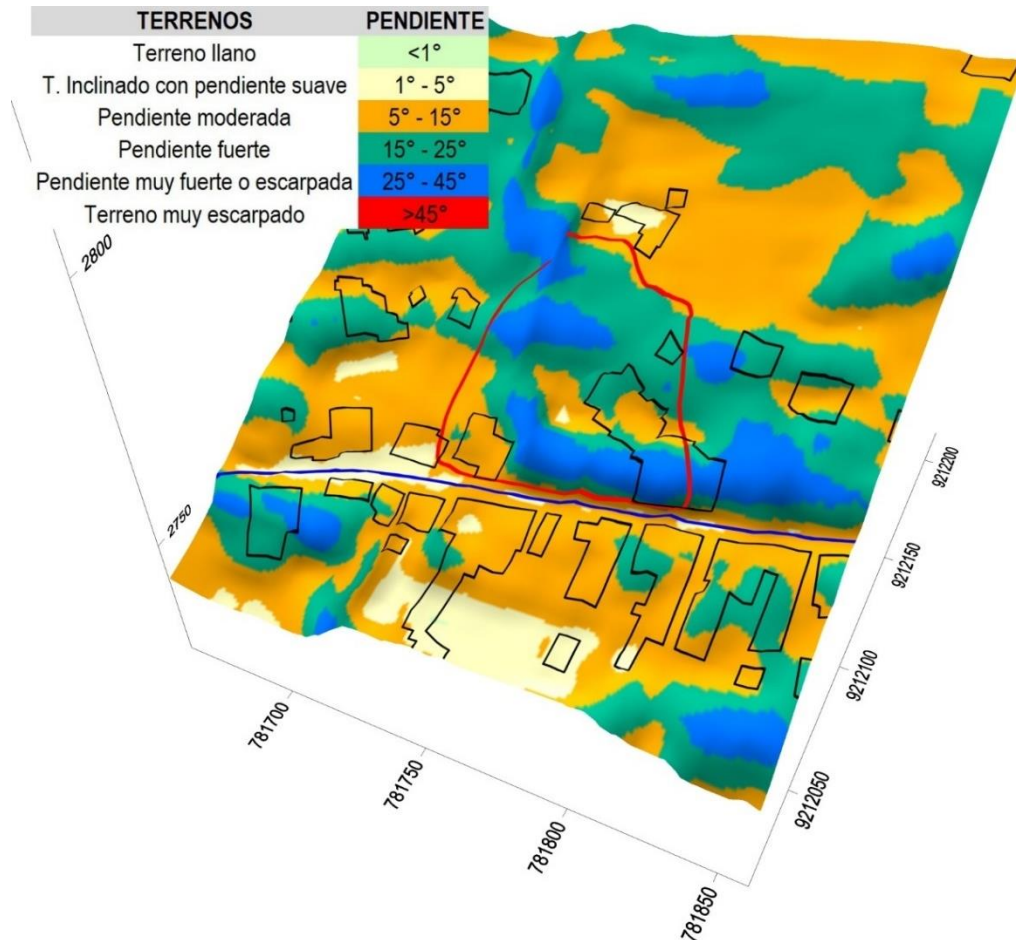
Figura 4. Modelo 3D de las pendientes del caserío Rinconada de Otuzco; el deslizamiento activo está delimitado en línea roja, dentro del cual se encuentran las viviendas afectadas delimitadas con líneas de color negro.
