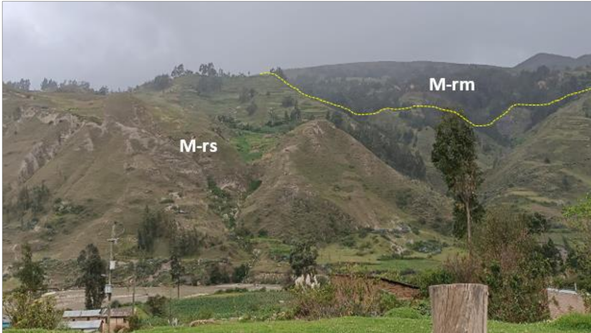
Figura 11. Vista con dirección al sureste, se observa el contacto de las subunidades geomorfológicas conformadas por montaña en roca sedimentaria (M-rs) y montaña en roca metamórfica (M-rm).
