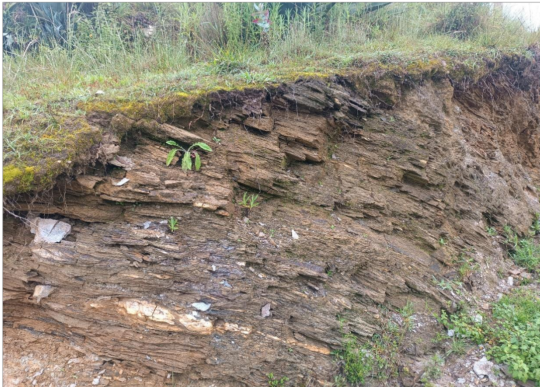
Fotografía 1. Afloramientos de esquistos meteorizados y muy deleznales pertenecientes al Complejo Marañón.
