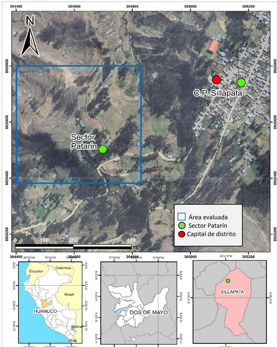
Figura 2. Ubicación del sector Patarín, al suroeste del C.P. Sillapata
