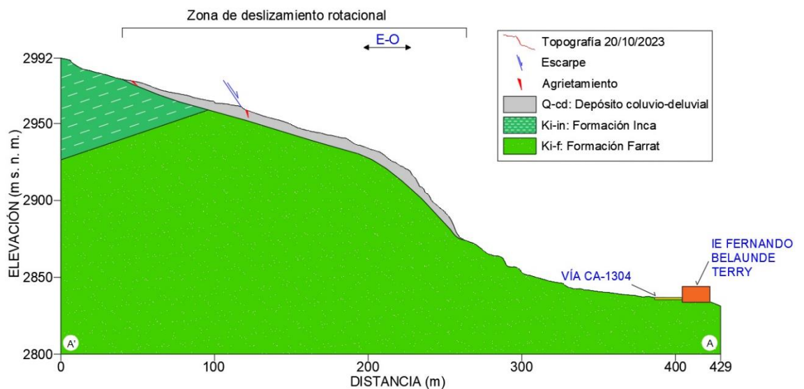
Figura 9. Perfil longitudinal A-A' que representa la distribución de los materiales geológicos y la institución educativa expuesta a daños.
