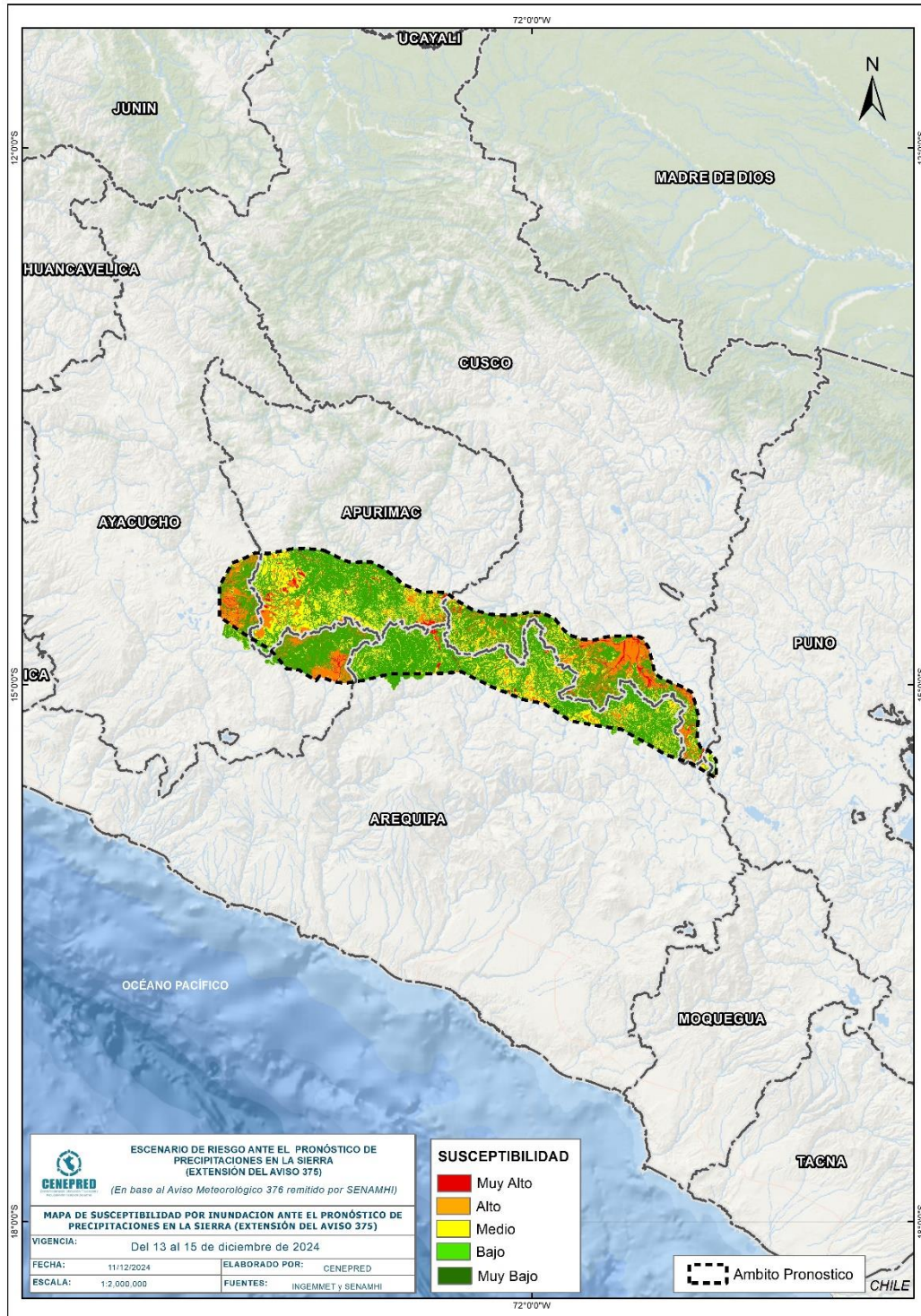
Figura 7. Escenario de riesgo por inundaciones en el ámbito del pronóstico de precipitaciones en la sierra del 13 al 15 de diciembre del 2024
