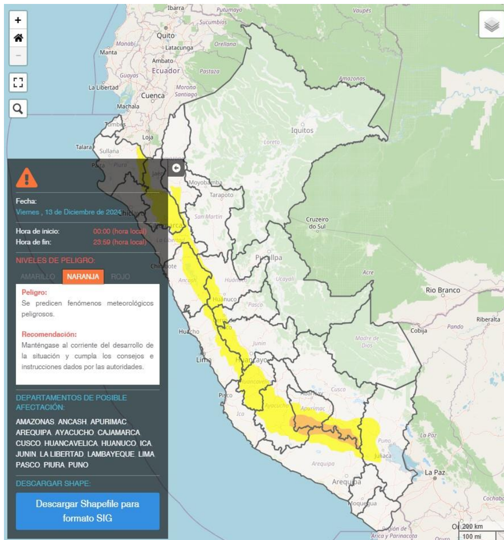
Figura 2. Pronóstico de precipitaciones en la sierra del 13 de diciembre del 2024
