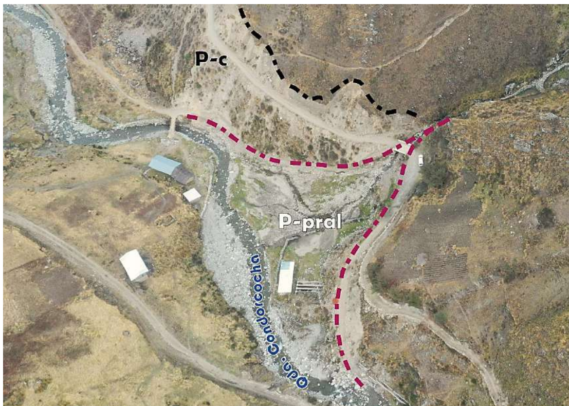
Figura 12. Vista de la subunidad de piedemonte proluvial o aluvio-torrencial (P-pral) reconocida en la quebrada Jayas, afluente a la quebrada Condorcocha. A su alrededor se observan geoformas de piedemonte coluvial (P-c).
