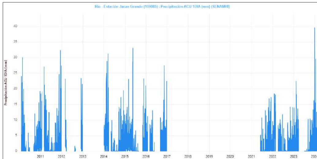
Figura 5. Precipitaciones máximas acumulada en mm, distribuidas a lo largo del periodo enero, 2010 – febrero, 2024. Fuente: https://snirh.ana.gob.pe/VisorPorCuenca/ .
