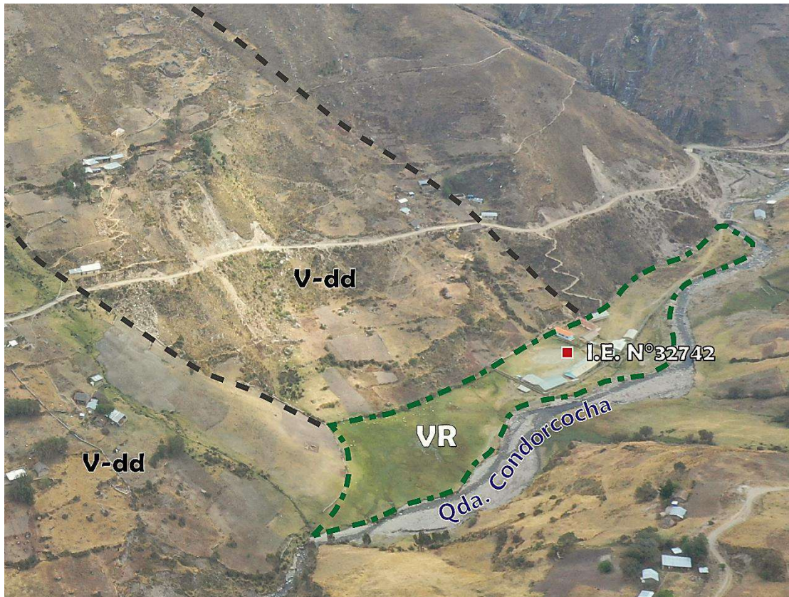
Figura 13. Vista de la subunidad valle de represamiento (VR), formado por el embalse de la quebrada Condorcocha a consecuencia de movimientos en masa antiguos apreciándose una superficie plana. En la actualidad la I.E. N°32742 se asienta sobre esta geoforma. Vista aguas arriba.
