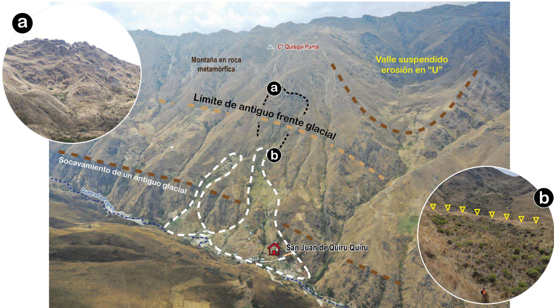
Figura 14. Evidencias geomorfológicas originadas de la dinámica glacial, periglacial y procesos de movimientos en masa que demarcan el relieve actual. a. Procesos de gelifracción (desintegración mecánica de la roca, como consecuencia del aumento de presión del agua congelada contenida en diaclasas, poros y fracturas). b. Escarpes de deslizamiento antiguo condicionado a partir de procesos de erosión, transporte y acumulación del periglacialismo. En líneas entrecortadas blancas se observa el deslizamiento-flujo y sobre el cual se asienta actualmente la población.
