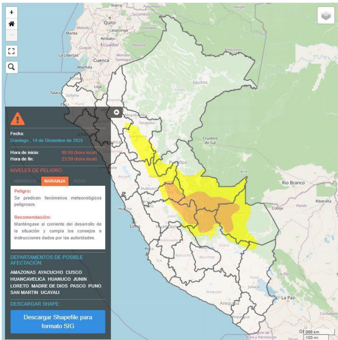
Figura 2. Pronóstico de lluvia en la selva del 14 de diciembre del 2025
