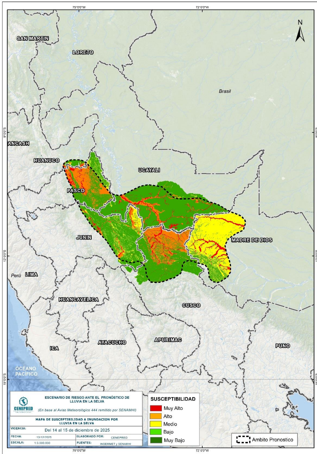
Figura 6. Escenario de riesgo por inundaciones en el ámbito del pronóstico de lluvia en la selva del 14 al 15 de diciembre del 2025
