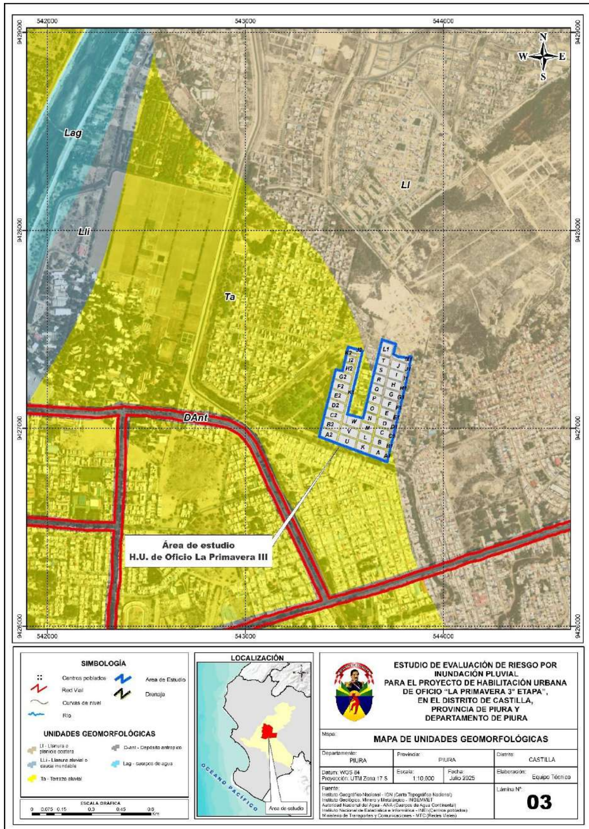
Figura 4. Mapa Geomorfológico
