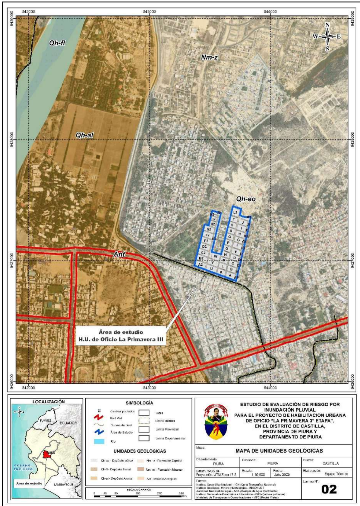
Figura 3. Mapa Geológico
