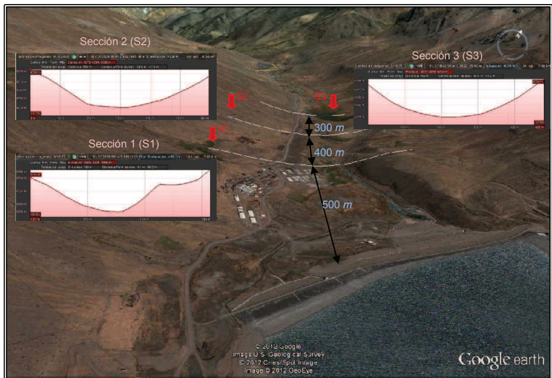
Figura 4-5: Forma del valle aguas abajo de la presa Yuracmayo
