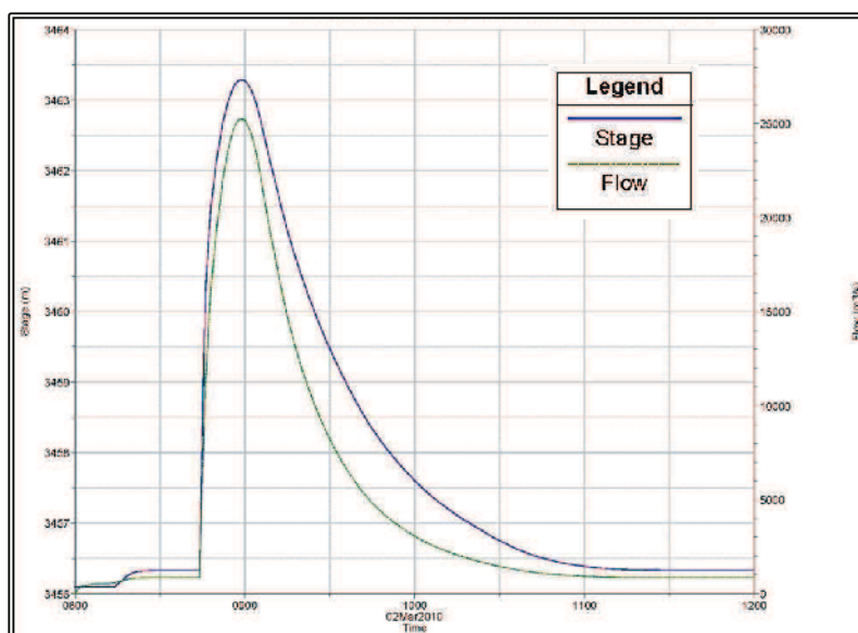
Figura A-3: Hidrograma en la sección 27
