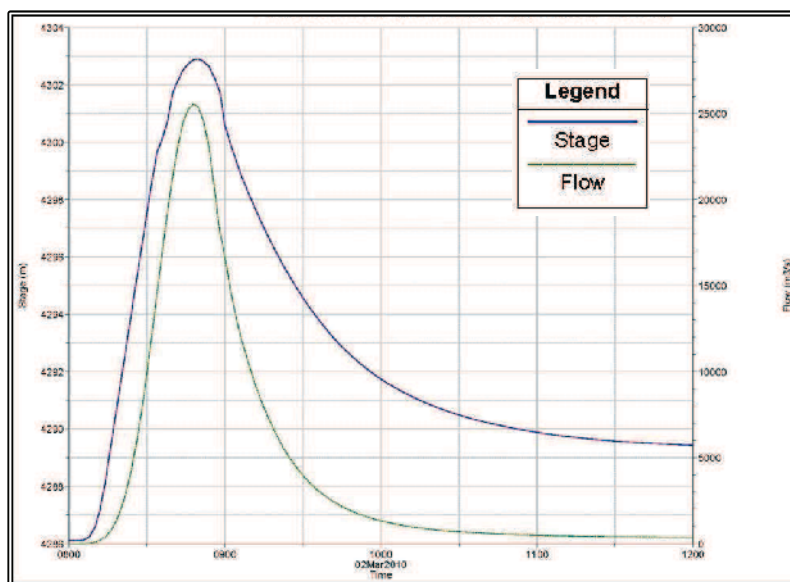
Figura A-2: Hidrograma en la sección 19432
