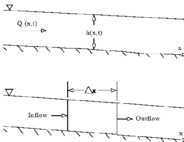
Figura 3-5: Volumen de control elemental para la derivación de las Ecuaciones de Continuidad y Momento
