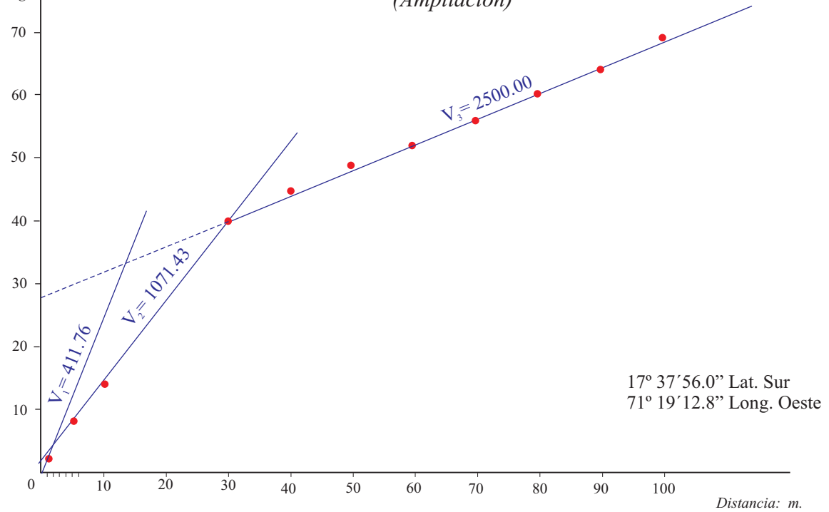
Perfil de Refracción Sísmica 12
