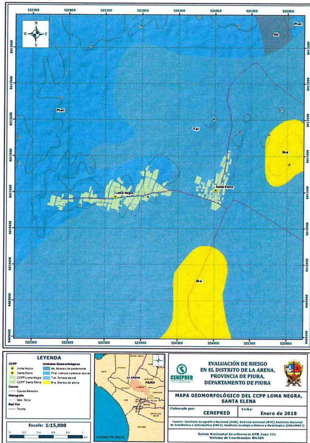
Figura 3. Mapa de Geomorfológico del CCPP Loma Negra-Santa Elena
