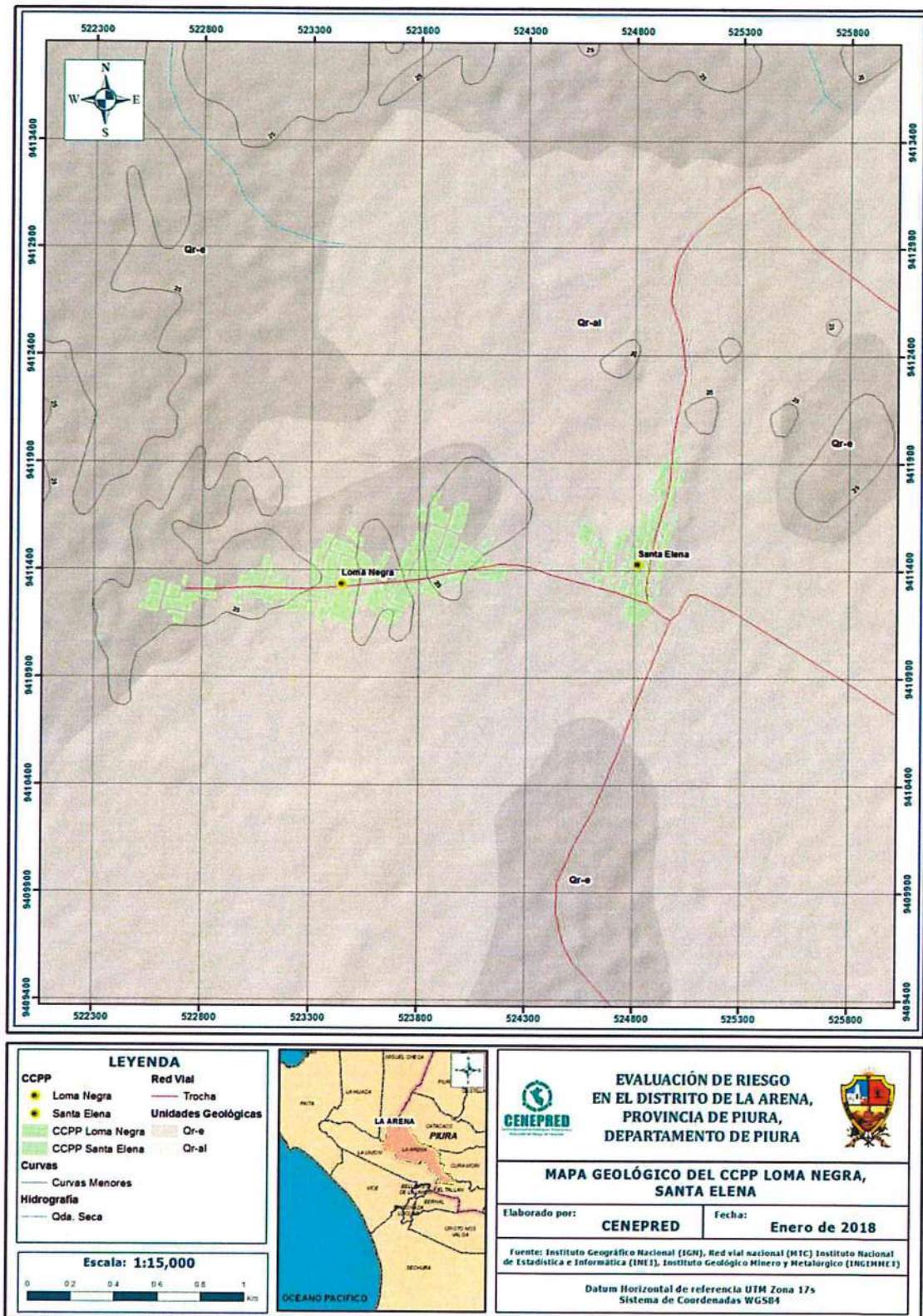
Figura 2. Mapa de Geología Local del CCPP Loma Negra-Santa Elena
