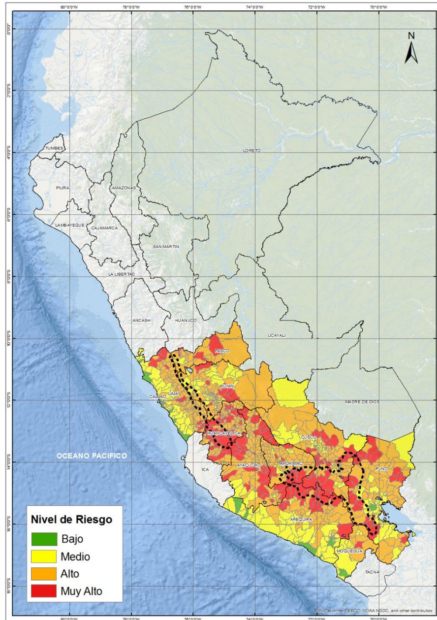
Figura 4. Escenario de riesgo por movimientos en masa en base al pronóstico de precipitación para el periodo del 25 al 28 de abril de 2018
