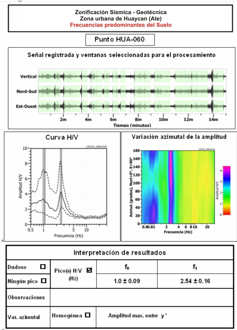
Figura 27: Ejemplo de la ficha H/V para el punto HUA-060 en la cual se recopila la información registrada y analizada. Arriba, señal registrada; Medio; razón espectral (H/V) en línea gruesa y su desviación estándar en línea discontinua. Espectrograma y Abajo: resultados.
