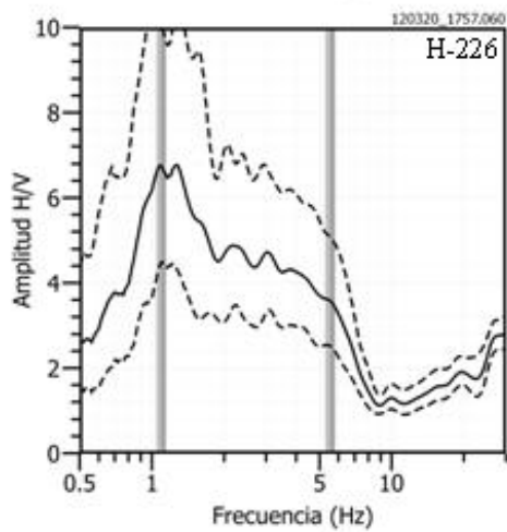
Figura 29: .../Continuación. Ejemplos de Razones espectrales (H/V) donde la frecuencia predominante sobresale en el rango de 0.5 - 3.0Hz. Las líneas continuas, representan la razón espectral y las discontinuas su desviación estándar. Las barras grises, definen la frecuencia predominante en este rango de frecuencias bajas.
