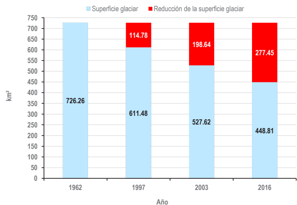
Gráfico 9. Reducción del área glaciaria por periodos (1962-2016).
