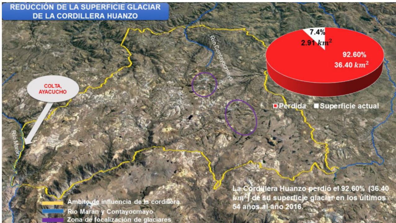
Figura 23. Reducción de la superficie glaciaria en la Cordillera Huanzo.
