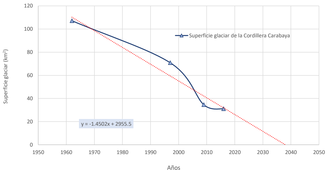
Gráfico 56. Tendencia estimada de la reducción de la superficie glaciaria de la Cordillera Carabaya.
