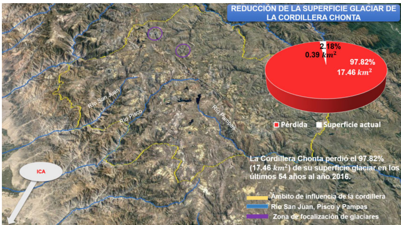
Figura 19. Reducción de la superficie glaciar en la Cordillera Chonta.
