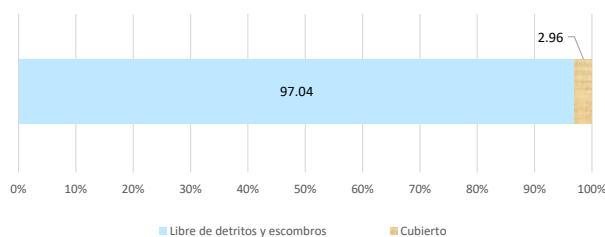
Gráfico 57. Proporción de superficies glaciares 2016 Cordillera Apolobamba.
