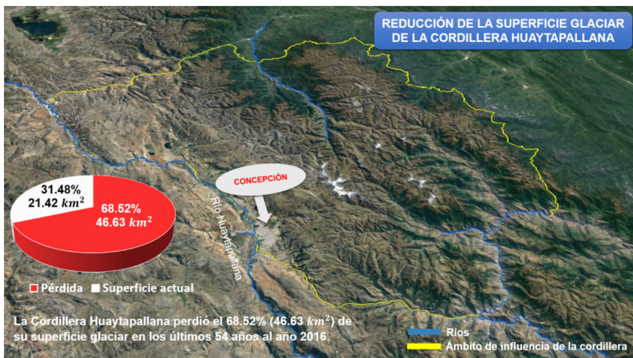
Figura 18. Reducción de la superficie glaciar en la Cordillera Huaytapallana.
