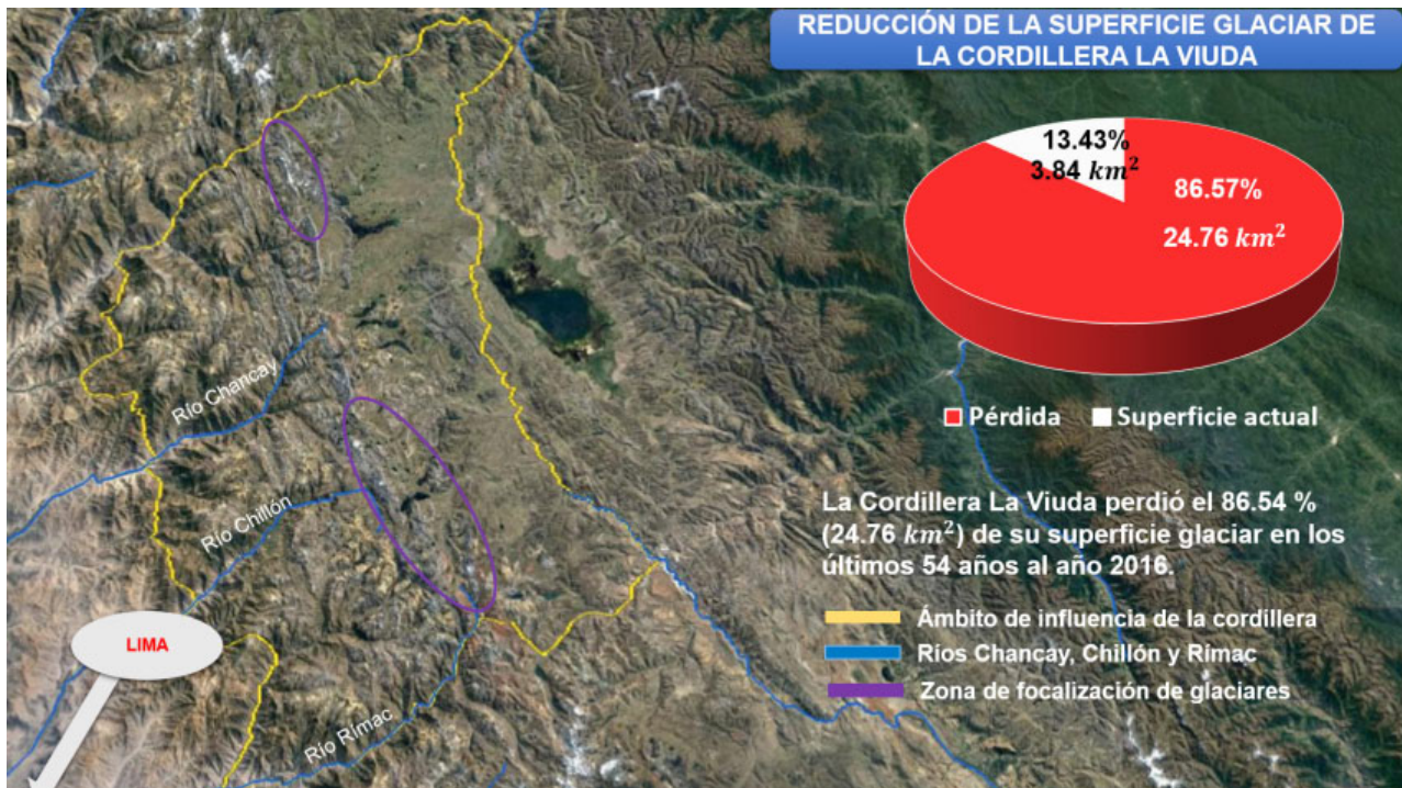
Figura 15. Reducción de la superficie glaciar en la Cordillera La Viuda.
