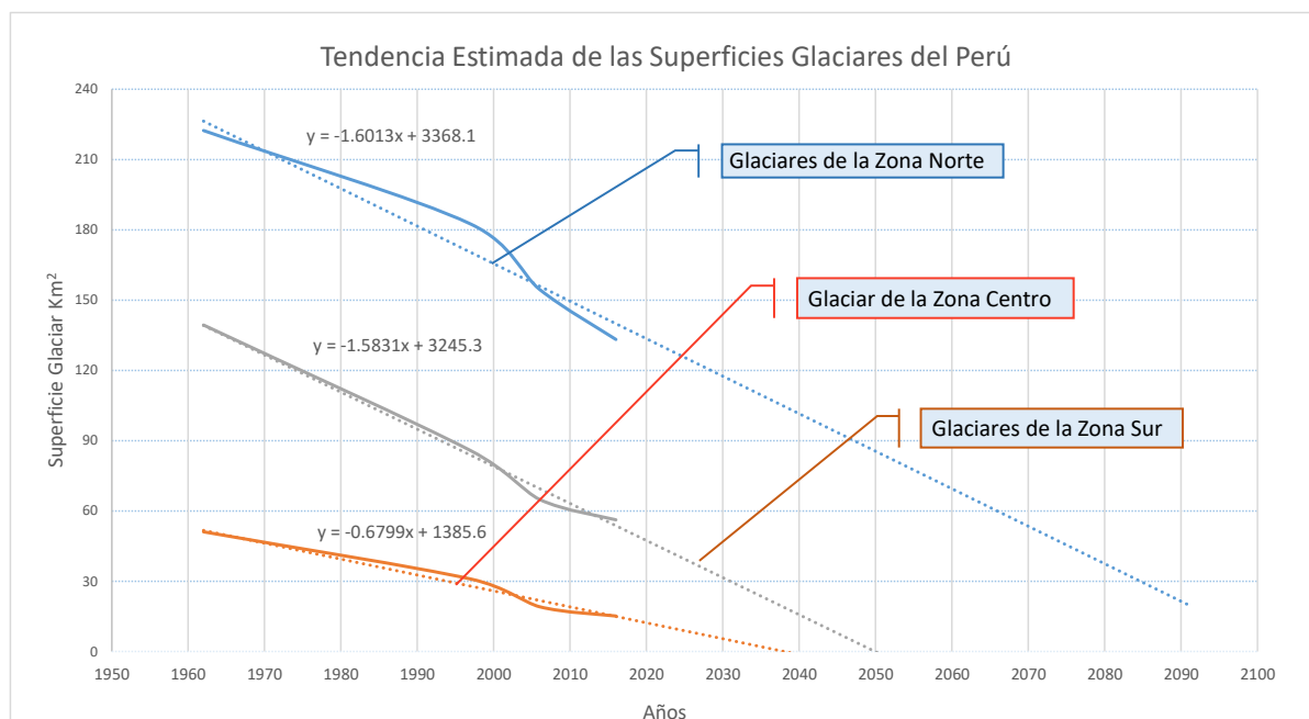
Gráfico 7. Tendencia estimada de la reducción de las superficies glaciares del Perú
