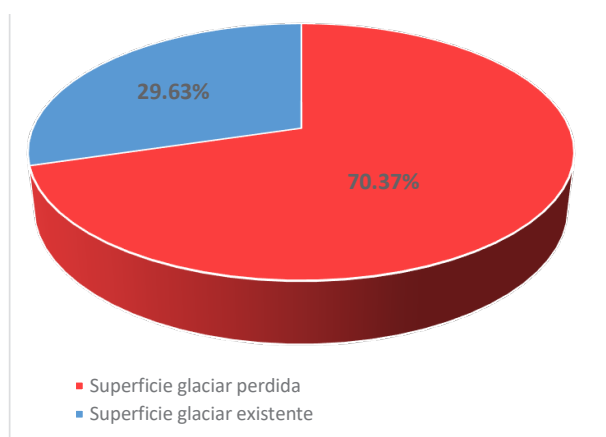
Gráfico 4. Reducción glaciaria en los Andes de la zona centro.
