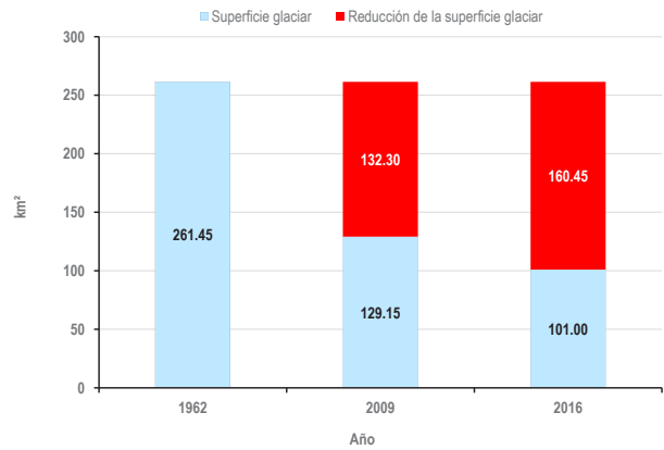
Gráfico 40. Reducción del área glaciaria por periodos (1962-2016) - Cordillera Vilcabamba
