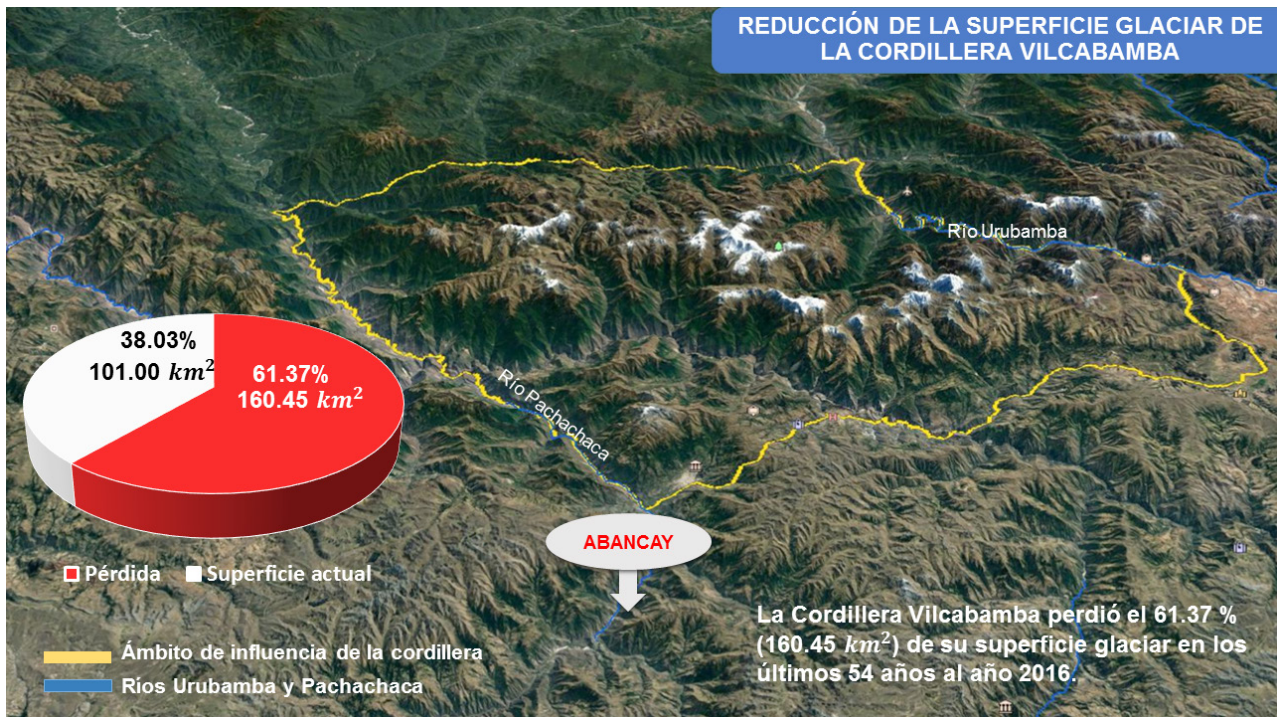
Figura 21. Reducción de la superficie glaciaria en la Cordillera Vilcabamba.
