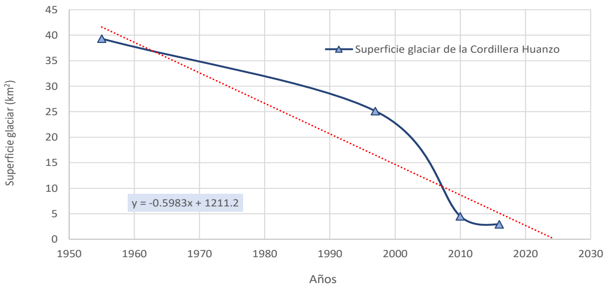
Gráfico 46. Tendencia estimada de la reducción de la superficie glaciaria de la Cordillera Huanzo.
