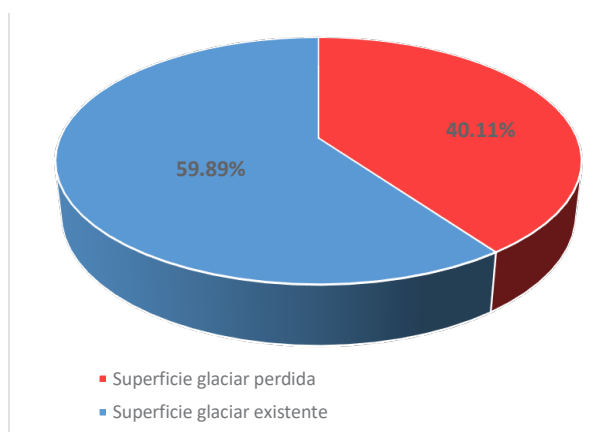
Gráfico 3. Reducción glaciaria en los Andes de la zona norte.
