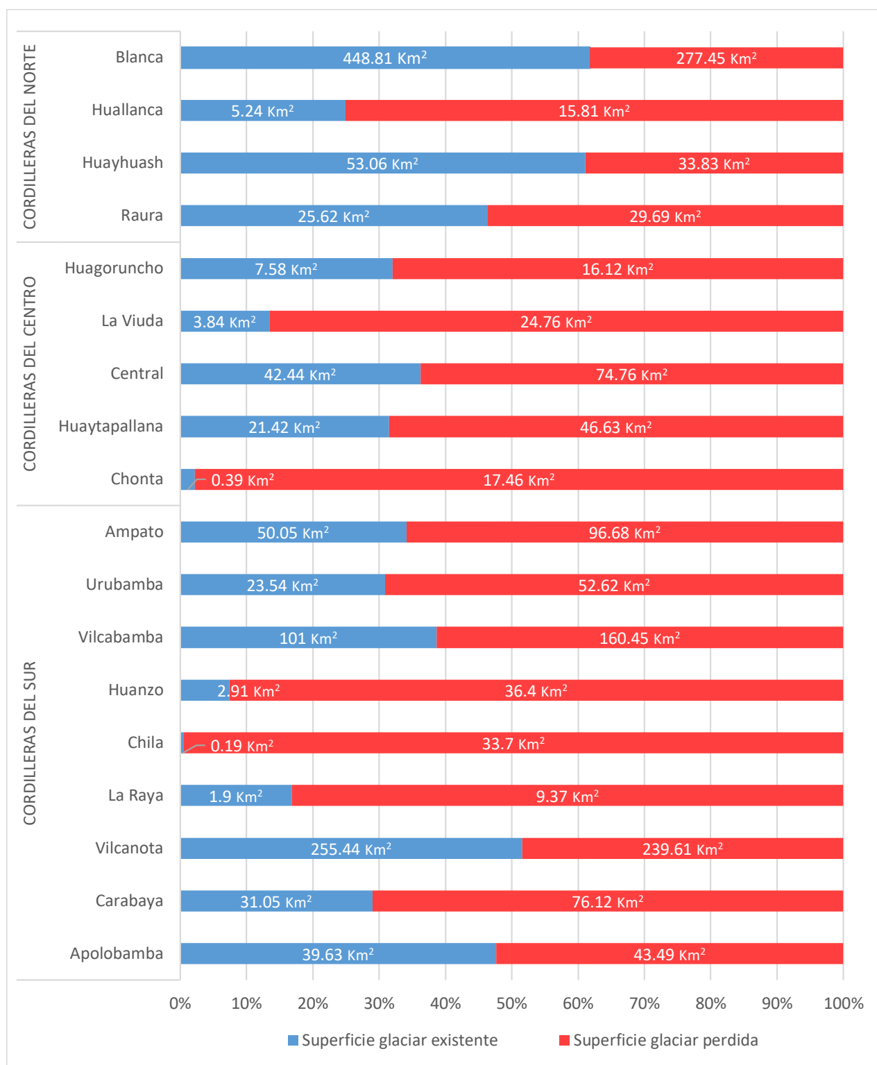
Gráfico 6. Reducción glaciaria porcentual por cada cordillera.
