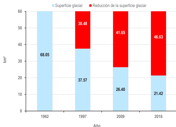
Gráfico 32. Reducción del área glaciar por periodos (1962-2016) - Cordillera Huaytapallana.
