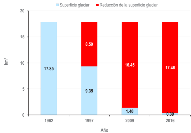
Gráfico 34. Reducción del área glaciar por períodos (1962-2016) - Cordillera Chonta.
