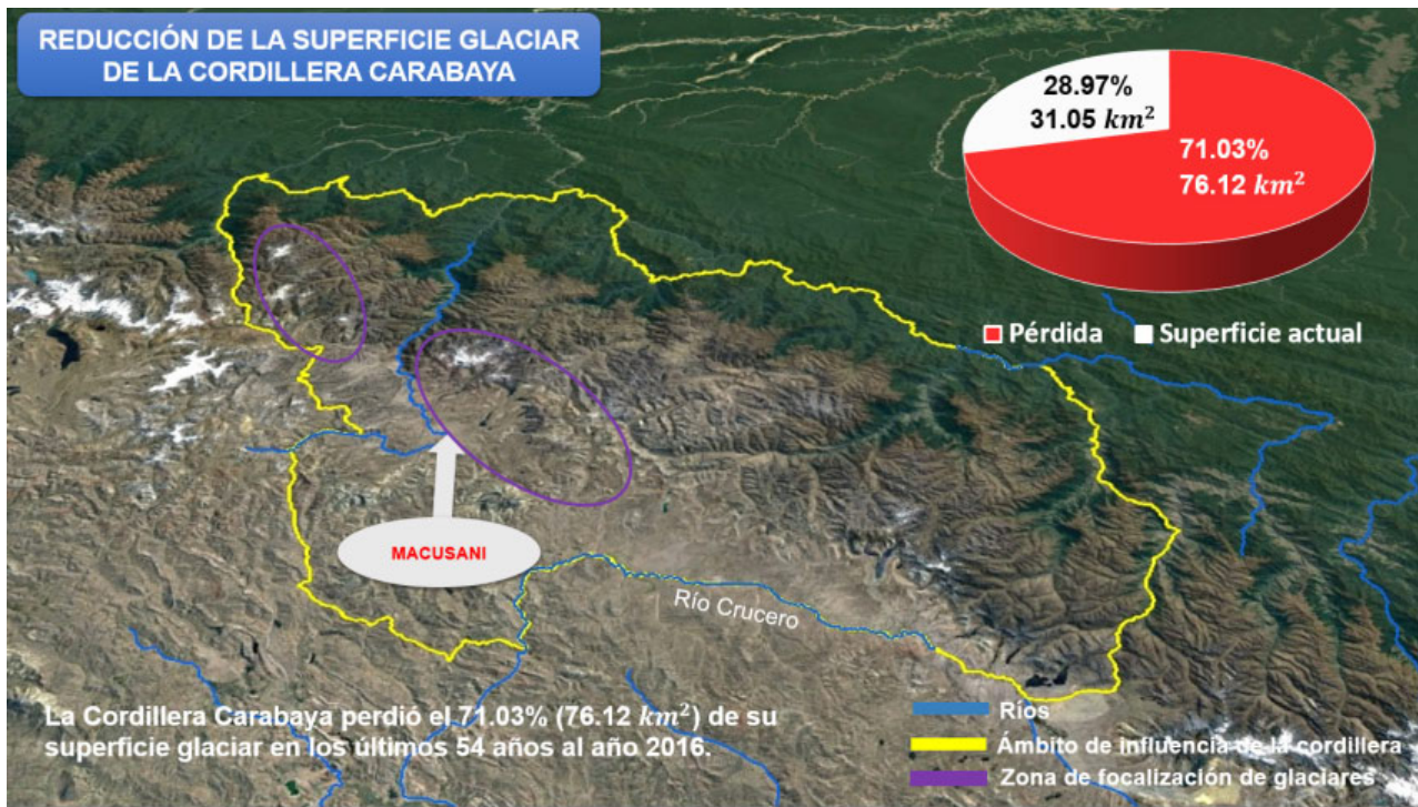
Figura 27. Reducción de la superficie glaciaria en la Cordillera Carabaya.
