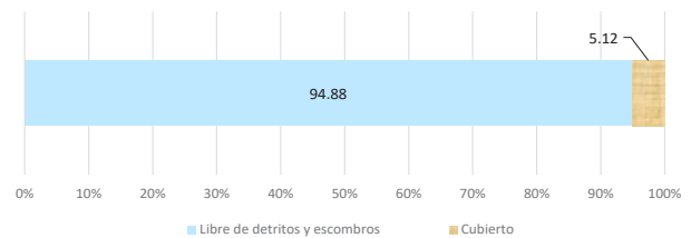
Gráfico 8. Proporción de superficies glaciares 2016 Cordillera Blanca
