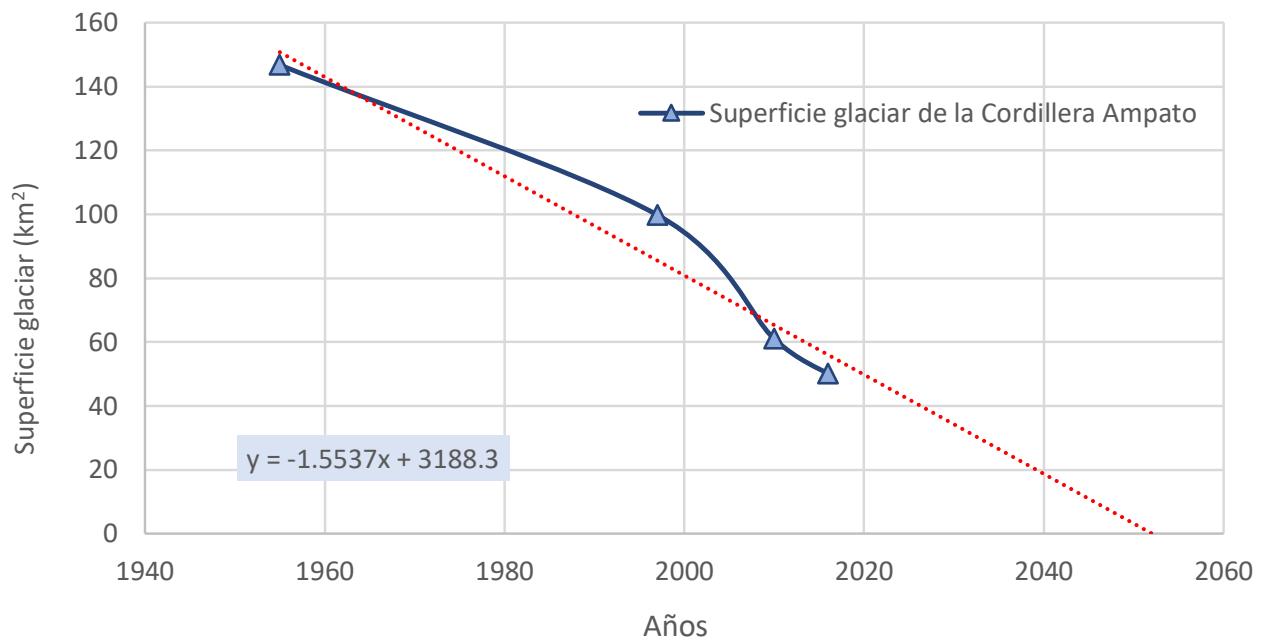
Gráfico 38. Tendencia estimada de la superficie glaciaria de la Cordillera Ampato.
