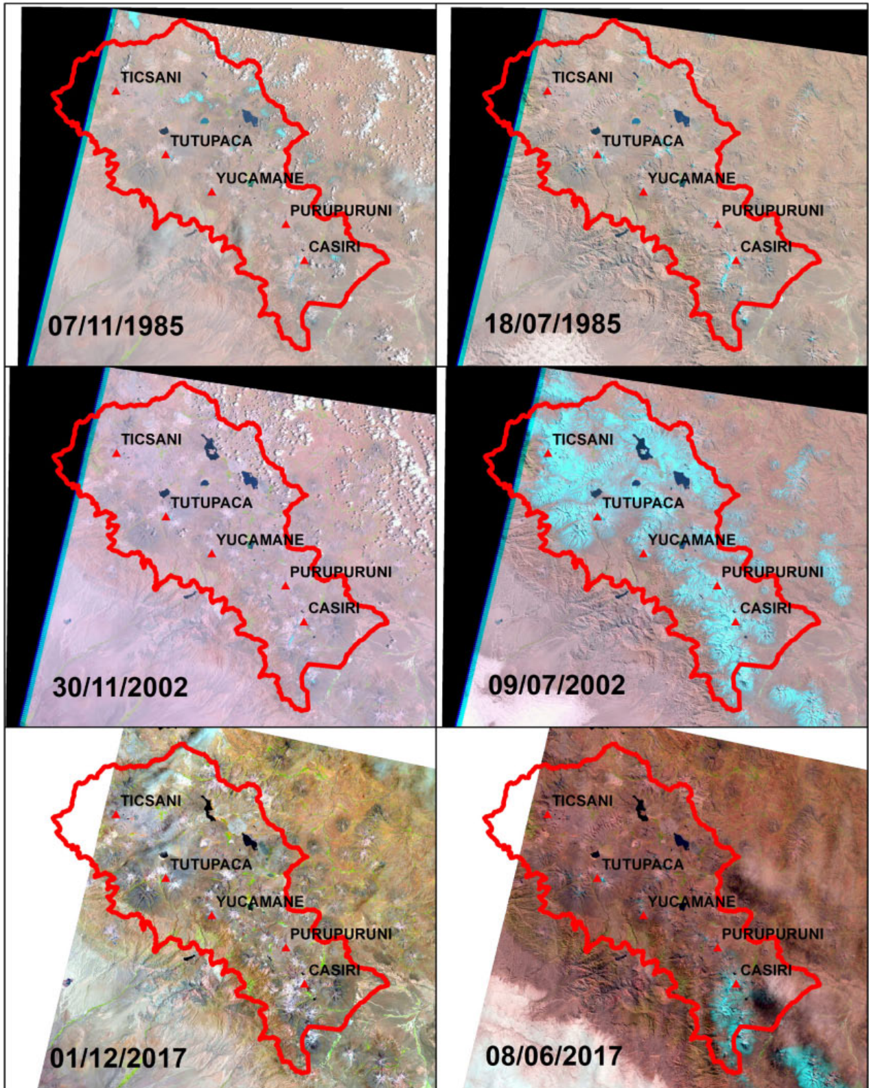
Figura 33. Análisis multitemporal de la cordillera Barroso mediante imágenes Landsat, donde se muestra los aportes de precipitaciones sólidas en forma de nevadas que muchas veces provocan confusión en que si aún hay masa glaciár. En la secuencia se observan periodos cuando el ámbito esta con cobertura nival y libre de nieve.
