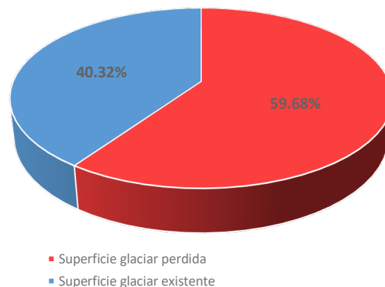
Gráfico 5. Reducción glaciaria en los Andes de la zona sur.
