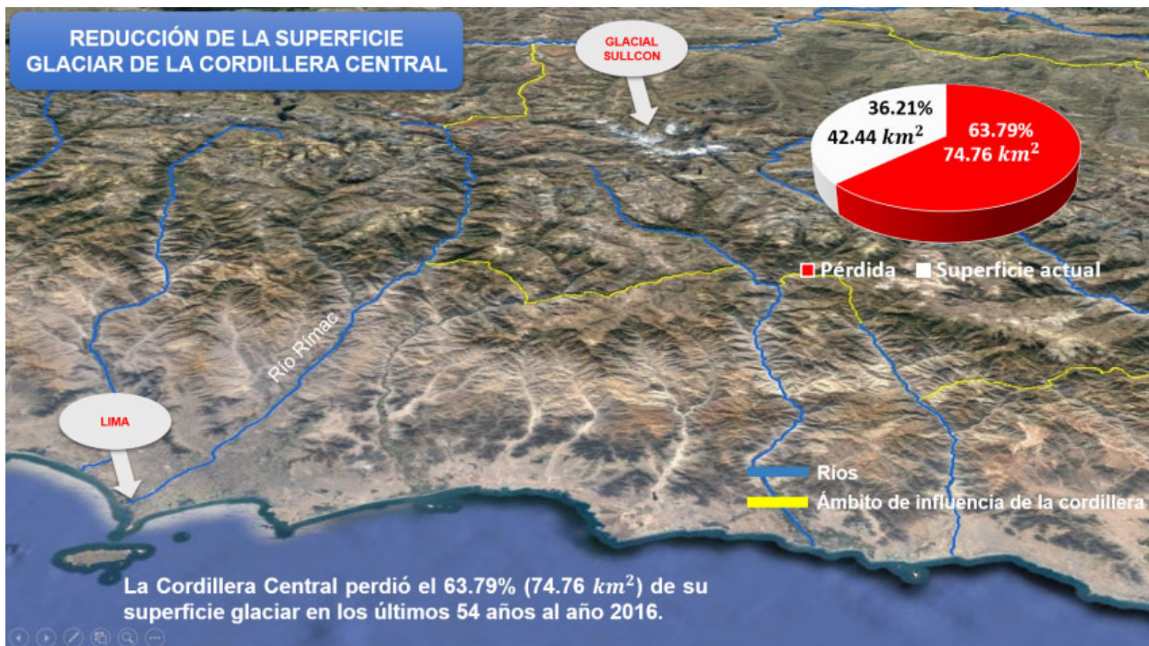
Figura 16. Reducción de la superficie glaciaria de la Cordillera Central.
