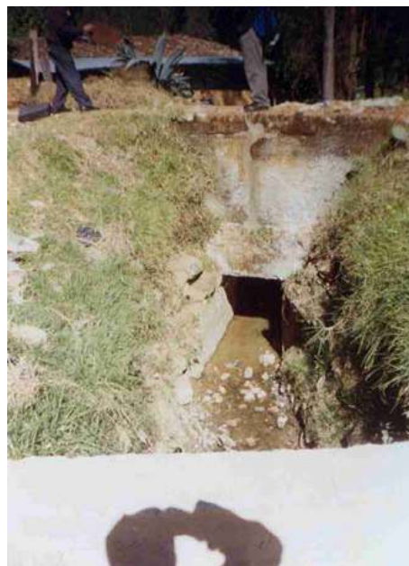
TRAMO CANALIZADO DE LA QUEBRADA SECA TINGO MAYO, EN EL PUNTO DONDE PASA POR ENCIMA DEL CANAL REMONTA 2
