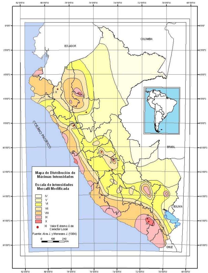
Figura 16: Curvas de intensidades máximas de Escala de Mercalli modificada.
