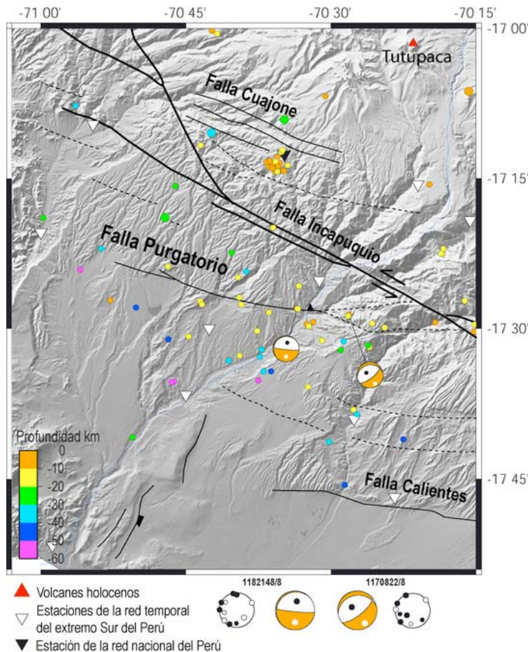
Figura 13: Sismicidad intracontinental y mecanismos focales entre 0 y 60 km de profundidad bajo la falla Purgatorio y mapeo tectónico.
