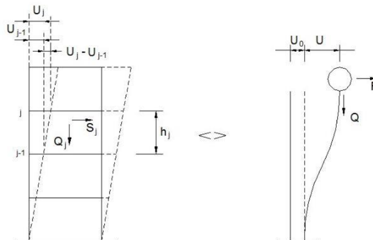
Figura 44. Edificación representada por un sistema equivalente
