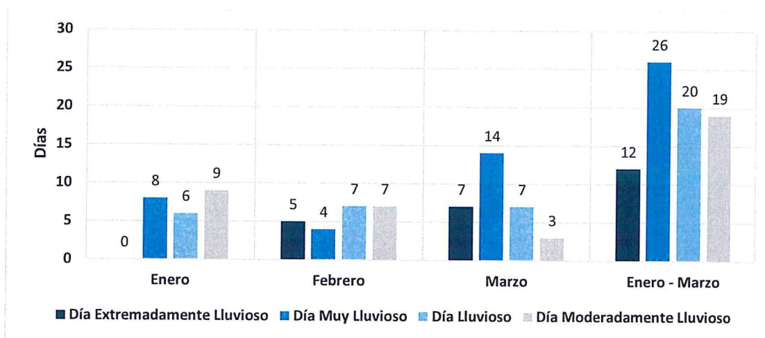
Gráfico 12. Frecuencia promedio de lluvias extremas durante El Niño Costero 2017 en el distrito de Frías
