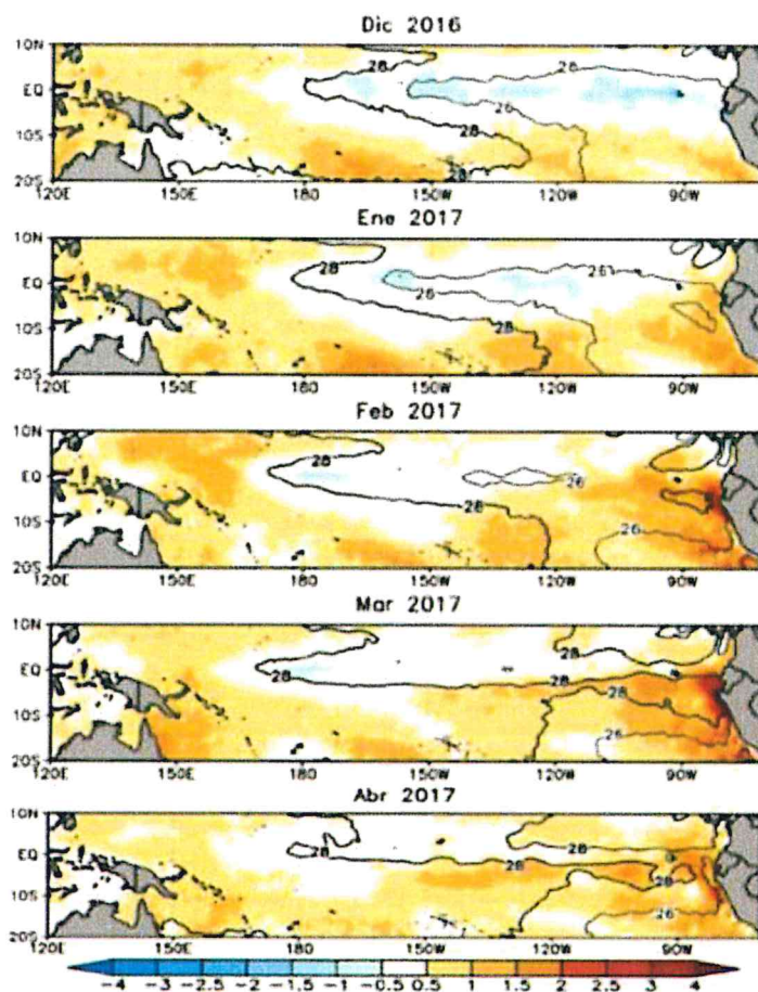
Gráfico 10. Anomalia de la Temperatura superficial del mar (°C) en el Pacífico ecuatorial para el periodo diciembre 2016 – abril 2017
