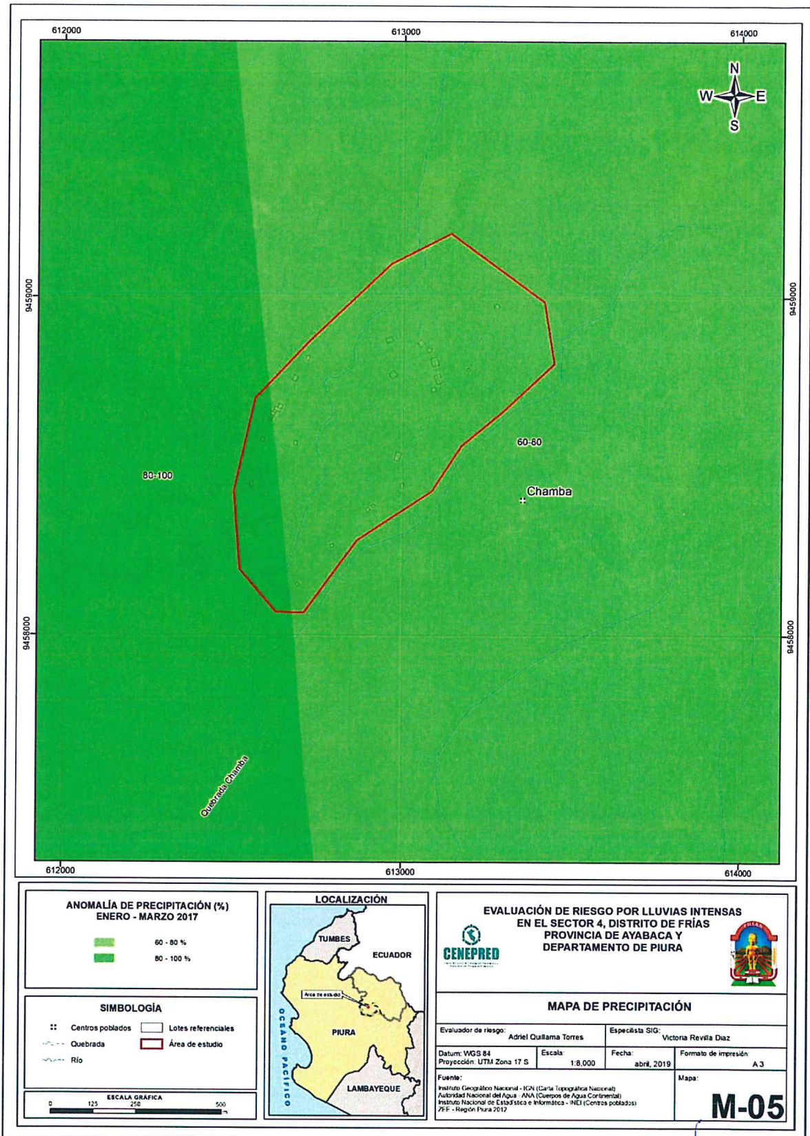
Figura 6. Mapa de Anomalías de Lluvias durante El Niño Costero 2017.
