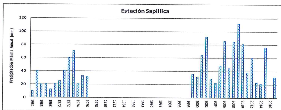
Gráfico 13. Precipitación máxima y Periodo de retorno Estación Sapillica – convencional
