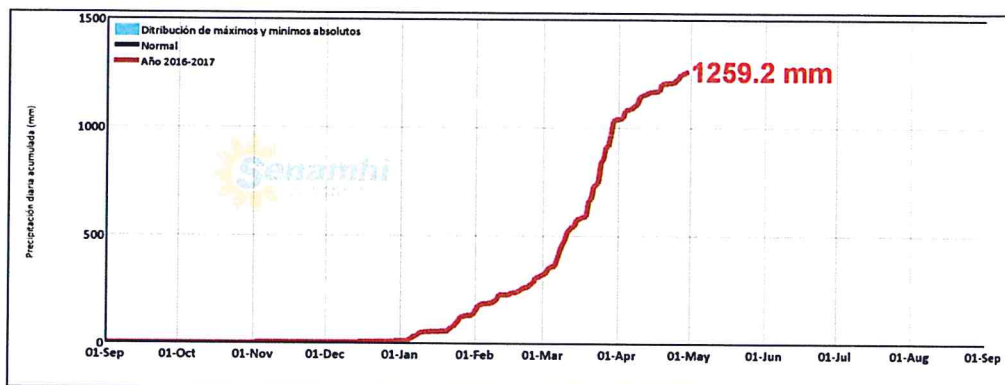
Gráfico 11. Precipitación diaria acumulada en la estación meteorológica Sapillica – automática
