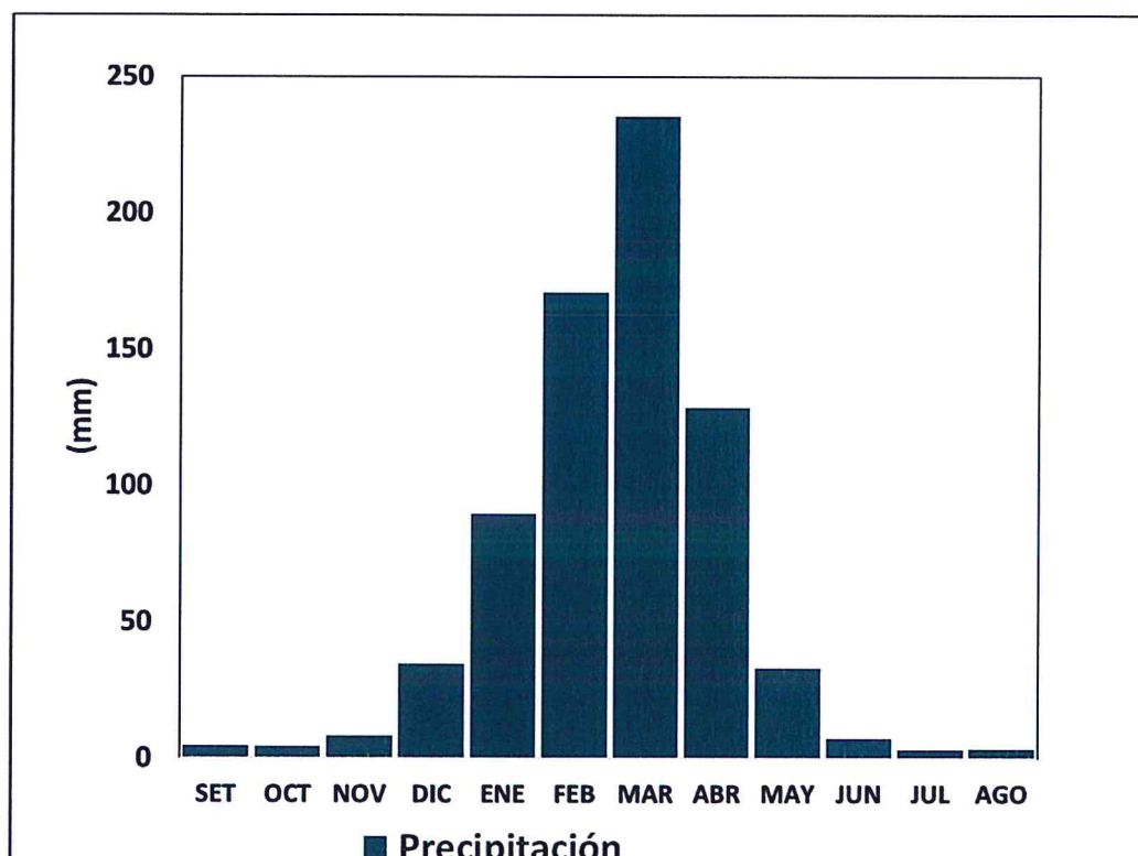
Gráfico 9. Comportamiento temporal de la precipitación promedio en la estación meteorológica Sapillica
