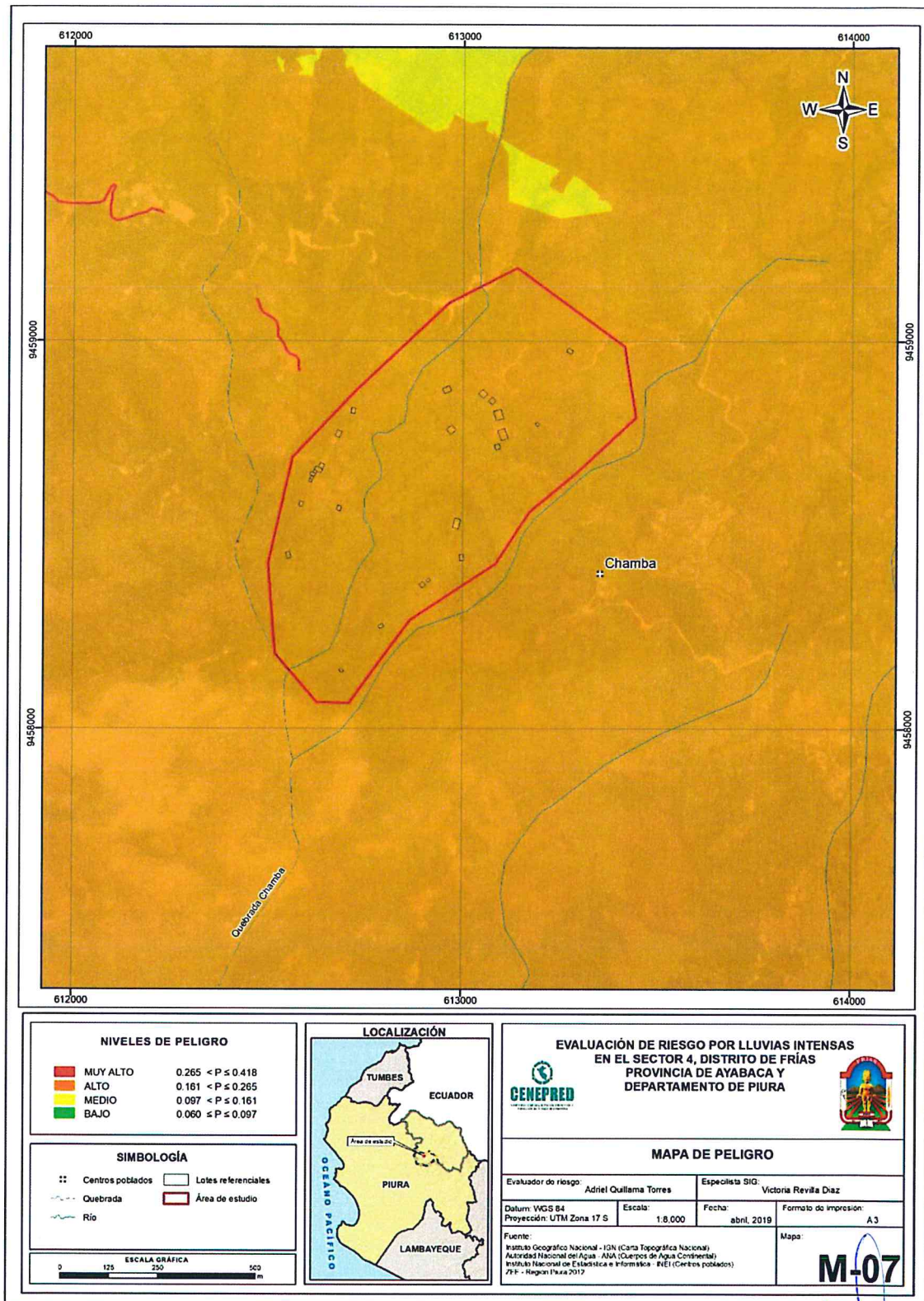
Figura 8. Mapa de Peligro, del Sector 4 del distrito de Frías.
