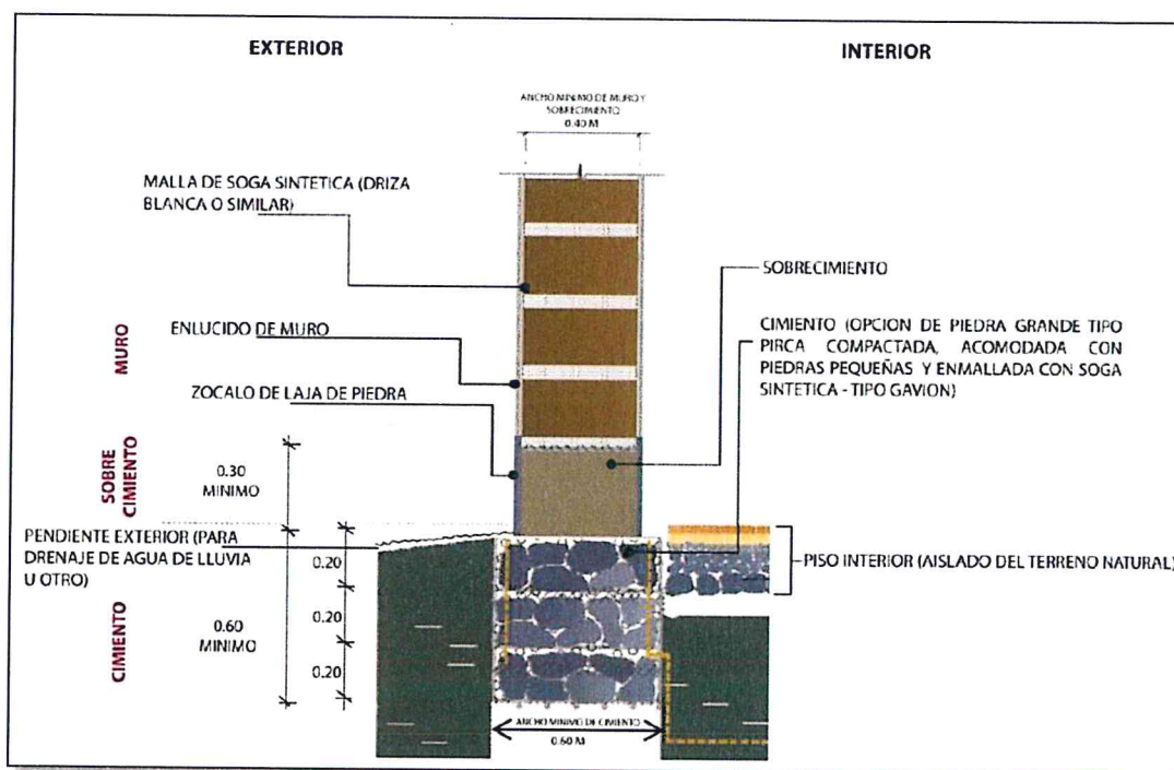
Figura 17. Cimentación en construcciones en Adobe.
