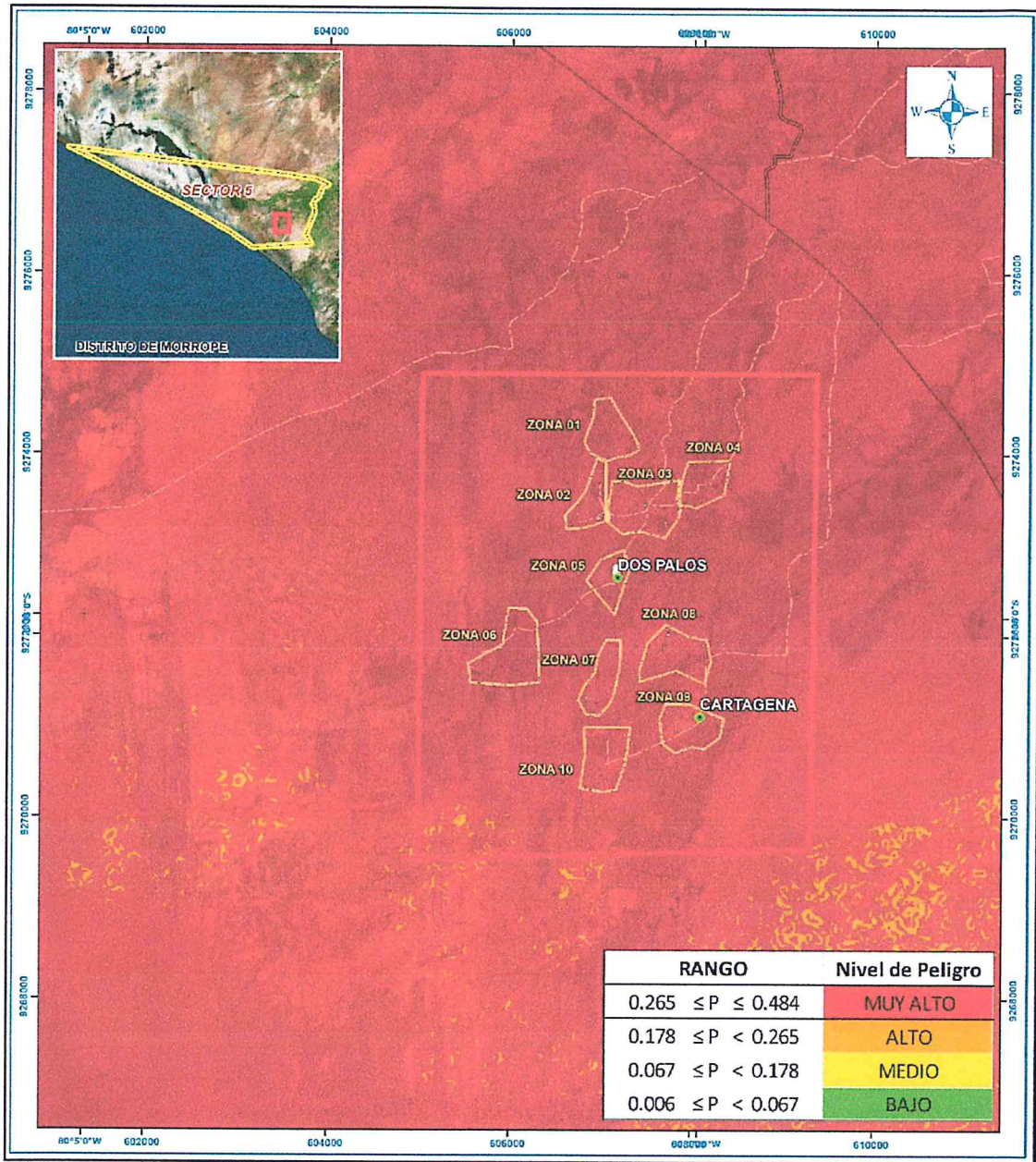
Figura 18. Mapa de Peligro del Sector 5 por Inundación Pluvial
