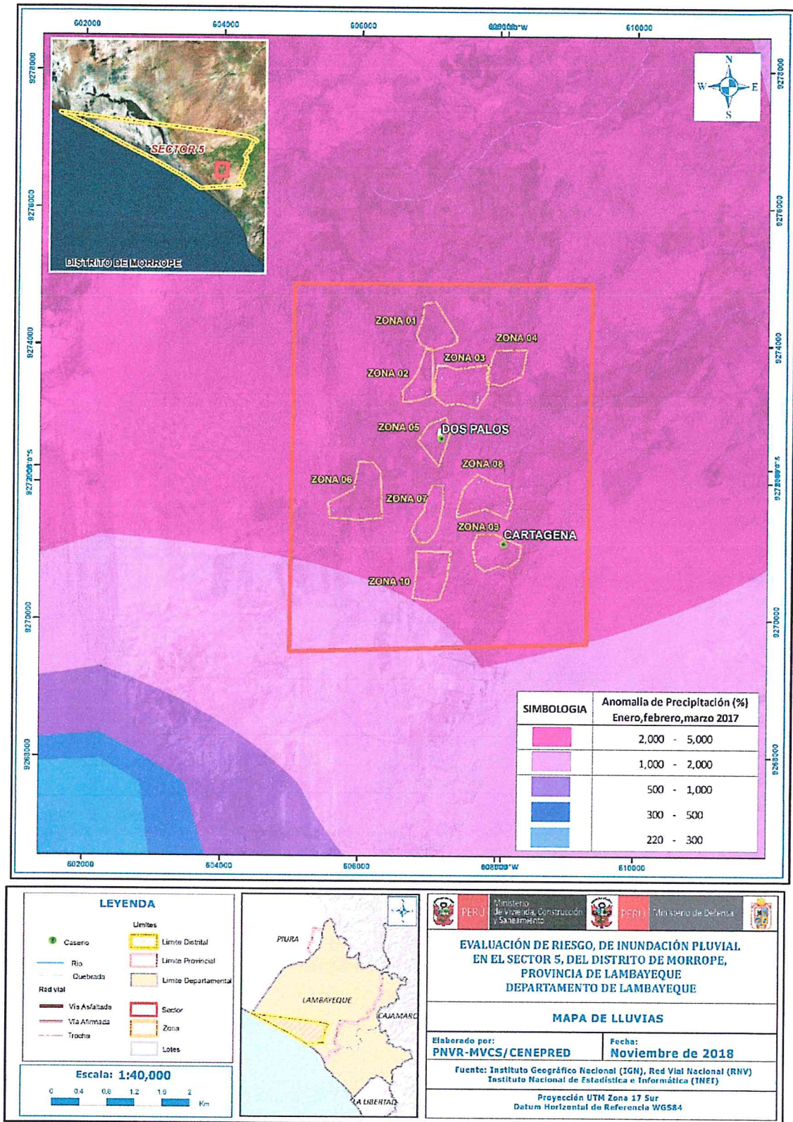
Figura 16. Mapa de Lluvia Anomalías de llluvias durante El Niño Costero 2017 (enero-marzo) para el Sector 5 del Distrito de Mórrope
