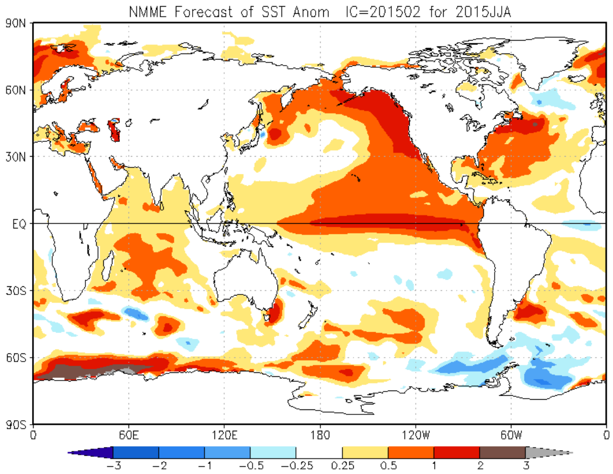
Figura 10. Similar a la Fig.9, pero para el trimestre junio – agosto de 2015.
