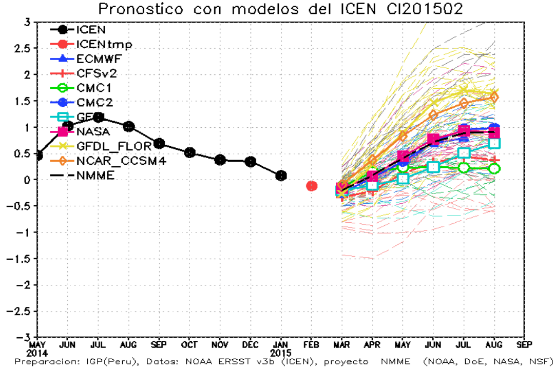
Figura 7. Índice Costero El Niño (ICEN, negro con círculos llenos) y sus valor temporal (ICENtmp, rojo con círculo lleno). Además, pronósticos numéricos del ICEN (media móvil de 3 meses de las anomalías pronosticadas de TSM en Niño 1+2) por diferentes modelos climáticos. Las líneas entrecortadas corresponden a los miembros de los "ensembles". Los pronósticos de los modelos CFSv2, CMC1, CMC2, GFDL, NASA GFDL_FLOR y NCAR_CCISM4 tienen como condición inicial el mes de febrero de 2015. El modelo ECMWF tiene como condición inicial el mes de febrero de 2015. (Fuente: IGP, NOAA, proyecto NMME, ECMWF).
