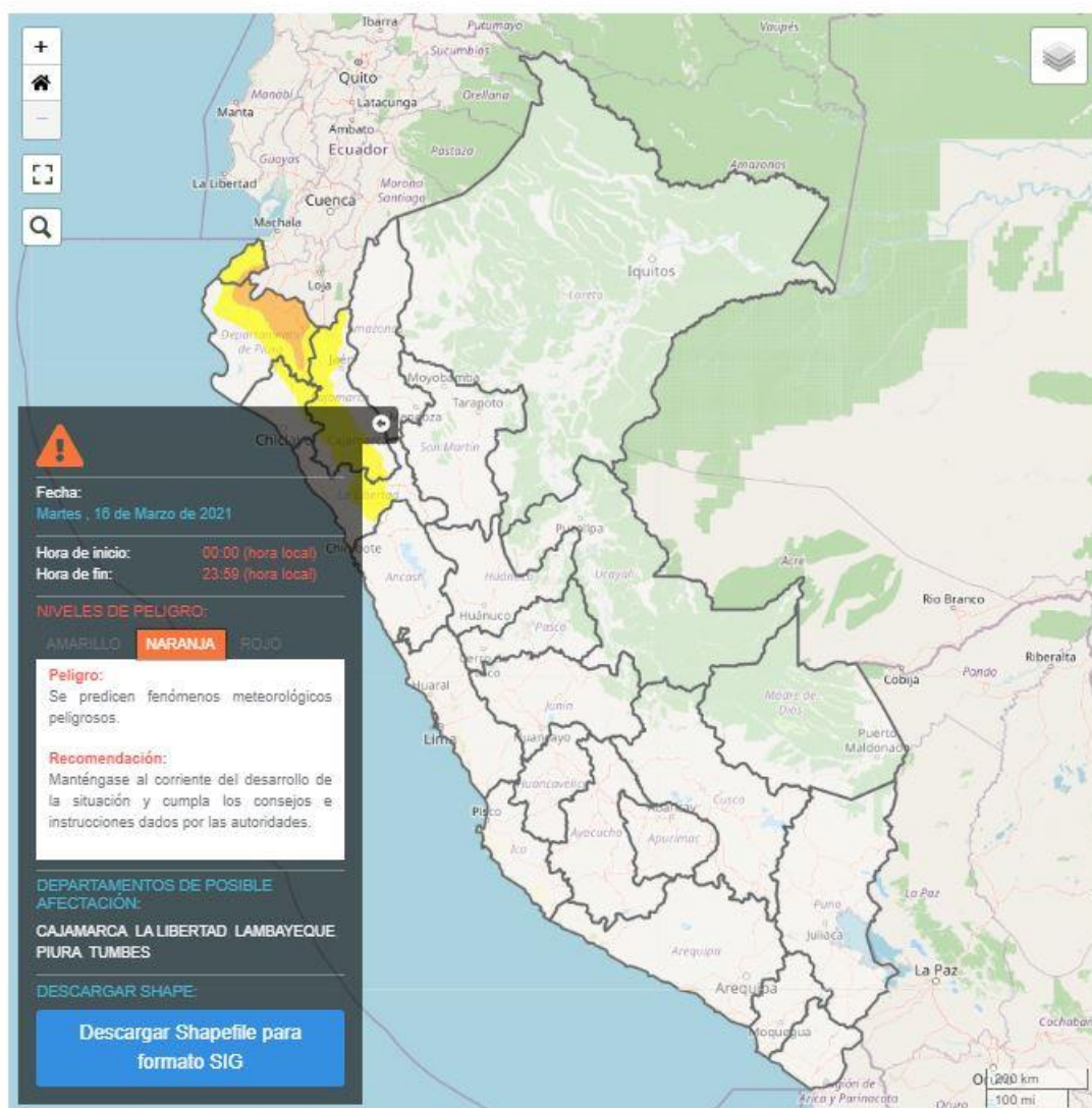
Figura 2. Pronóstico de precipitaciones en la costa y sierra norte del 16 de marzo de 2021
