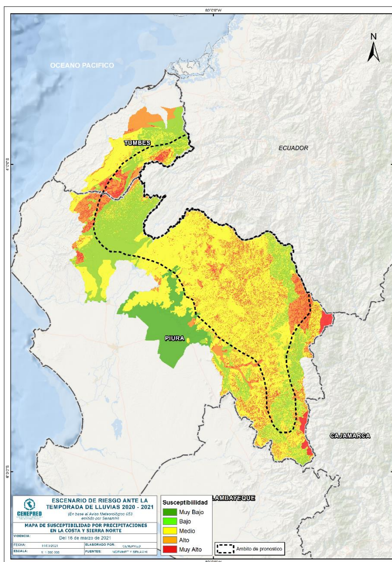
Figura 5. Susceptibilidad a movimientos en masa en la costa y sierra norte
