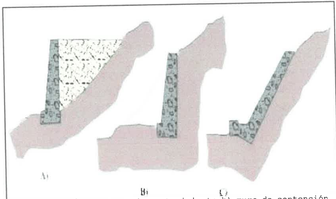
Imagen N° 13: a) muro de sostenimiento b) muro de contención c) muro de revestimiento, fuente: INGEMMET, 2020.
