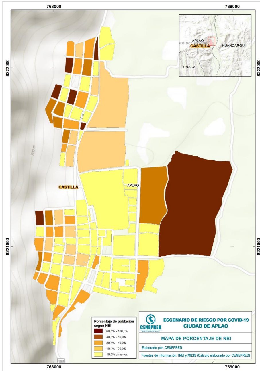
Figura 8. Ciudad de Aplao: Mapa de porcentaje de población según NBI
