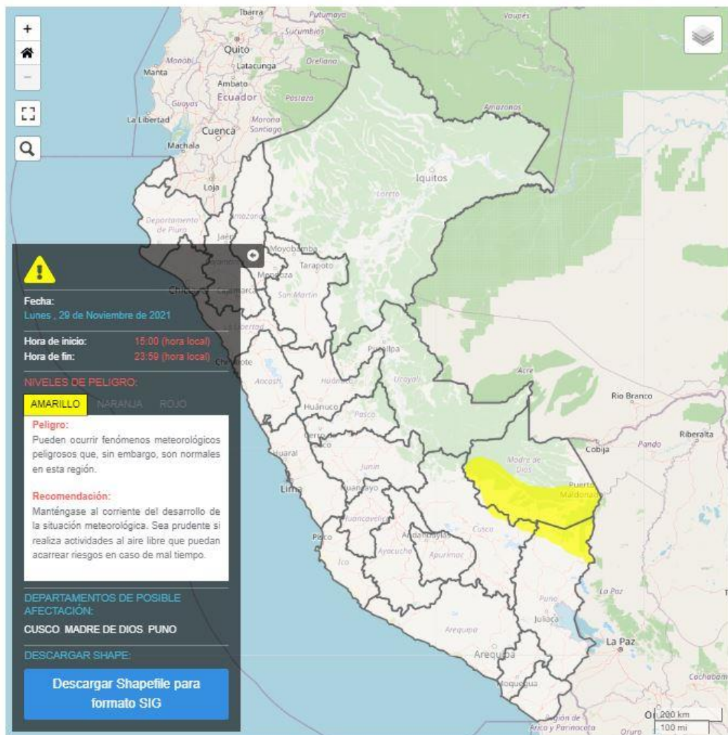
Figura 2. Pronóstico de lluvia en la selva 29 de noviembre de 2021
