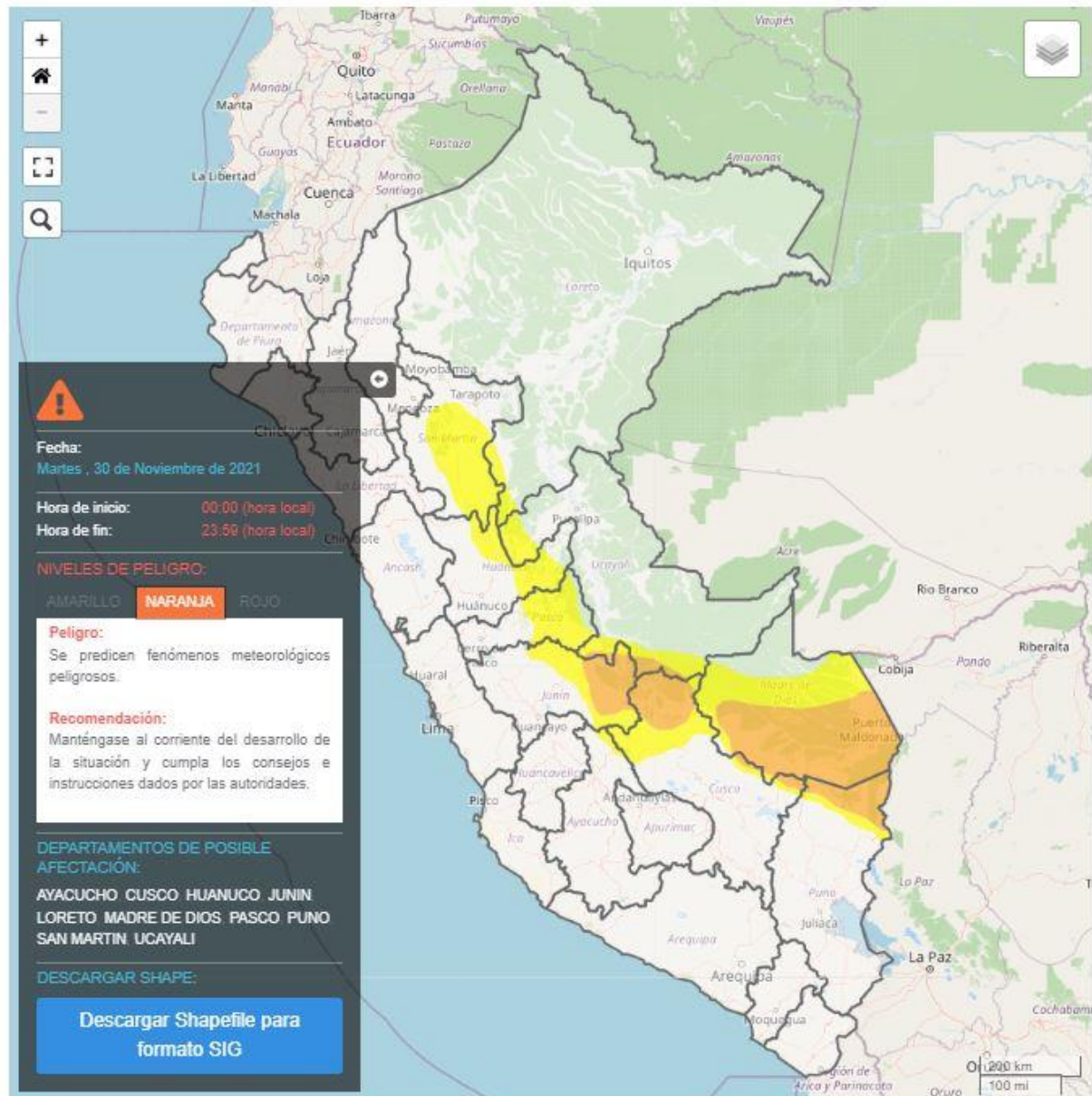
Figura 4. Pronóstico de lluvia en la selva del 30 de noviembre de 2021
