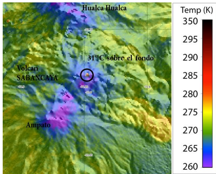
Figura 3.- Imagen ASTER-thermal infrarrojos, nocturno, de la zona de cráter del volcán Sabancaya, tomado el 24/4/2013.
