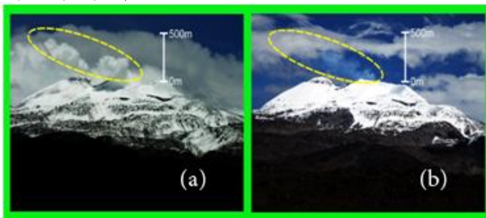
Figura 4.- Emisión de fumarolas en el volcán Sabancaya. (a) Inicialmente solo se observaba de color blanquecino. (b) Después del 14 de marzo ocasionalmente se observa emisiones azulinas.
