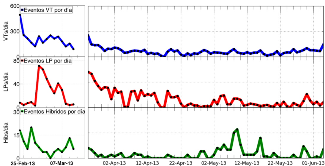
Figura 5.- Evolución temporal de la sismicidad en la zona del volcán Sabancaya. Parte izquierda del grafico: estación sísmica CAJ temporal; parte derecha: estación telemétrica SAB permanente. Se observa una amplia predominancia de los eventos VT o de fractura. En general, los sismos asociados al paso de fluidos se presentan escasos.
