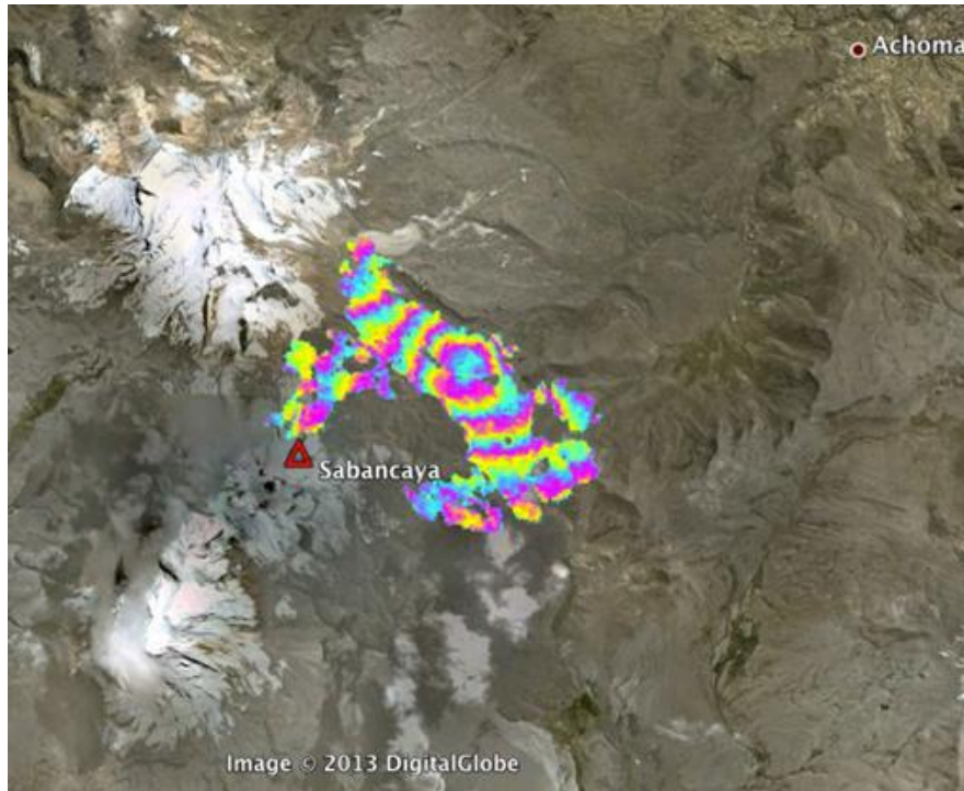
Figura 2.- Interferograma InSAR (14/01/12-29/03/13) de la zona del volcán Sabancaya. La zona de deformación central se correlaciona con la zona de epicentros sísmicos de la figura 1.
