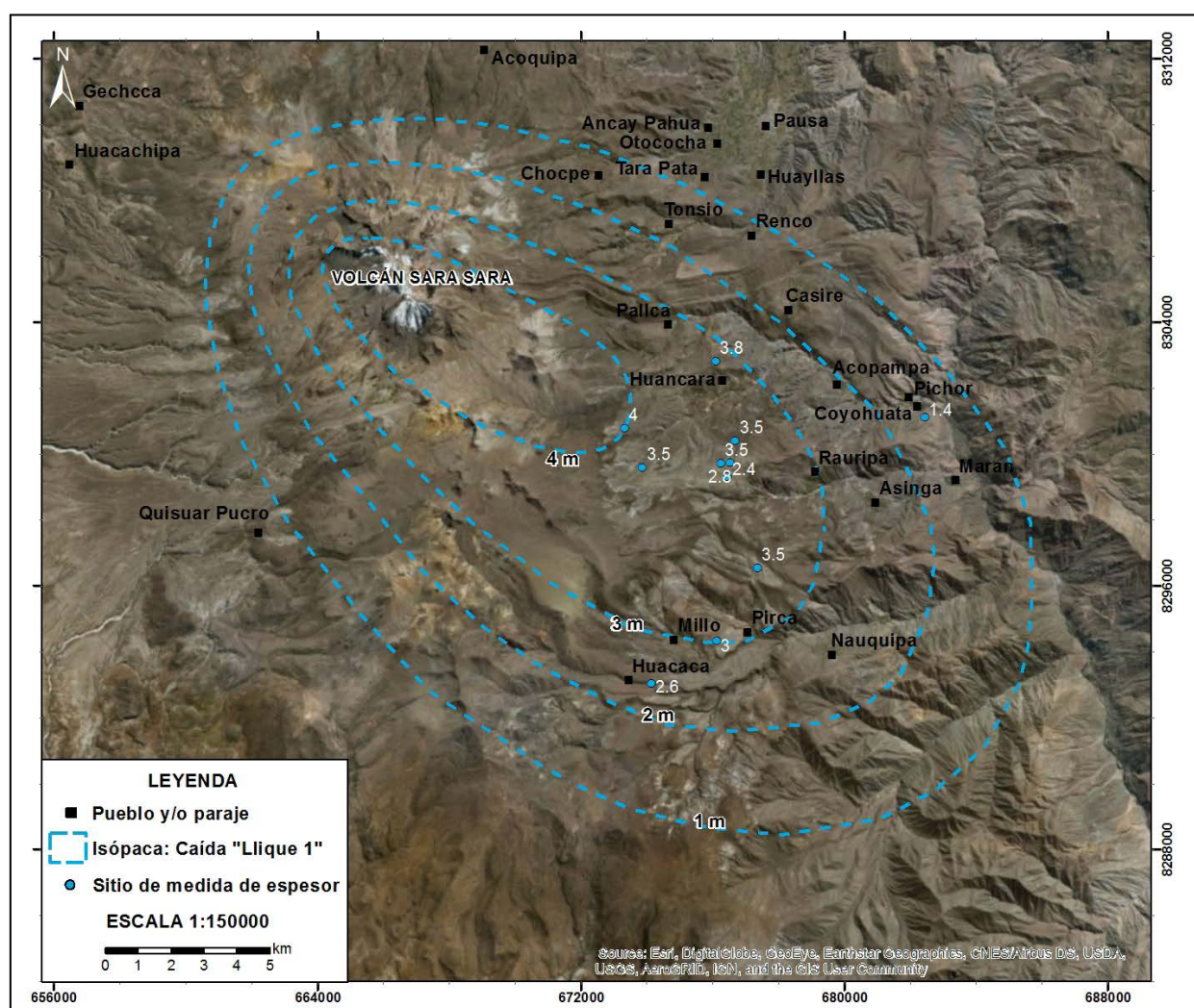
Figura 3.24 Mapa de isópaca del depósito de caída de lapilli de pómez "Llique I"
