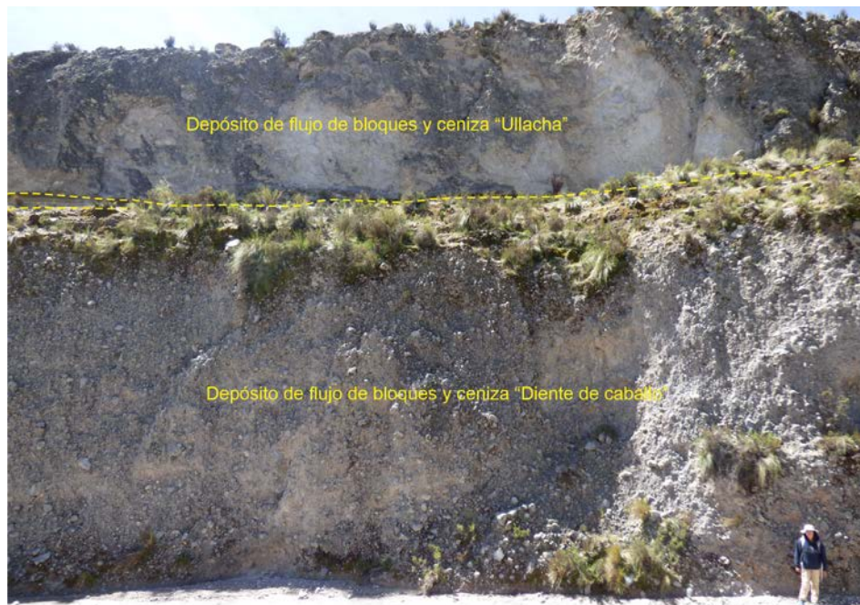
Figura 3.37 Depósitos de flujo de bloques y ceniza, a 13.5 km al oeste del volcán Sara Sara, en la confluencia del río Salla Salla y quebrada Ullacha Grande
