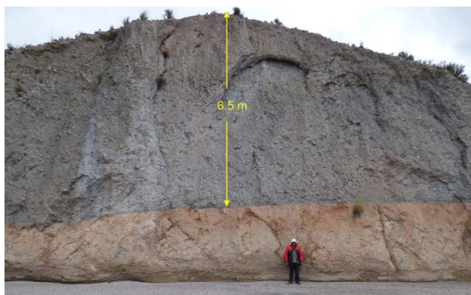
Figura 3.32 Depósito de flujo de bloques y ceniza “Diente de caballo” que aflora a 15 km al oeste del volcán Sara Sara, donde mide hasta 6.5 m de espesor
