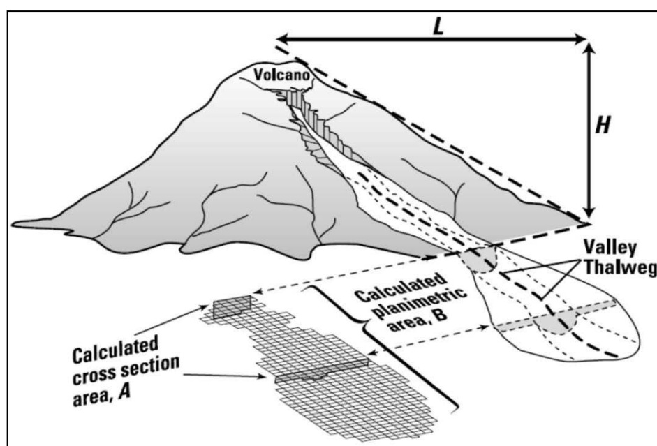
Figura 6.2 Relaciones entre la distancia ( L ) y la altura ( H ) por donde recorrerán los lahares, así como las áreas en sección transversal ( A ) y planimétrica ( B ), inundadas por un evento lahárico (Schilling, 1998)
