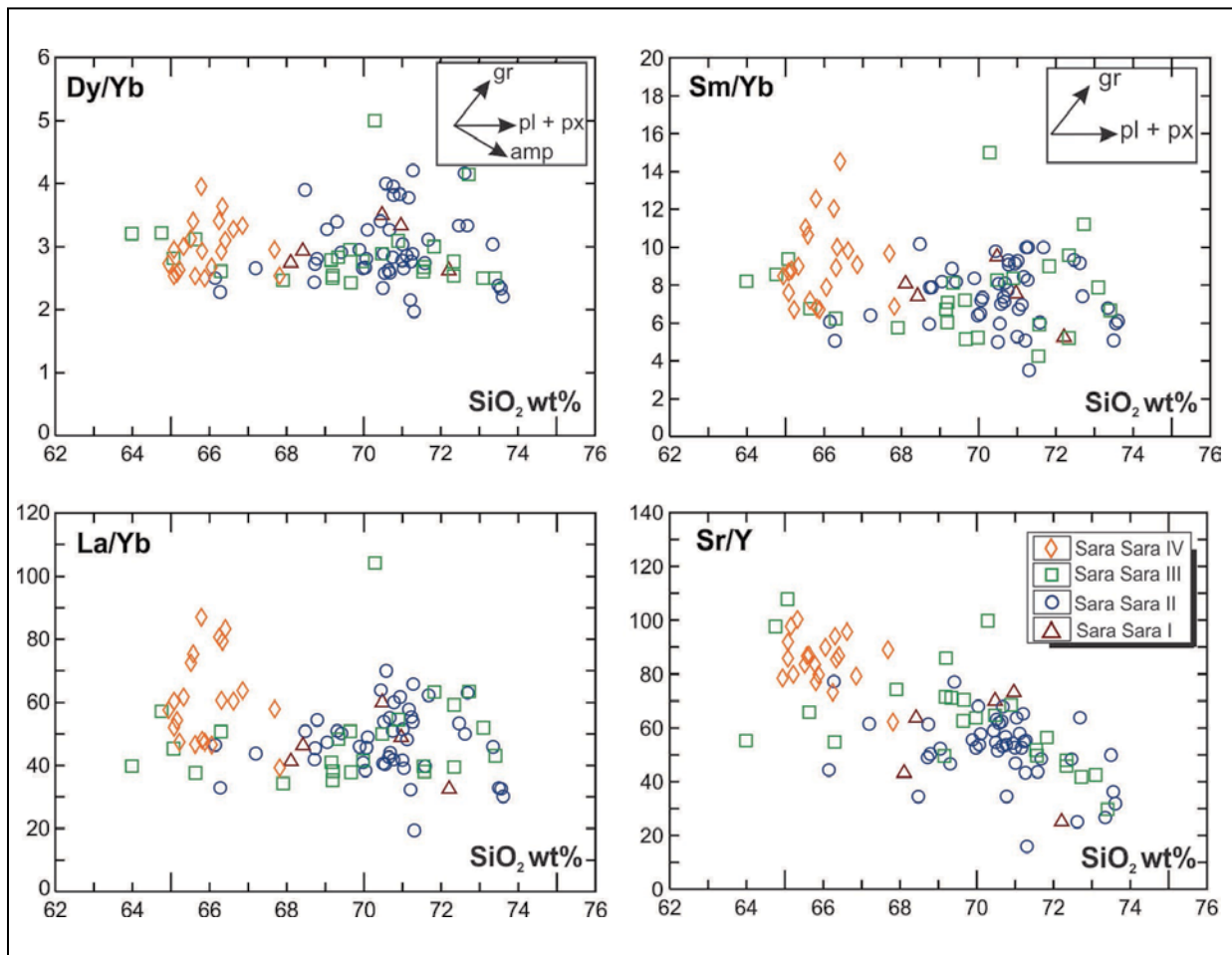
Figura 5.8 Diagramas de ratios Dy/Yb, Sm/Yb, La/Yb y Sr/Y vs. \text{SiO}_2 de rocas del volcán Sara Sara, (gr) granate, (pl) plagioclase, (px) piroxenos, (amp) anfíbol
