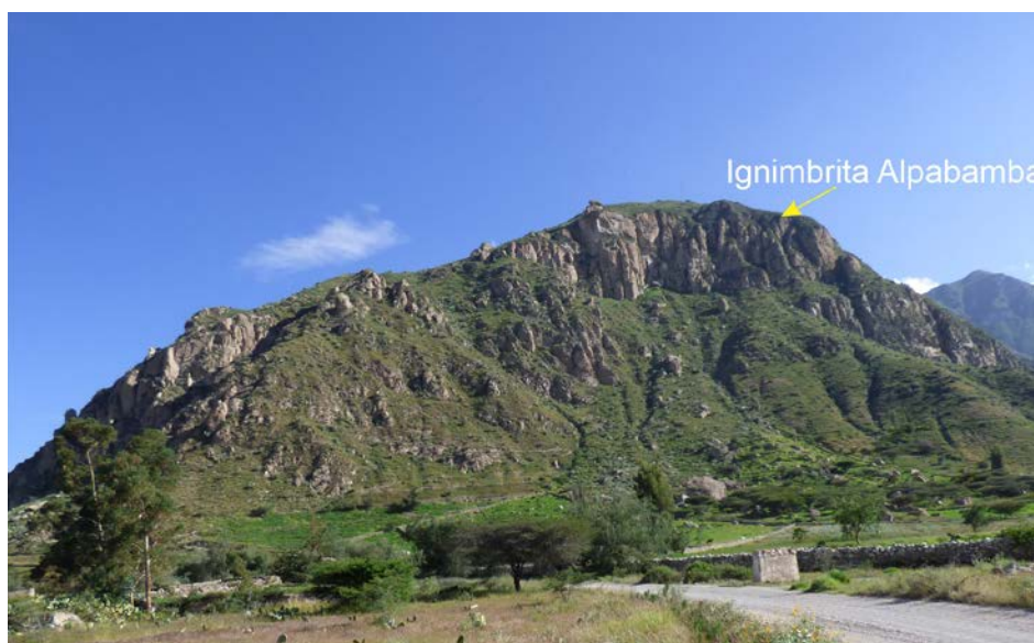
Figura 3.3 Ignimbritas riolíticas pertenecientes a la Formación Alpabamba, en inmediaciones de la localidad de Santa Ana (Pausa)
