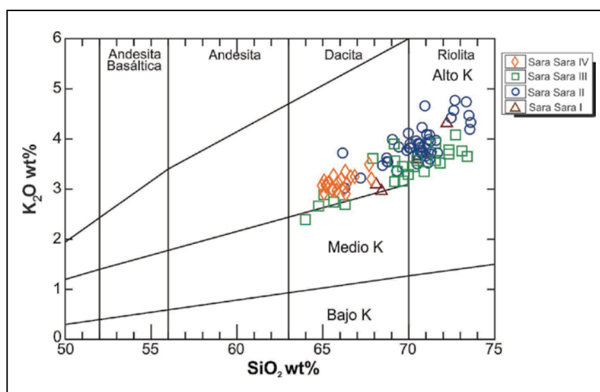
Figura 5.3 Diagrama K_2O vs. SiO_2 de Peccerillo & Taylor, de rocas del volcán Sara Sara, que muestra tendencia moderada a fuertemente potásica.
