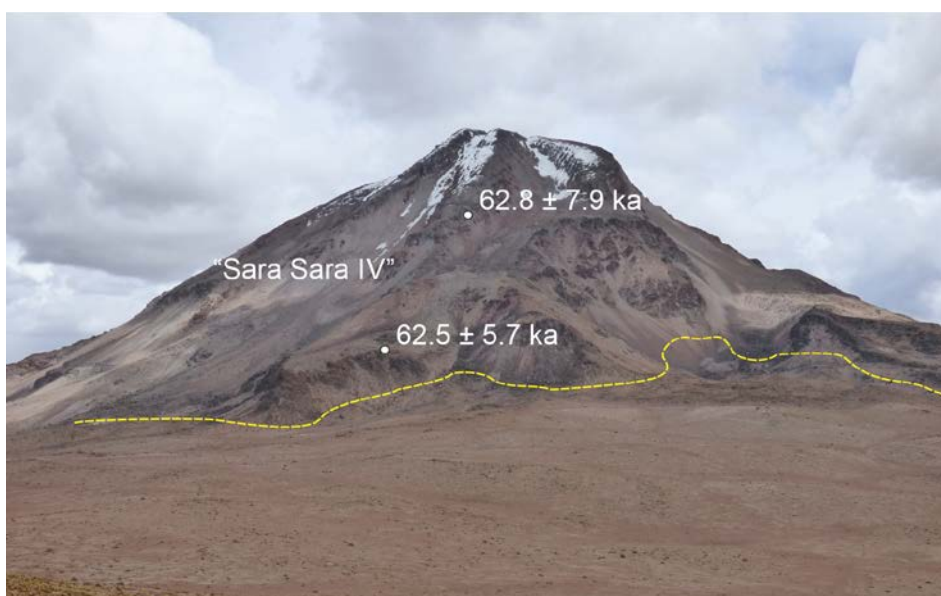
Figura 3.39 Vista del flanco sureste del volcán Sara Sara, donde se aprecia flujos de lavas asignados a la etapa “Sara Sara IV”
