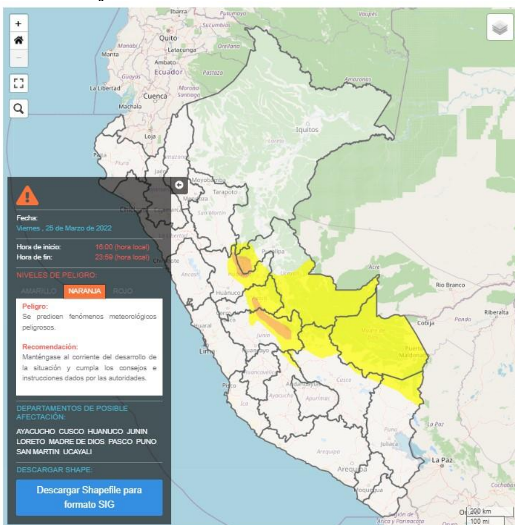
Figura 2. Pronóstico de lluvia en la selva del 25 de marzo del 2022
