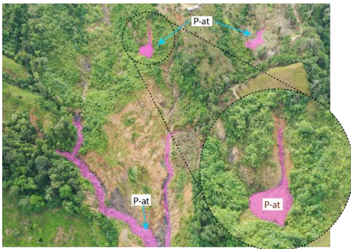
Figura 10. Subunidades geomorfológicas conformadas por Vertiente aluvio-torrencial (P-at), ubicado en el cuerpo del deslizamiento activo.
