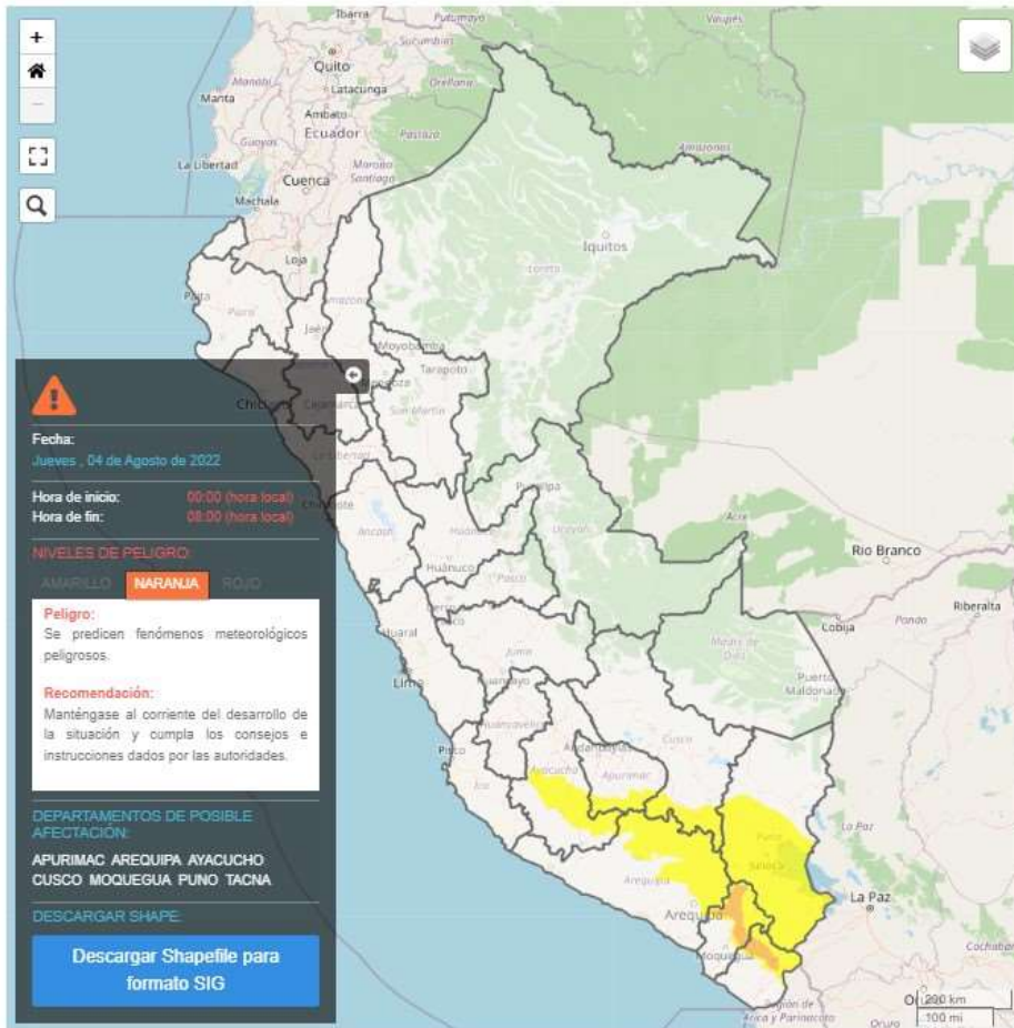
Figura 1. pronóstico de descenso de temperatura nocturna en la sierra centro y sur del 04 de agosto 2022.
