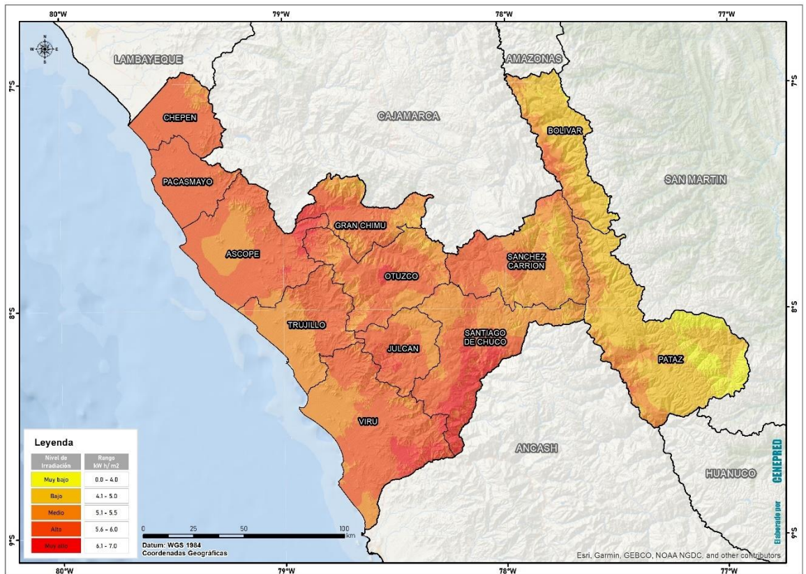
Figura 13. Mapa de irradiación de energía solar incidente
