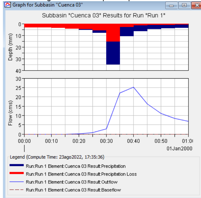
Gráfico N° 17. Hidrograma del caudal para un periodo de retorno de 25 años.
