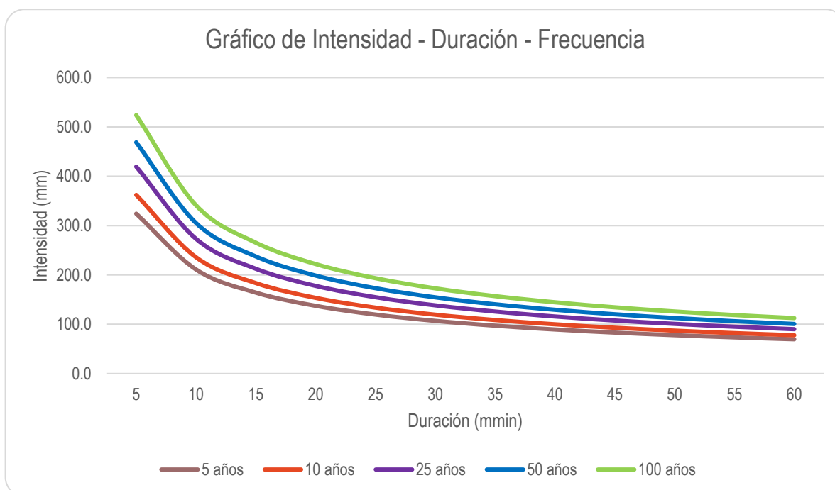
Gráfico N° 08. Curva intensidad – duración – frecuencia.
