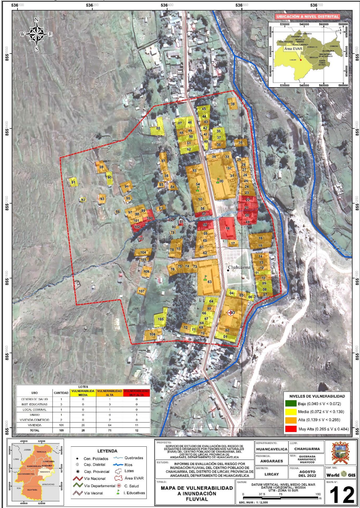
Figura N° 35: Mapa de vulnerabilidad a inundación fluvial, del área en evaluación
