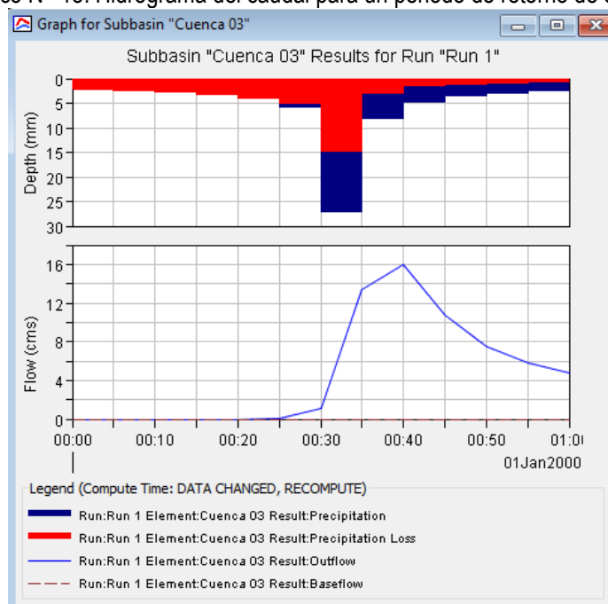
Gráfico N° 15. Hidrograma del caudal para un periodo de retorno de 5 años.
