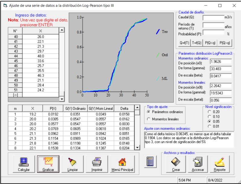
Gráfico N° 05. Cálculo de distribución Log-Pearson tipo III
