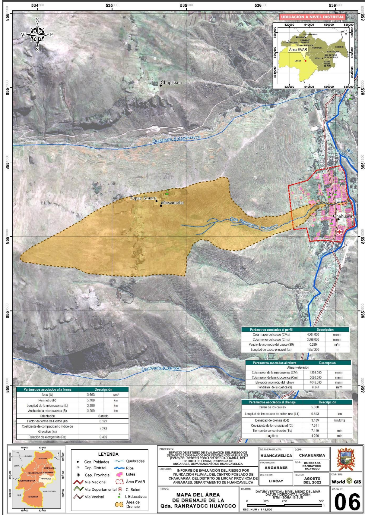
Figura N° 027. Mapa de la unidad hidrográfica Ranrayocc Huaycco (área de drenaje)
