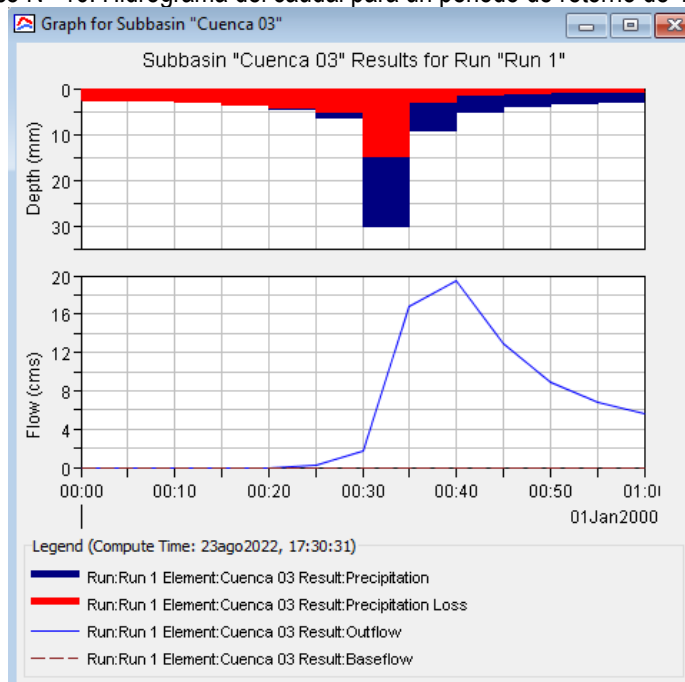
Gráfico N° 16. Hidrograma del caudal para un periodo de retorno de 10 años.
