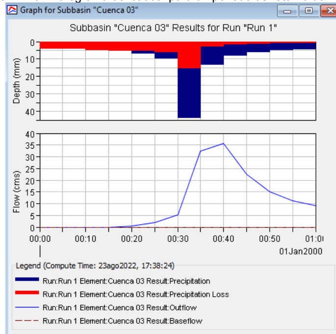
Gráfico N° 19. Hidrograma del caudal para un periodo de retorno de 100 años.
