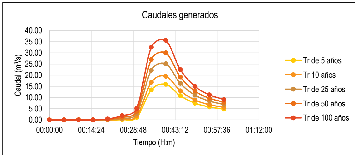
Gráfico N° 011. Comparación de los caudales para diferentes periodos de retorno.
