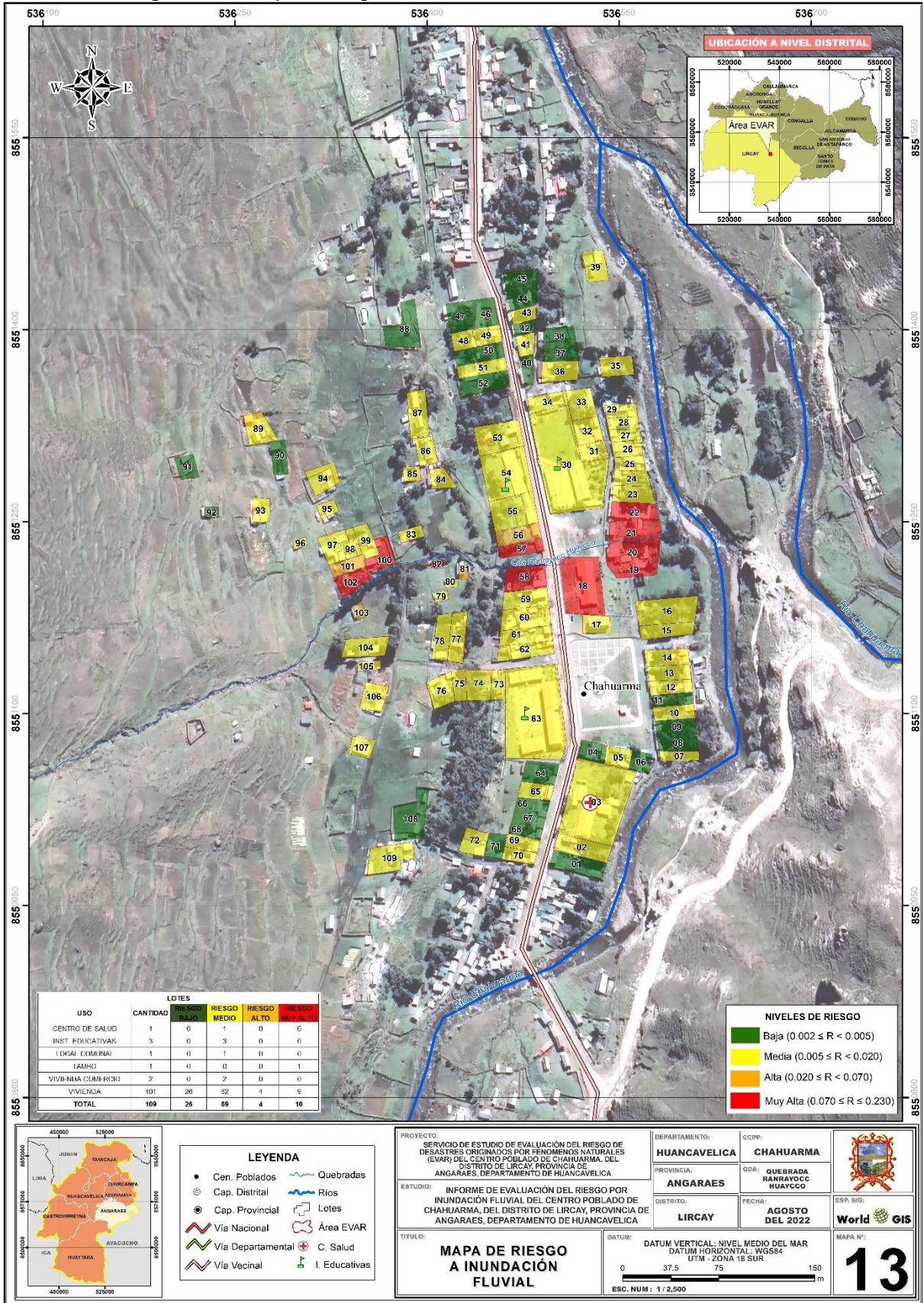
Figura N° 36: Mapa del riesgo a inundación fluvial, del área en evaluación
