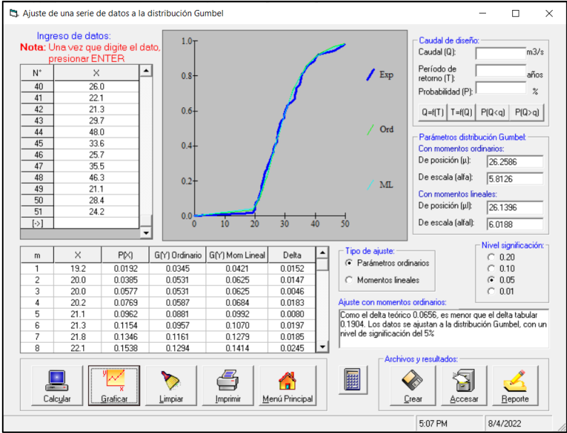
Gráfico N° 06. Cálculo de distribución de Gumbel.
