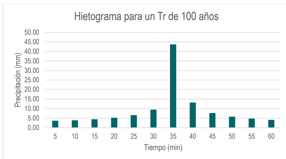
Gráfico N° 13. Hietograma para un tiempo de retorno de 100 años para la unidad hidrográfica Ranrayocc Huaycco.
