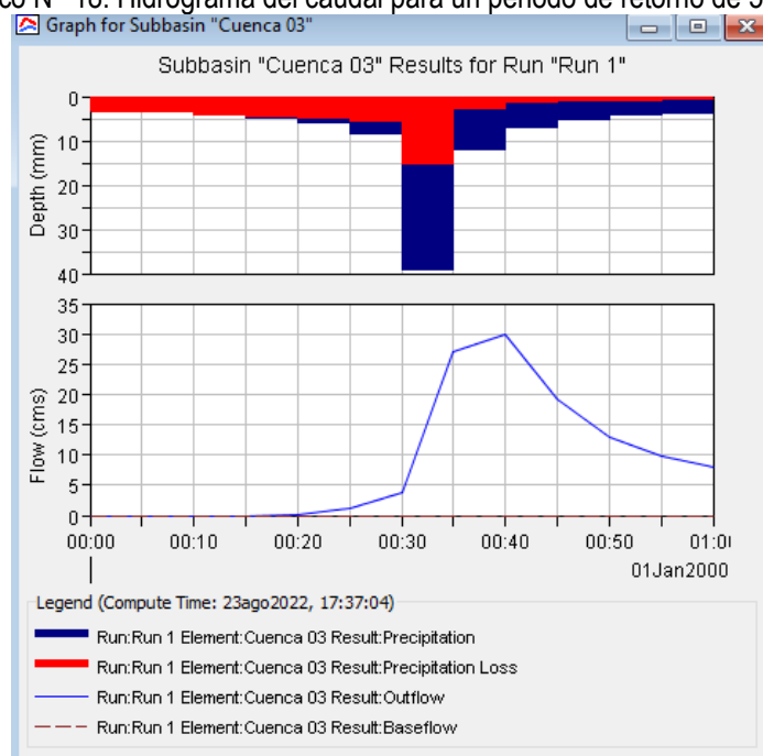
Gráfico N° 18. Hidrograma del caudal para un periodo de retorno de 50 años.
