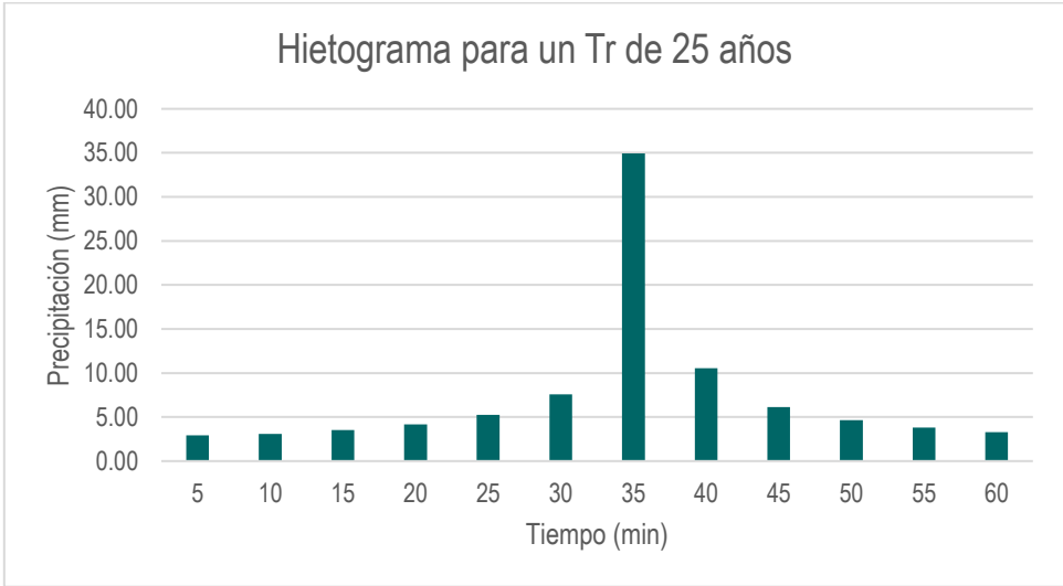
Gráfico N° 11. Hietograma para un tiempo de retorno de 25 años para la unidad hidrográfica Ranrayocc Huaycco.
