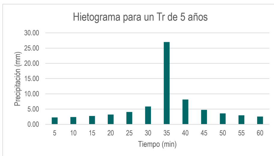
Gráfico N° 09. Hietograma para un tiempo de retorno de 5 años para la unidad hidrográfica Ranrayocc Huaycco.
