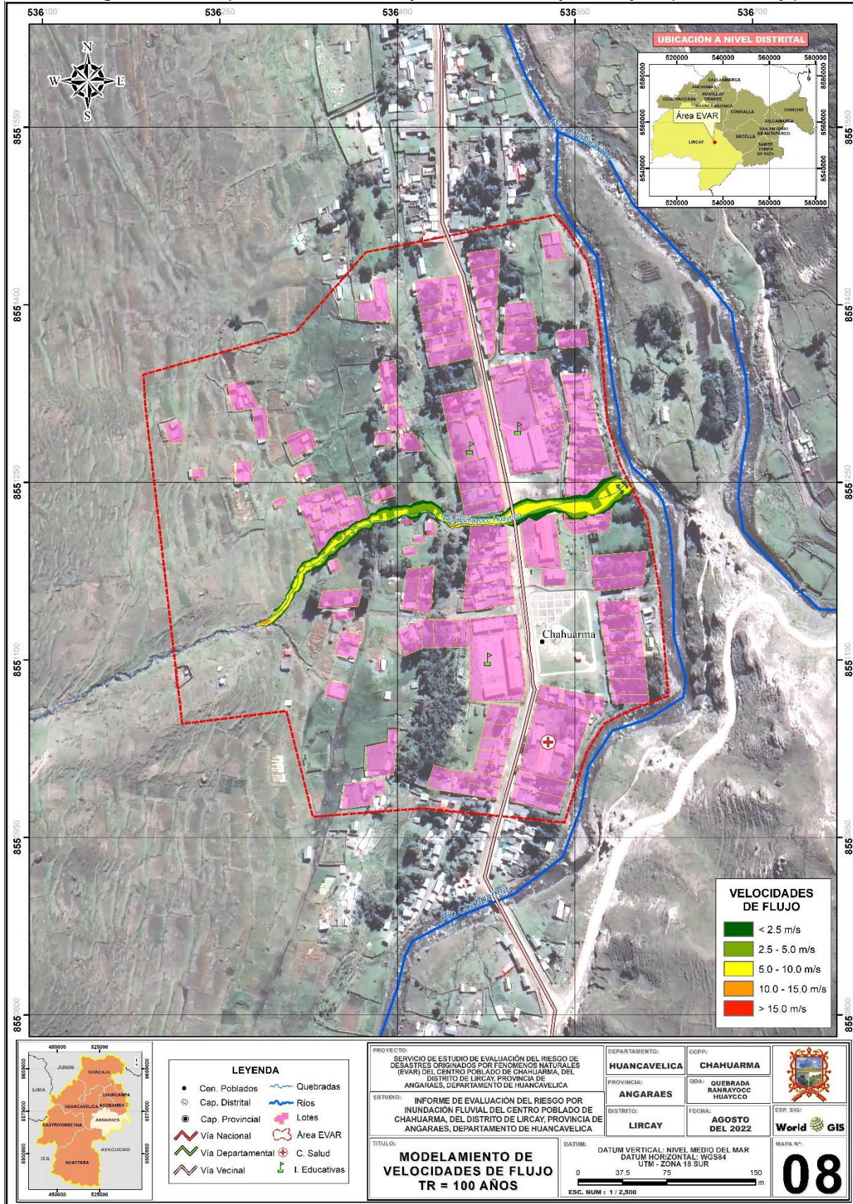
Figura N° 030. Mapa de velocidades de flujo de la Qda. Ranrayocc Huaycco (área de drenaje)
