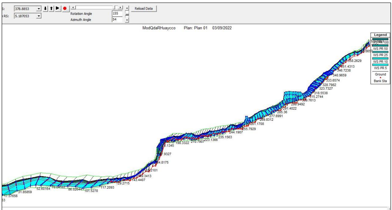
Gráfico N° 012. Modelación hidráulica – vista de secciones transversales
