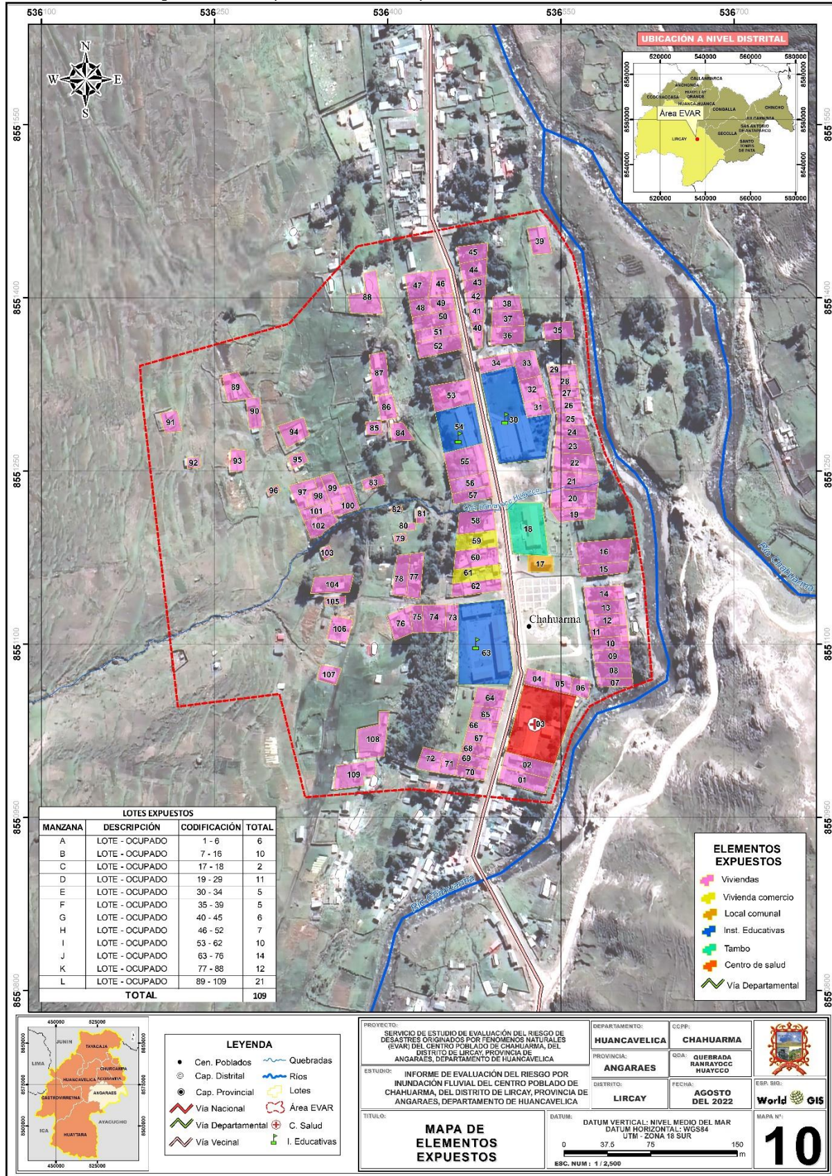
Figura N° 33: Mapa de elementos expuestos del área en evaluación
