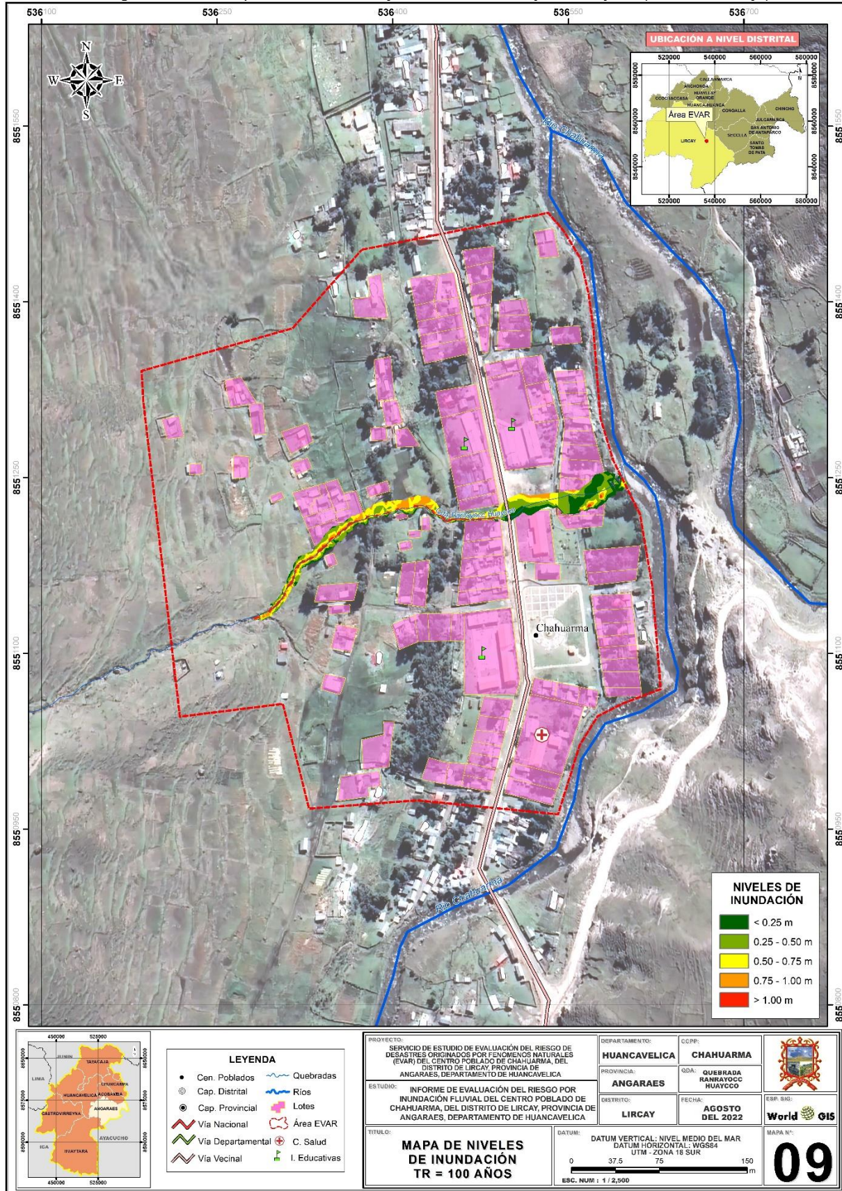
Figura N° 031. Mapa de niveles de flujo de la Qda. Ranrayocc Huaycco (área de drenaje)
