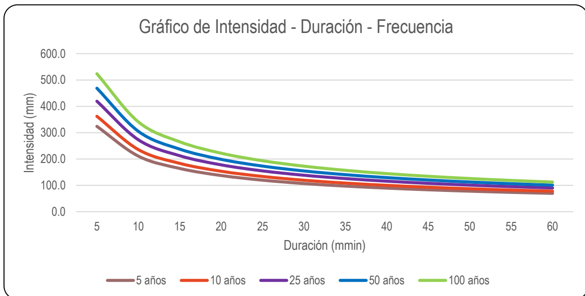
Gráfico N° 010. Curva intensidad – duración – frecuencia.
