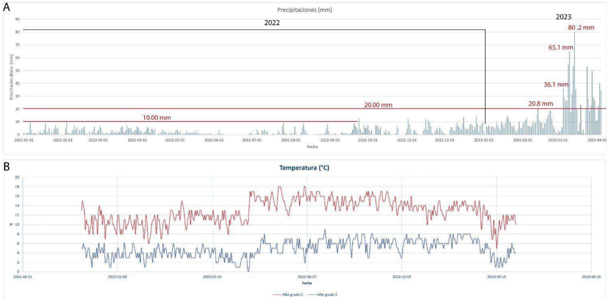
Figura 6. A) precipitación en el caserío Lactash y B) temperaturas en el caserío Lactash (periodo 2022-2023). Fuente: análisis espacial de datos meteorológicos AWERE.
