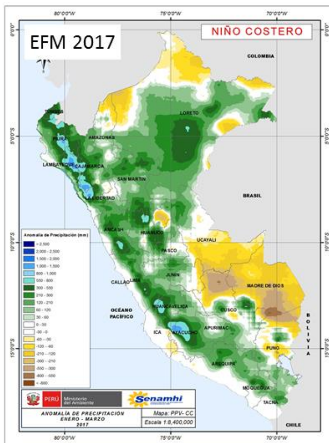
Figura 3. Anomalías de precipitación durante El Niño Costero 2017
