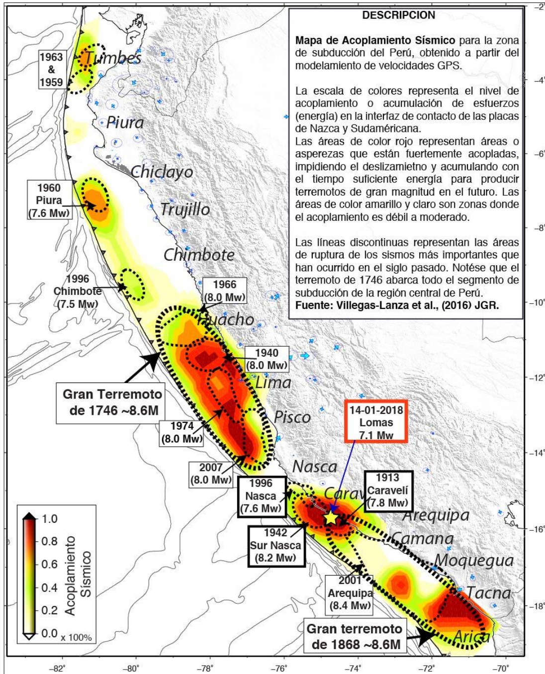
Figura N° 14. Distribución espacial de zonas de acoplamiento sísmico máximo (asperezas) en el borde occidental del Perú.
