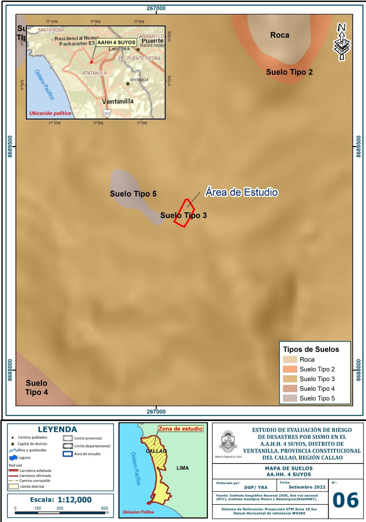
Figura N° 12. Mapa de Tipo de suelo del área de estudio.
