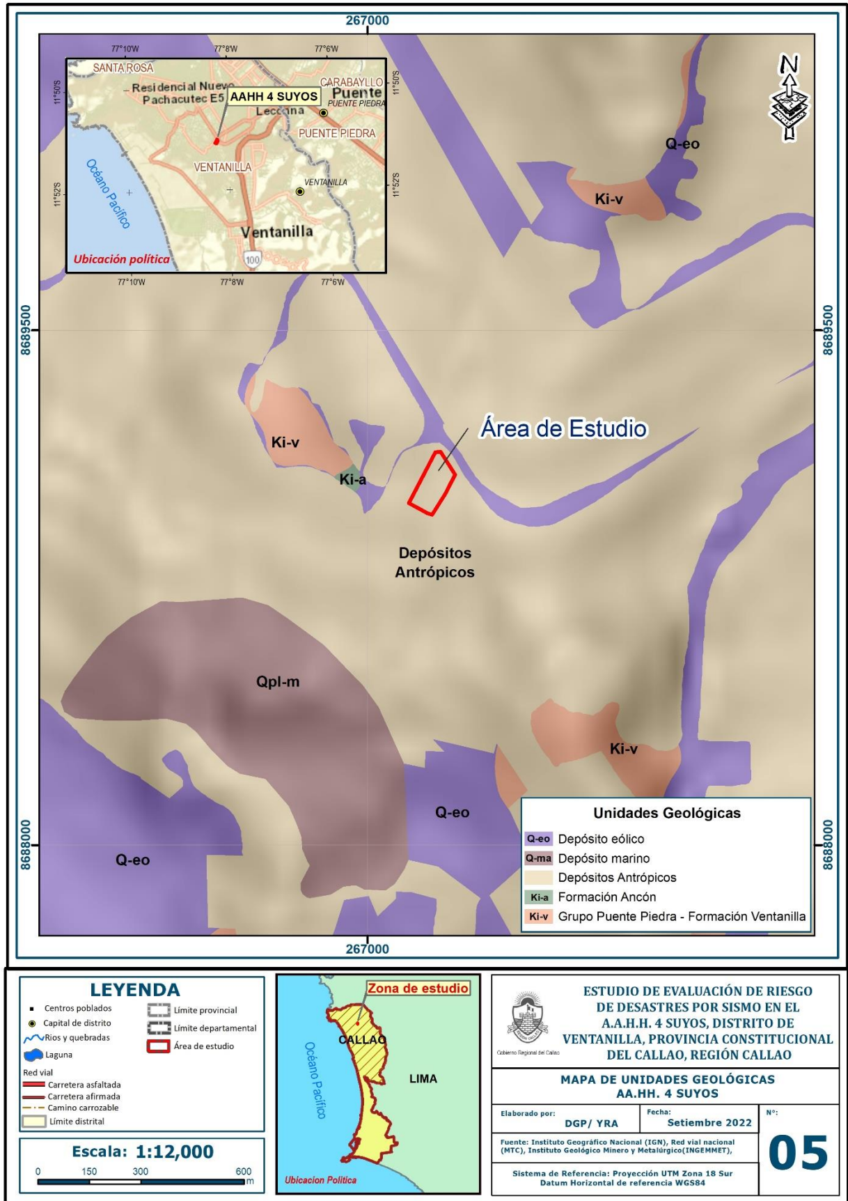
Figura N° 11. Mapa geológico del área de estudio.
