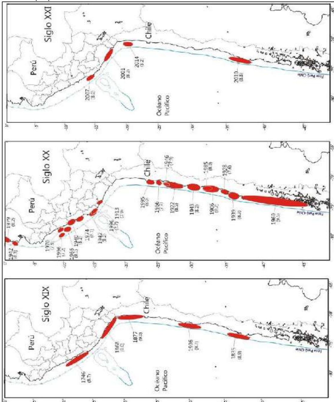
Figura N° 07. Borde occidental de Perú y Chile, y distribución de áreas de ruptura y lagunas sísmicas durante los siglos XIX, XX y XXI. La magnitud de los sismos está expresada en la escala de magnitud momento (Mw).
