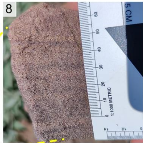
Figura 7 y 8. En el terreno evaluado se observa areniscas de grano fino a grueso de color rojizo, moderadamente meteorizada y muy fracturada. Coordenadas: UTM WGS-84, 17S: E: 775981; N: 9386035.
