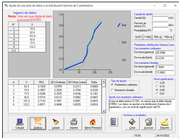
Gráfico N° 07. Cálculo de distribución Gamma de 2 parámetros
