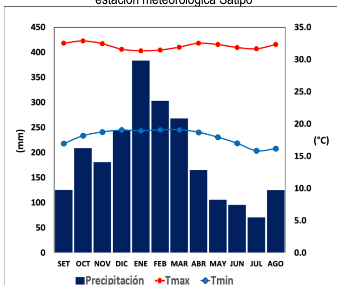
Gráfico N° 06. Comportamiento temporal de la temperatura del aire y precipitación promedio en la estación meteorológica Satipo
