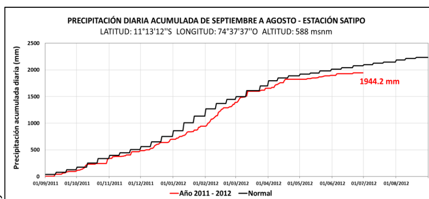
Figura N° 13. Precipitación diaria acumulada en la estación meteorológica Satipo
