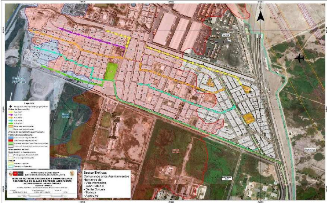
Figura N° 18. Ruta de evacuación propuesta – SECTOR TIWINZA.
