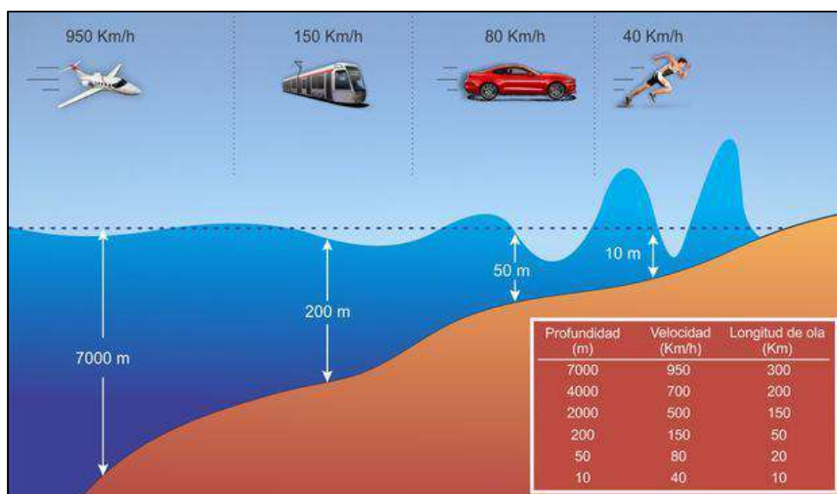
Figura N° 12. Relación entre profundidad, velocidad y longitud de onda de un tsunami.
