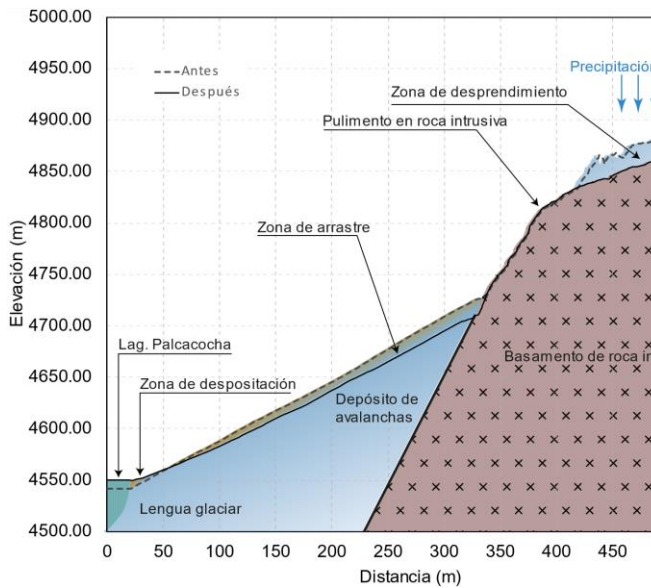
Figura 3. Perfil longitudinal del área de avalancha
