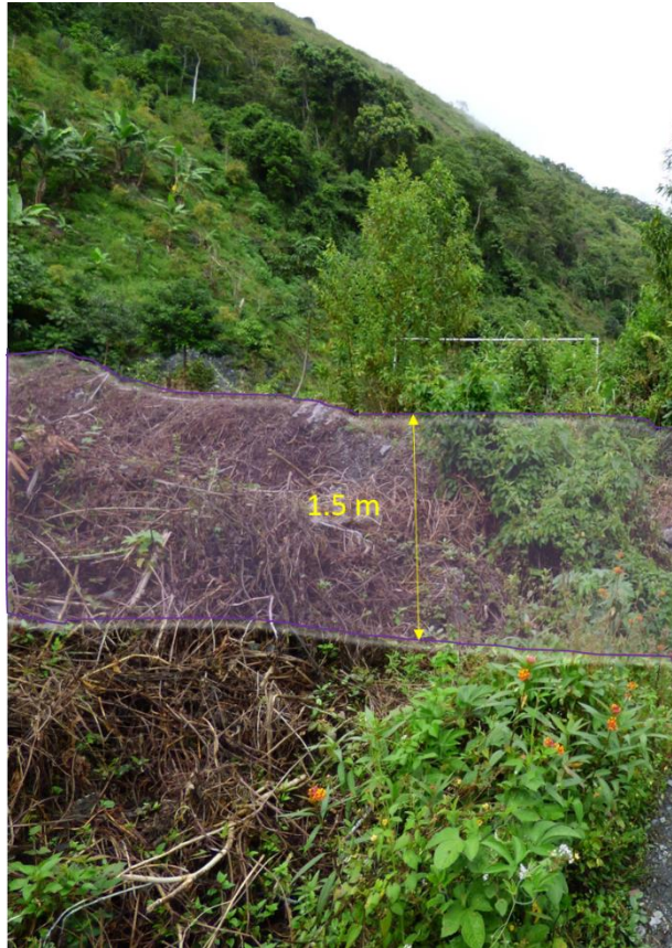
Figura 6. En la imagen se observa el depósito que alcanza 1.5 m de altura aproximada, producto del flujo de detritos ocurrido el año 2017. Los pobladores explanaron la superficie para erigir una cancha de fútbol.
