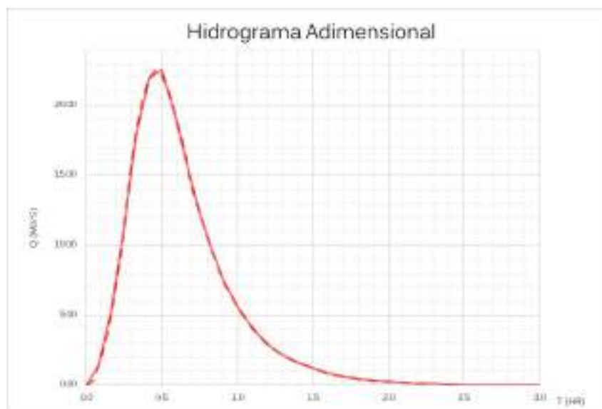
Gráfico 14. Hidrograma adimensional
