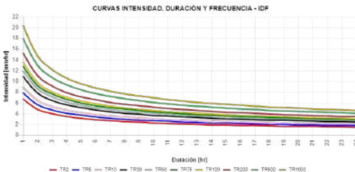
Gráfico 11. Curvas Intensidad – Duración – Frecuencia - IDF ESCENARIO CAMBIO CLIMATICO RCP 8.5
