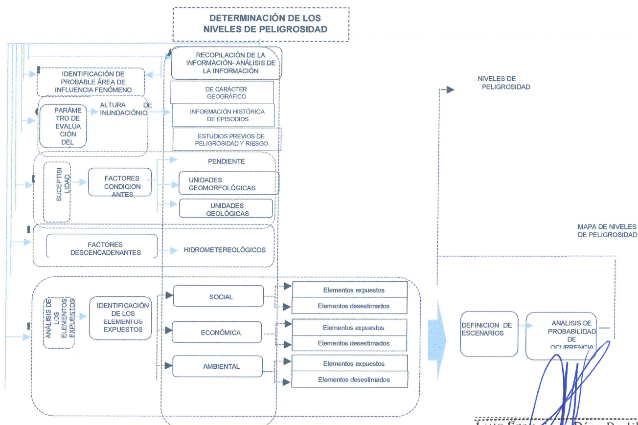
Gráfico 2: Metodología general para determinar el nivel de peligrosidad
