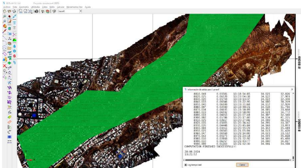
Ilustración 34 - Simulación Iber en la Quebrada San Lázaro Sector Mateo Pumacahua para periodo de retorno de 100 años
