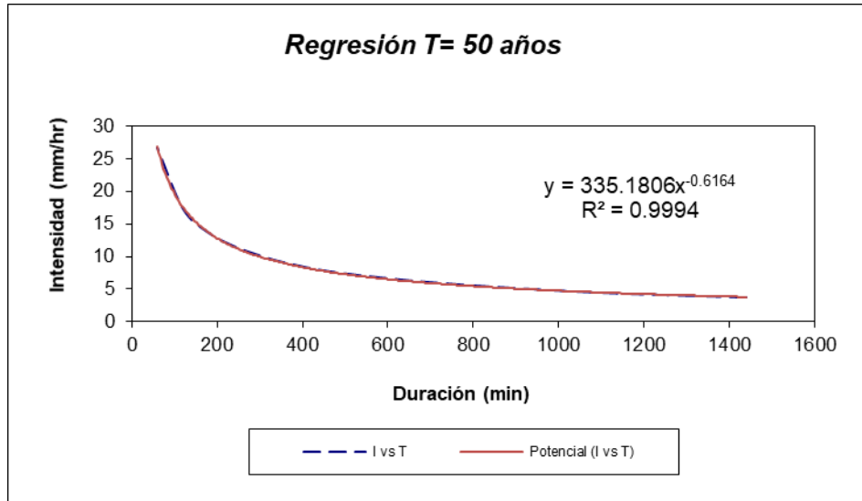
Ilustración 6 - Regresiones IDF para TR: 50 años.
