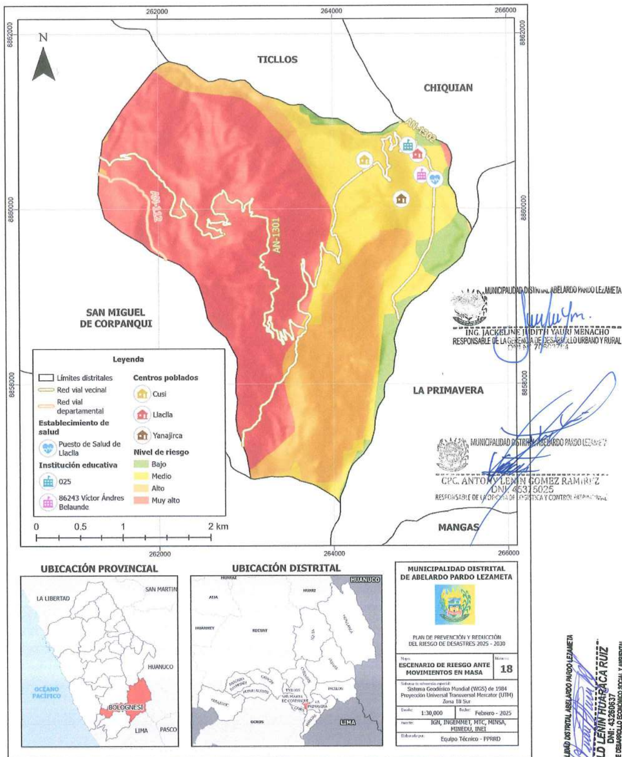
Mapa 18 Escenario de riesgo ante movimientos en masa
