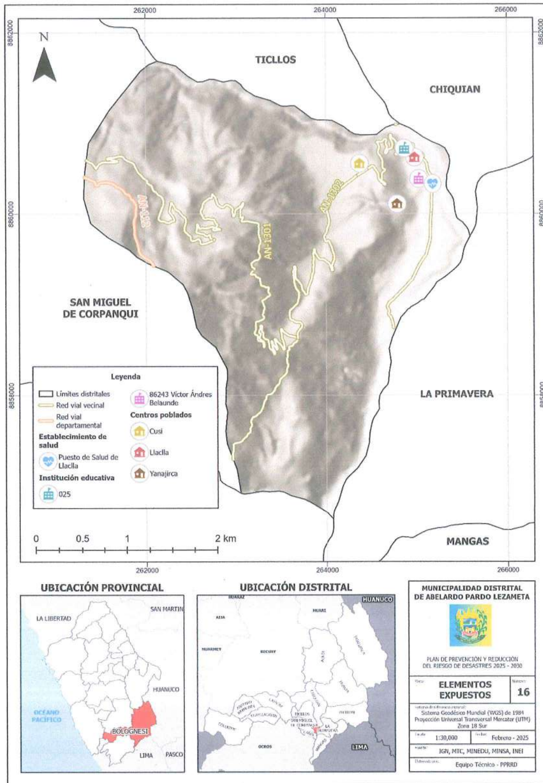
Mapa 16 Elementos expuestos ante los peligros de movimientos en masa e inundación fluvial
