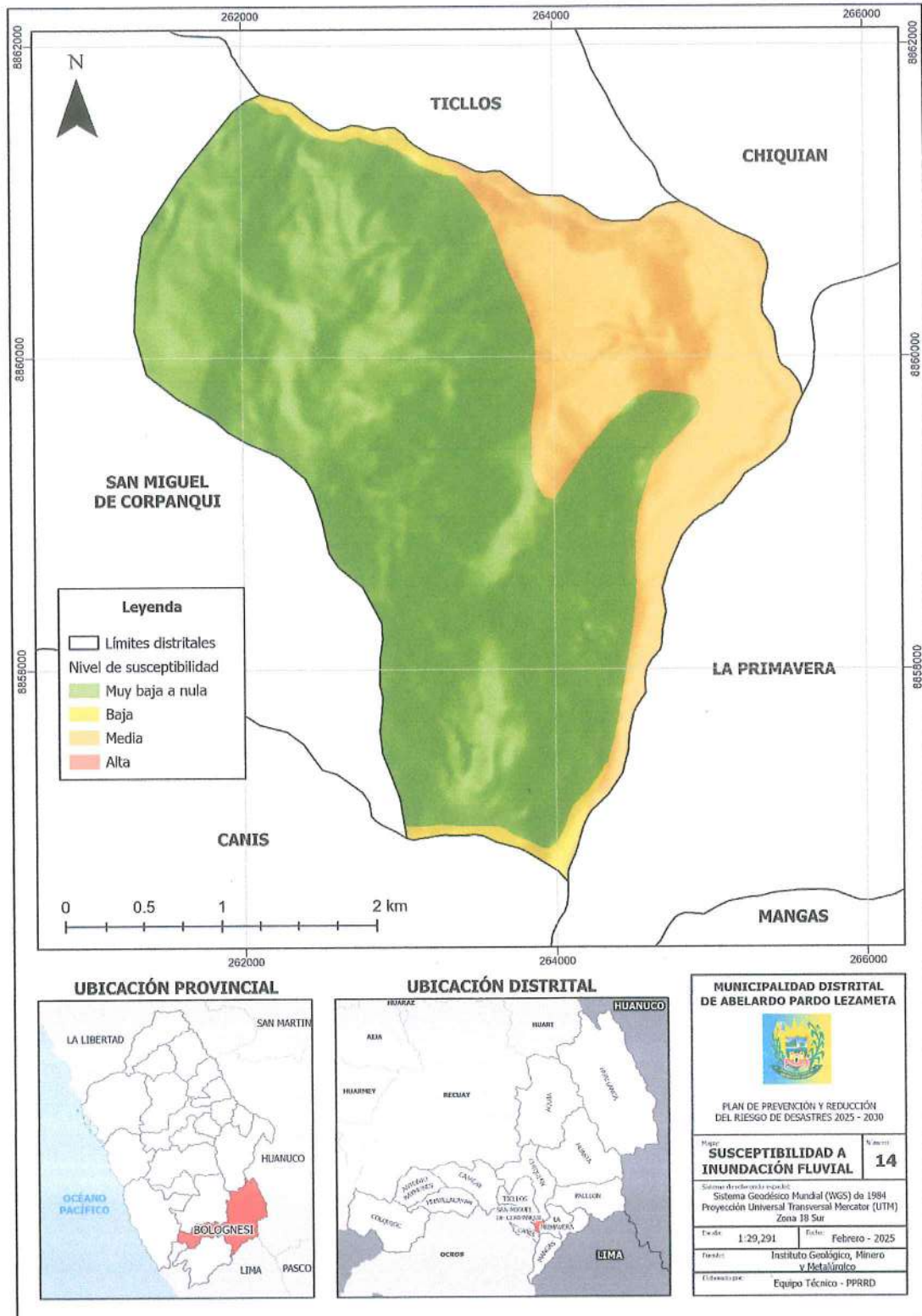
Mapa 14 Susceptibilidad ante inundación fluvial
