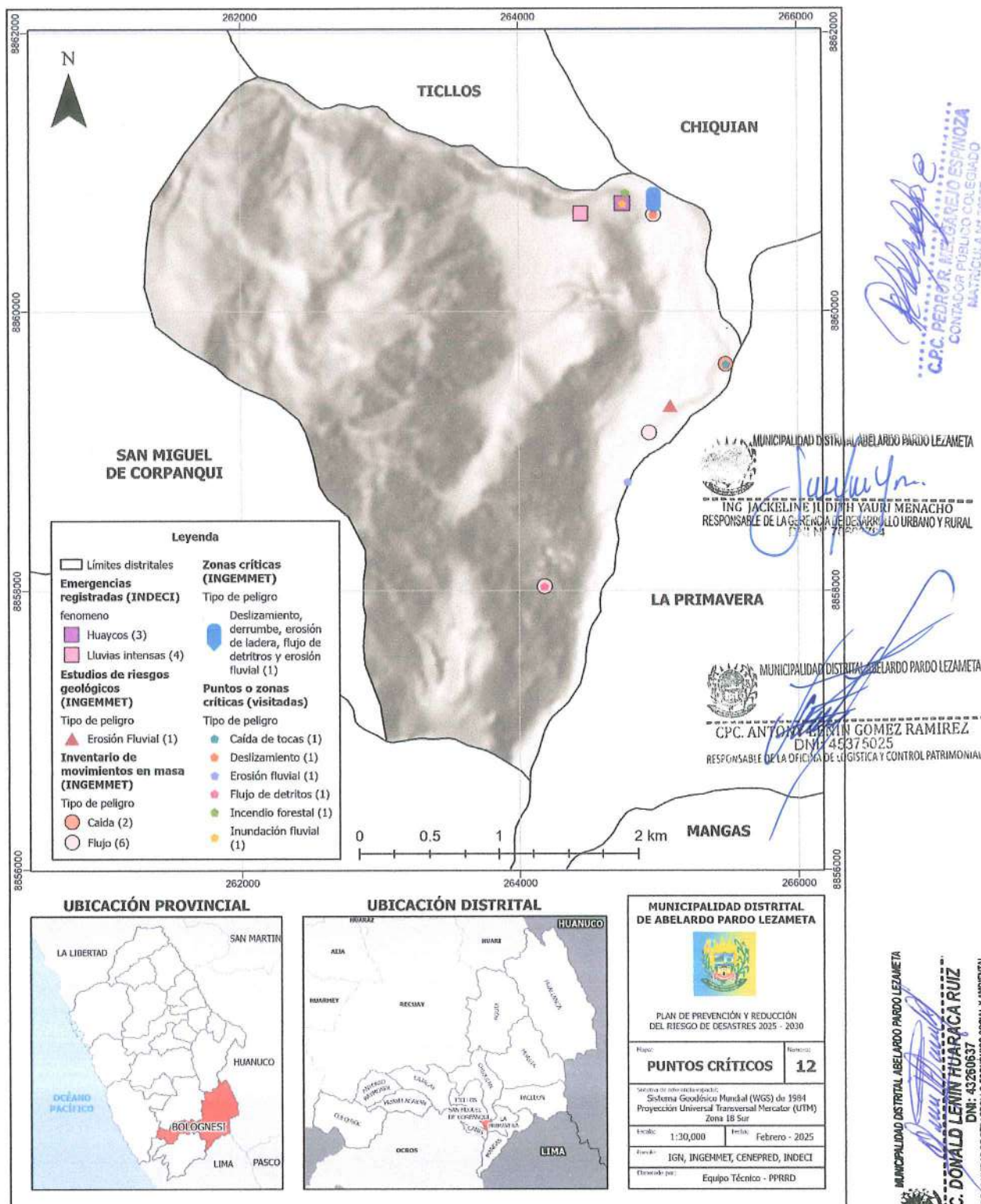
Mapa 12 Puntos y/o zonas críticas
