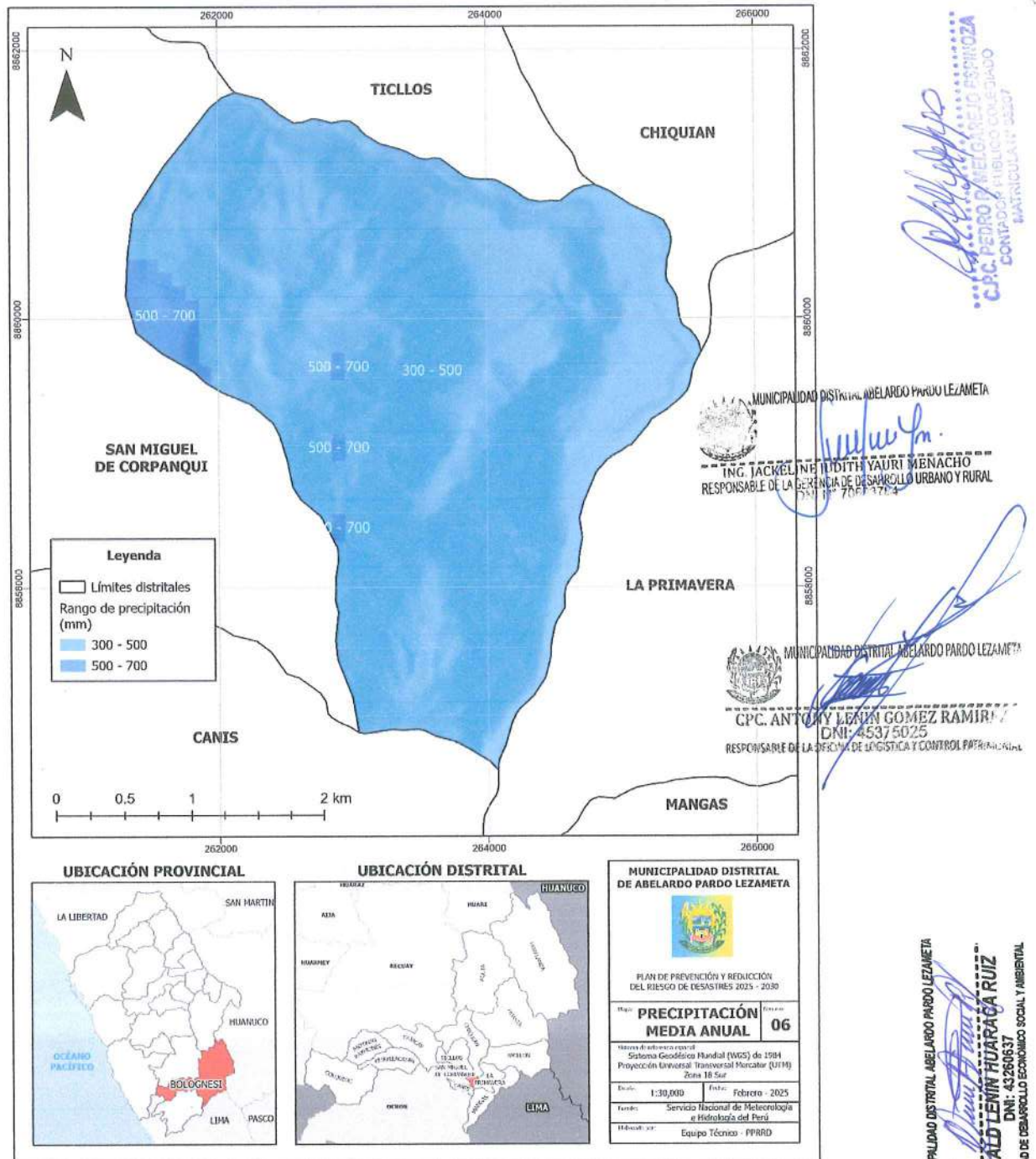
Mapa 6 Precipitación media anual
