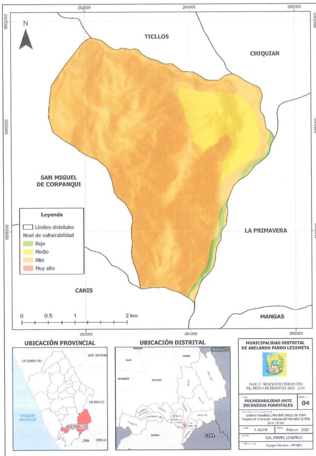
Mapa 17 Vulnerabilidad ante incendios forestales
