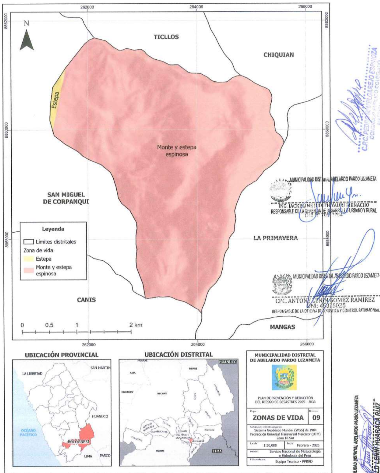
Mapa 9 Zonas de vida
