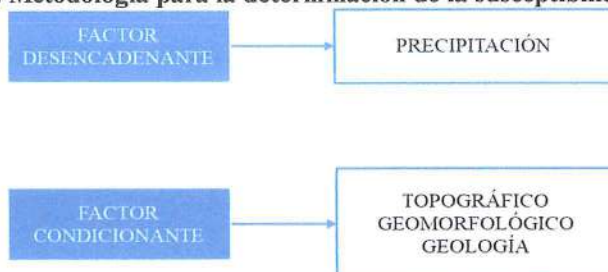
Gráfico 12 Metodología para la determinación de la susceptibilidad
