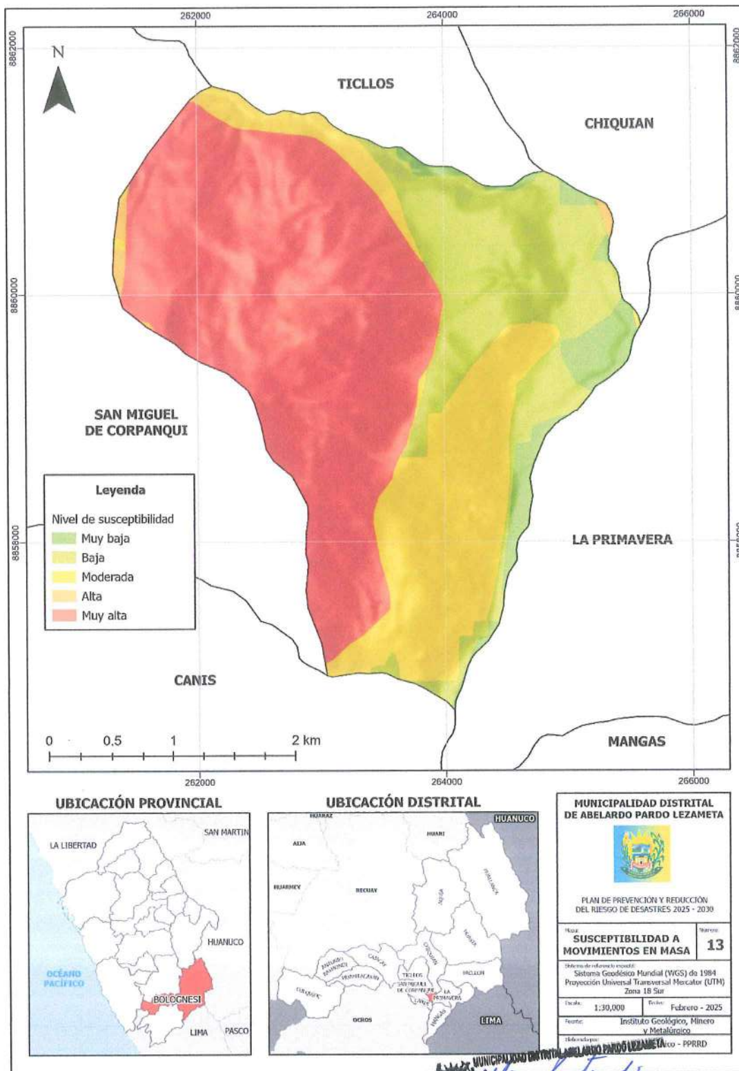
Mapa 13 Susceptibilidad a movimiento en masa
