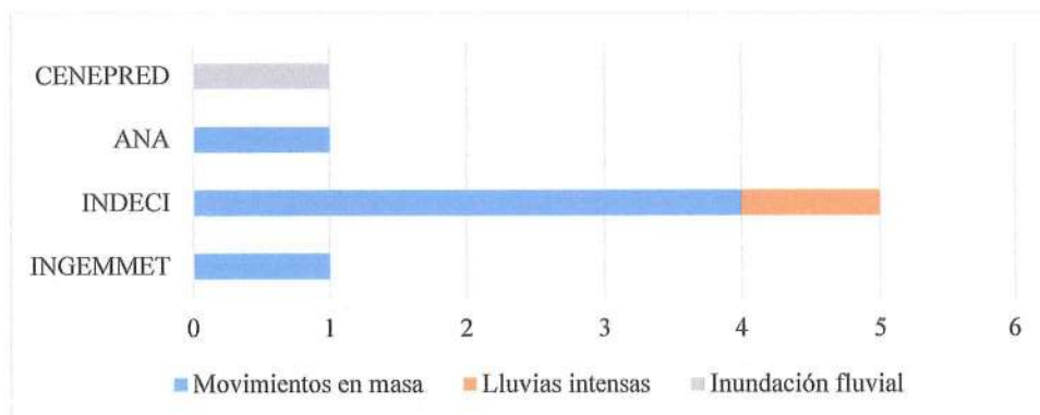
Gráfico 11 Resumen de peligros identificados
