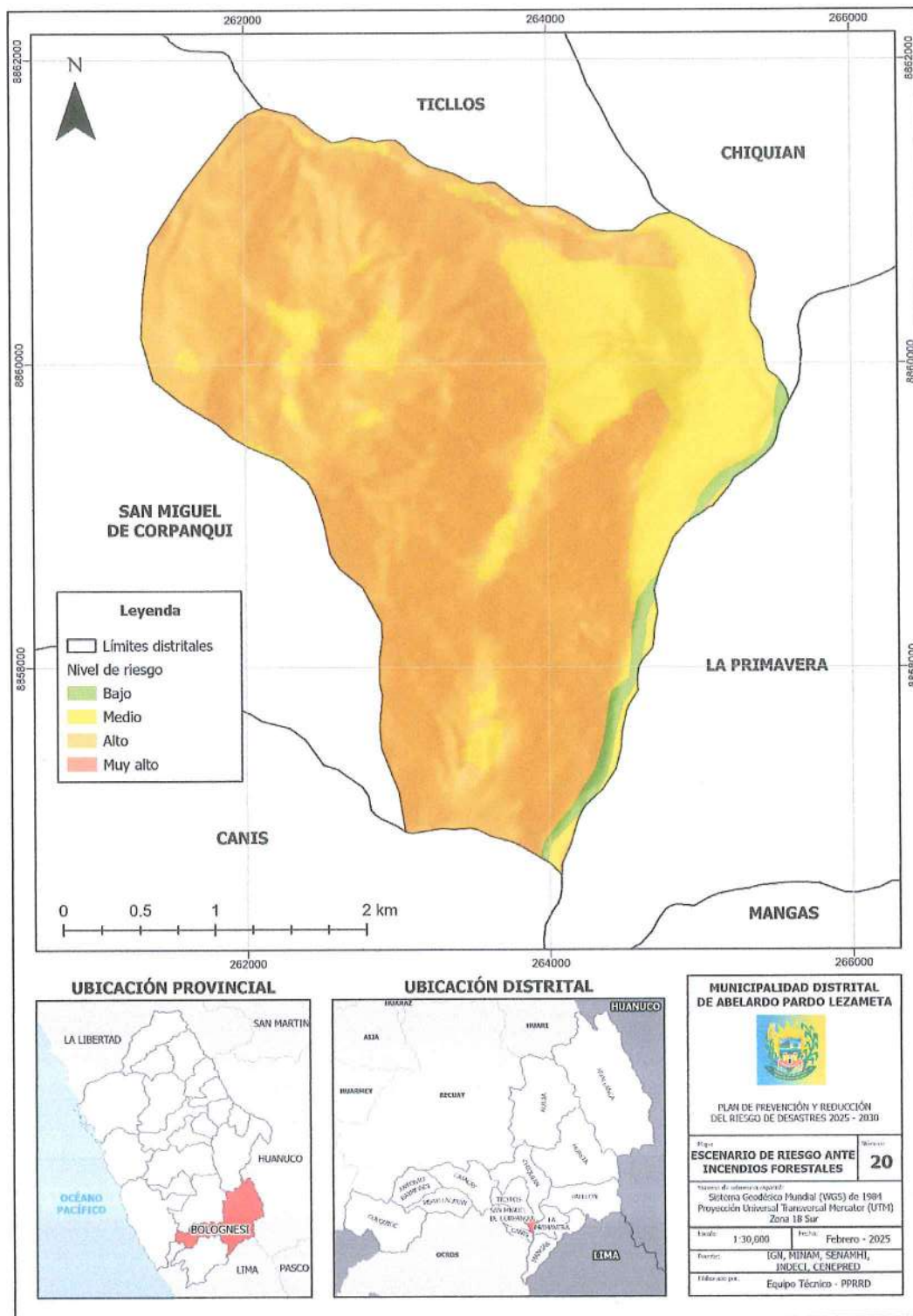
Mapa 20 Escenario de riesgo ante incendio forestal
