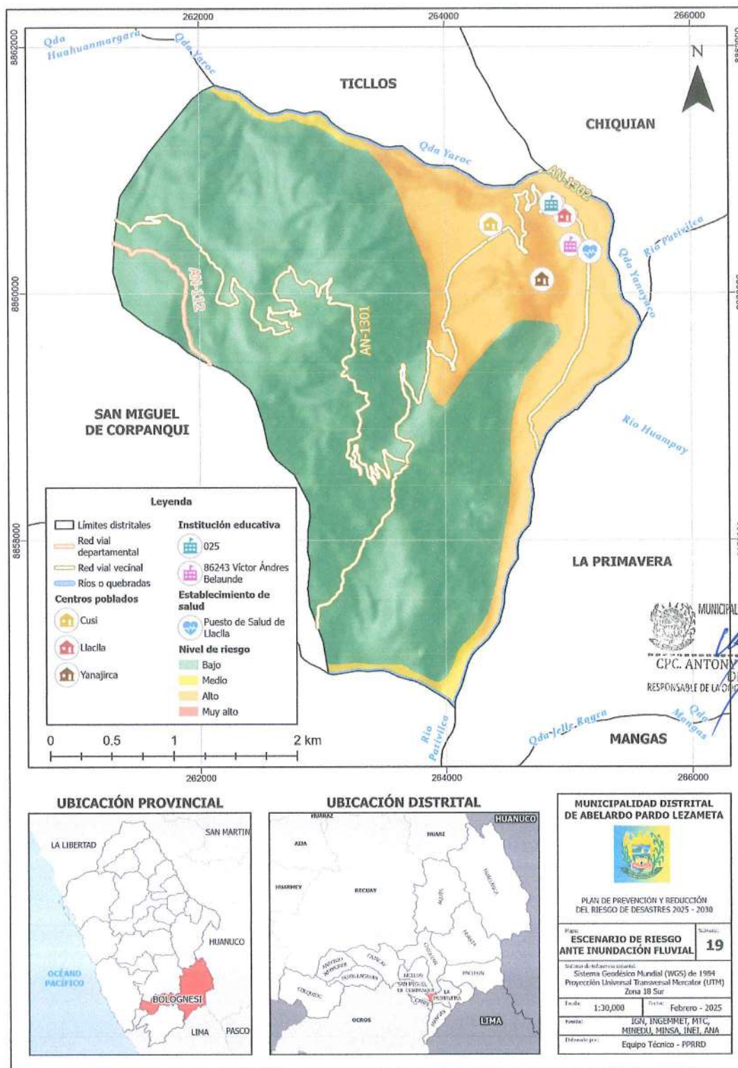
Mapa 19 Escenario de riesgo ante inundación fluvial
