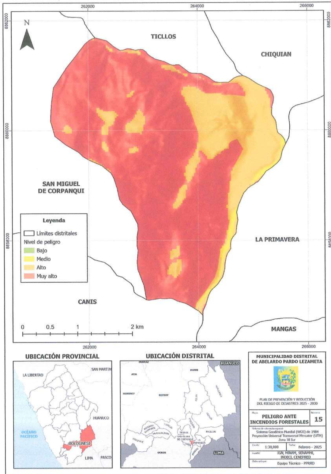
Mapa 15 Peligro ante incendio forestal
