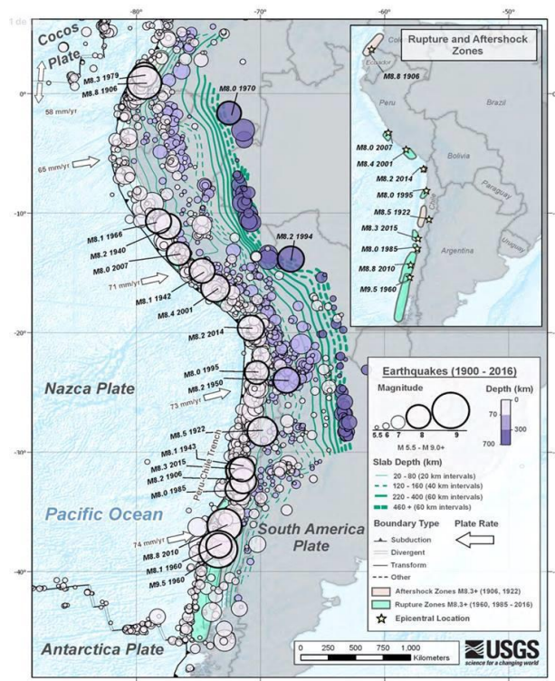
MAPA N° 014: PRINCIPALES SISMIOS OCURRIDOS ENTRE 1900 Y 2016 EN LA ZONA DE SUBDUCCION DE LA PLACA DE NAZCA
