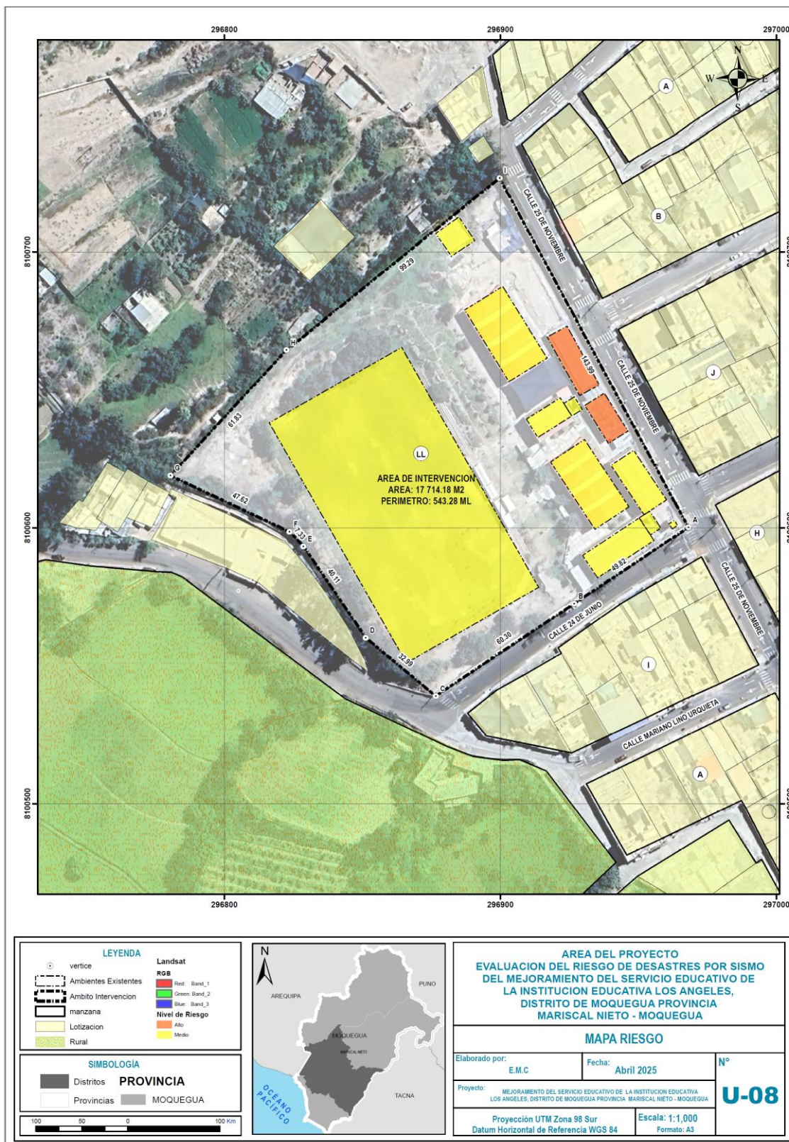
MAPA N° 019. MAPA DE RIESGOS
