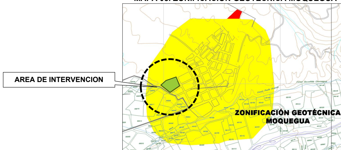
MAPA 08. ZONIFICACION GEOTECNICA MOQUEGUA
