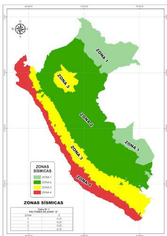
MAPA N° 013: ZONIFICACION SISMICA DEL PERU
