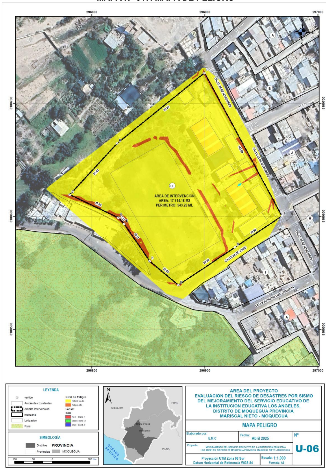
MAPA N° 017. MAPA DE PELIGRO
