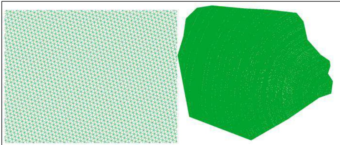
Figura 14 : Malla computacional del modelo hidráulico
